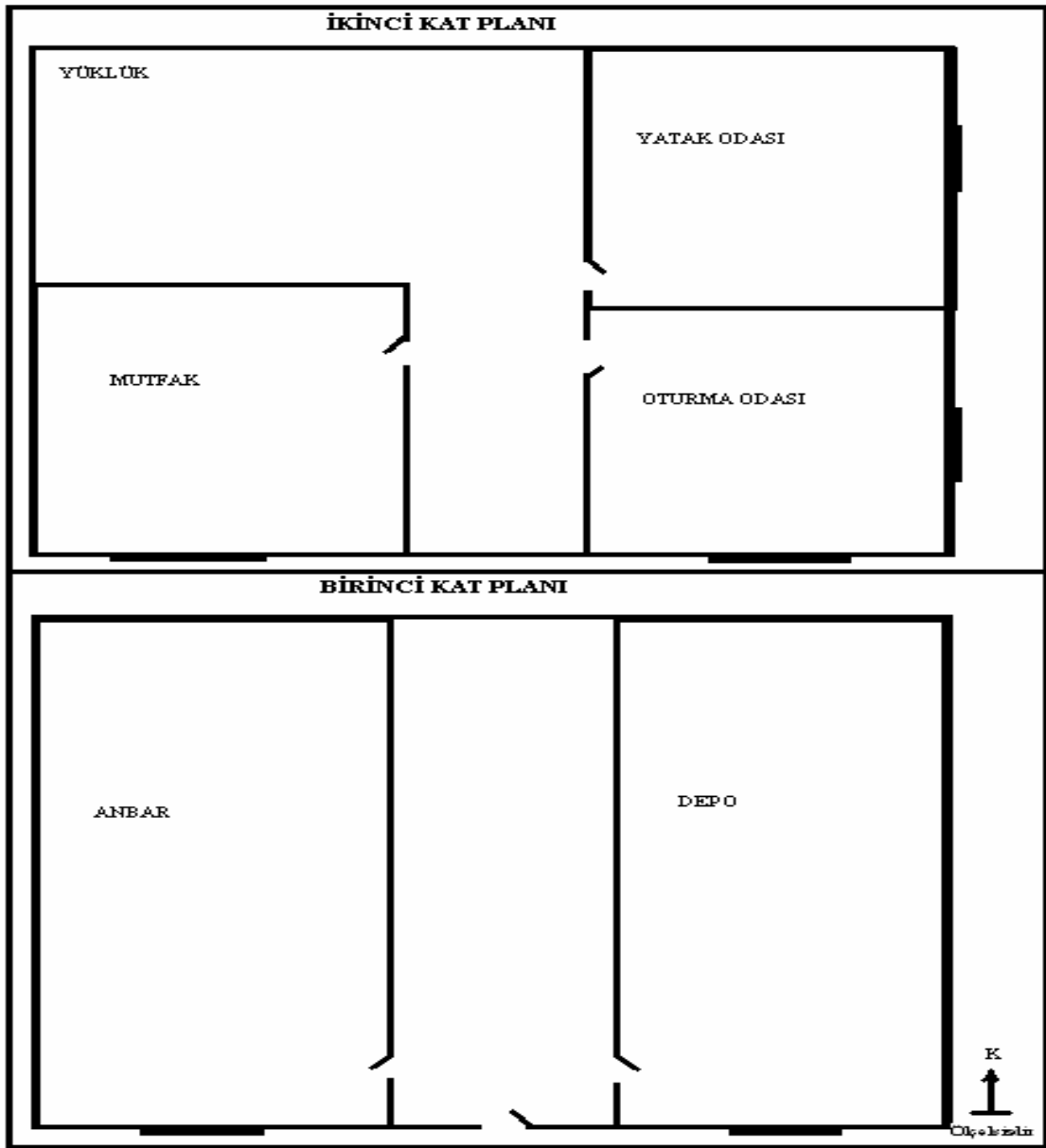
Şekil:33 Yusufkuyusu Köyü'nden İki Katlı Bir Ev Planı
