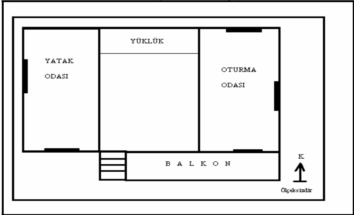
Şekil:34 Kırsal Kesimde Bir Ev Planı (Şerefli davutlu Köyü)
