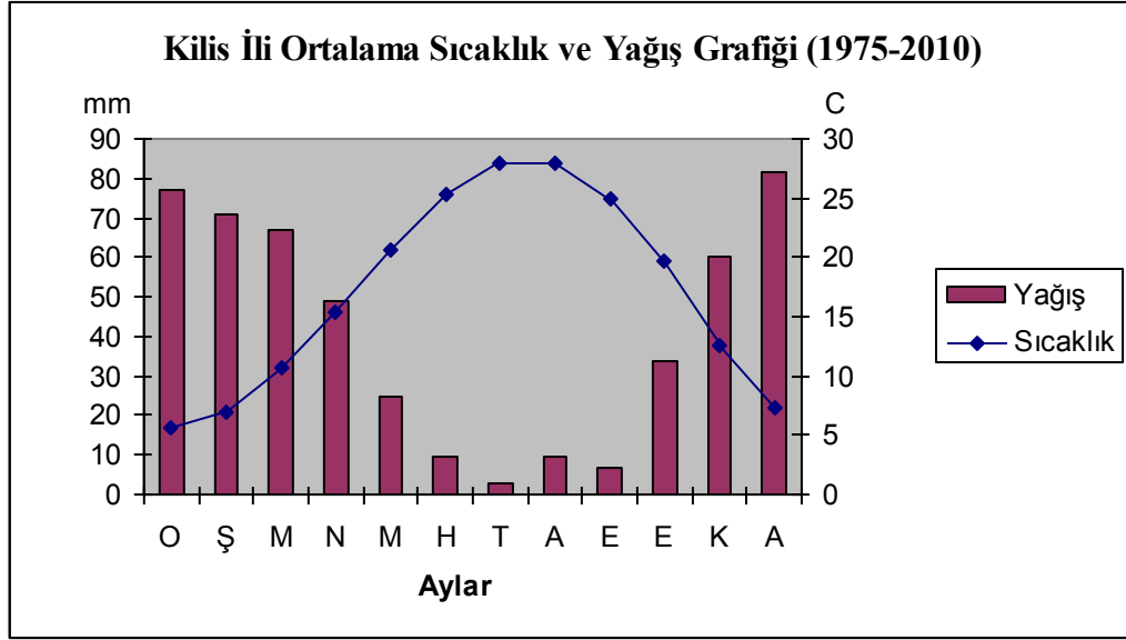
Grafik 1. Kilis Yağış ve Sıcaklık Ortalamaları (1975-2010)
