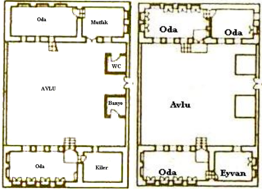
Şekil 5. Zemin ve 1. Kat Ev Planları
