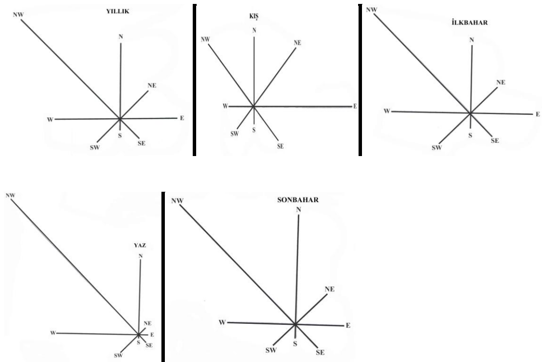
Şekil 2. Kilis Mevsimlere Göre Rüzgar Gülü Diyagramları (DMİ)
