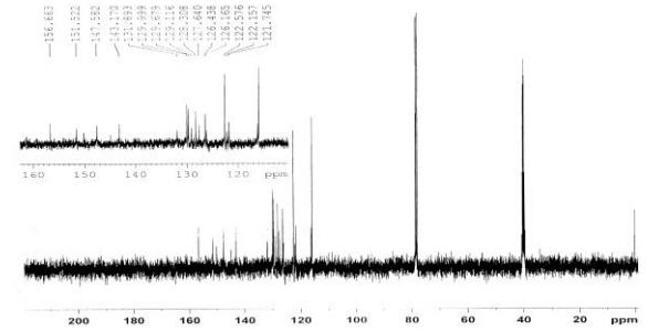
Şekil 4. 9 Bileşiğinin ^{13}\text{C} -NMR spektrumu
