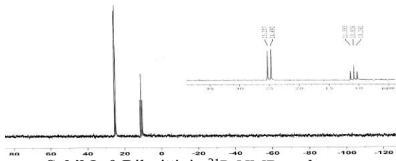
Şekil 2. 9 Bileşiğinin ^{31}\text{P} -NMR spektrumu
