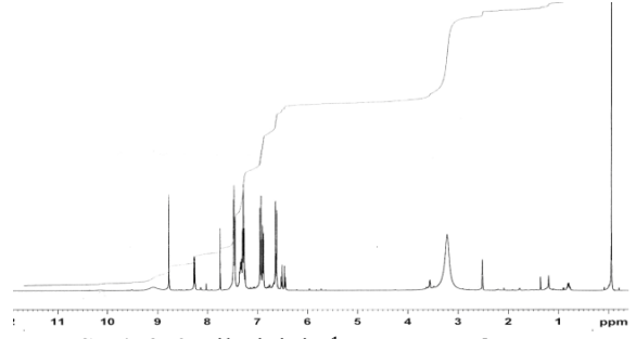
Şekil 3. 9 Bileşiğinin ^1\text{H} -NMR spektrumu
