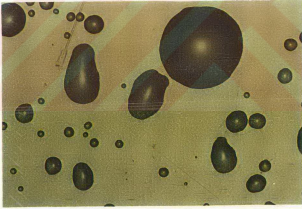
Resim 5.29. İslî Cam Üzerine Püskürtülen %75 Pamuk Yağı + %25 Motorin Karışımı Damlacıklarının Görüntüsü. (Püskürtme Açıklığı 100 cm. )
