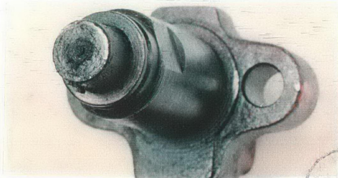
Resim 5.60. %25 Pamuk Yağı + %75 Motorin ile 100 Saatlik Çalışma Sonunda Enjektörün Görünüşü.
