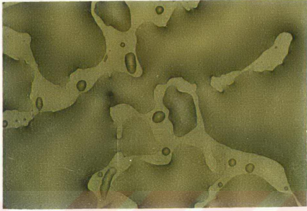
Resim 5.28. İslî Cam Üzerine Püskürtülen %75 Pamuk Yağı + %25 Motorin Karışımı Damlacıklarının Görüntüsü. (Püskürtme Açıklığı 50 cm. )
