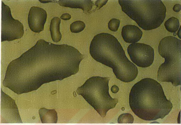
Resim 5.26. İslı Cam Üzerine Püskürtülen %50 Pamuk Yağı + %50 Motorin Karışımı Damlacıklarının Görüntüsü. ( Püskürtme Açıklığı 100 cm. )
