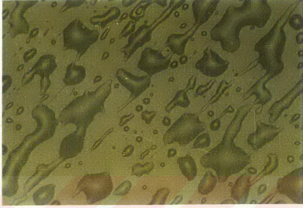
Resim 5.20. İsli Cam Üzerine Püskürtülen %25 Pamuk Yağı + %75 Motorin Karışımı Damlacıklarının Görüntüsü. ( Püskürtme Açıklığı 20 cm. )
