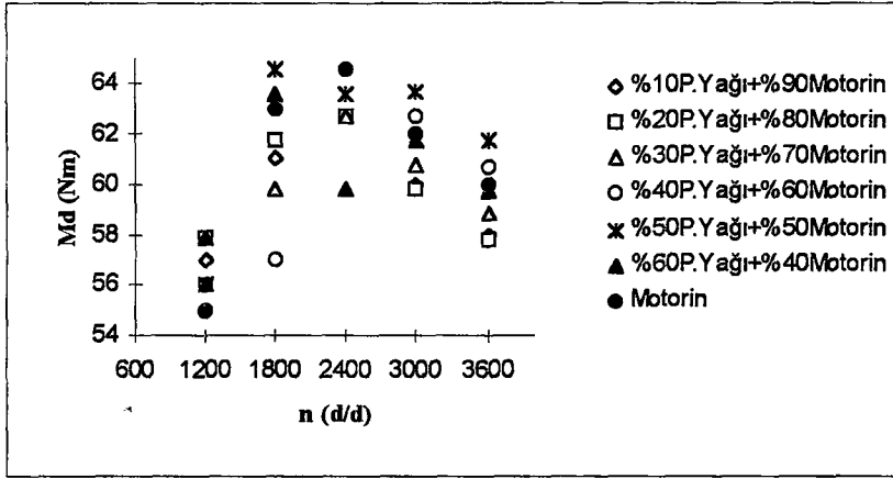
Şekil 5.32. Motorin ile Çeşitli Oranlardaki Pamuk Yağı + Motorin Karışımları Kullanılması Halinde Tam Gazda Çalışmada Md Değişimi.
