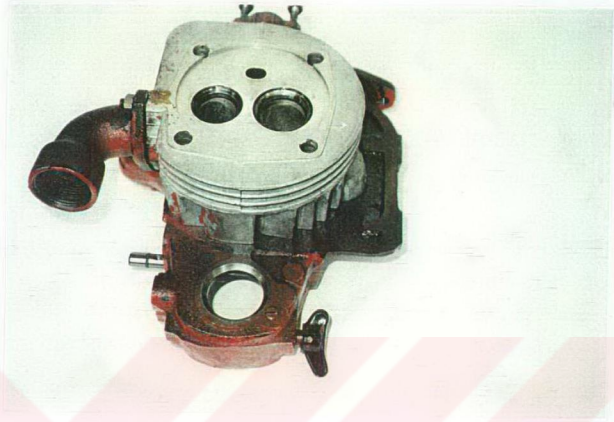
Resim 5.33. Silindir Kafası ve Yanma Odasının Deneyler Yapılmadan Önceki Görünüşü.
