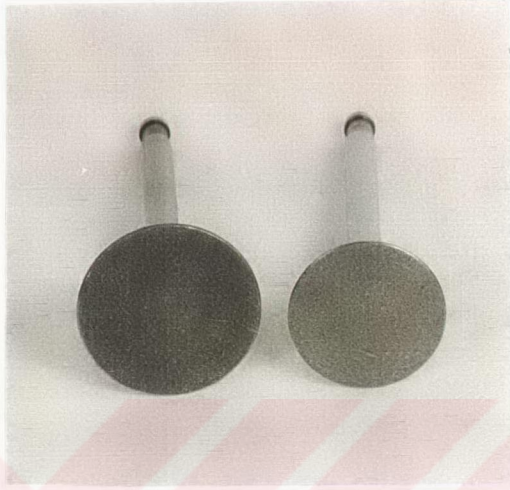
Resim 5.35. Emme ve Egzoz Supabının Deneyler Yapılmadan Önceki Görünüşü.
