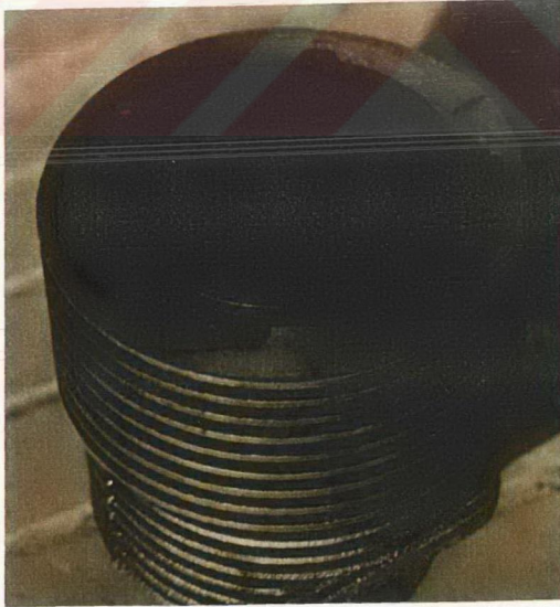
Resim 5.78. %75 Pamuk Yağı + %25 Motorin ile 100 Saatlik Çalışma Sonunda Gömleğin Görünüşü.
