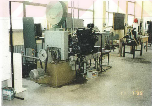
Resim 4.3. Deney Motoru ve Dinamometre.
