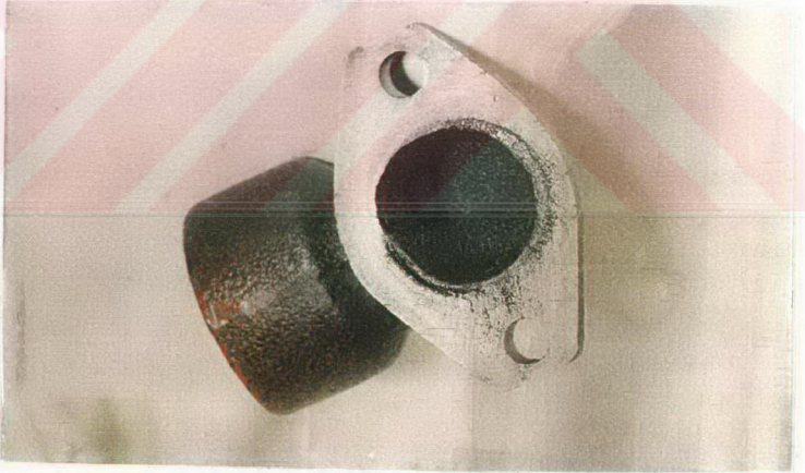
Resim 5.56. %25 Pamuk Yağı + %75 Motorin ile 100 Saatlik Çalışma Sonunda Egzoz Manifoldunun Görünüşü.
