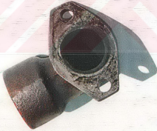
Resim 5.50. Motorin ile 100 Saatlik Çalışma Sonunda Egzoz Manifoldunun Görünüşü.
