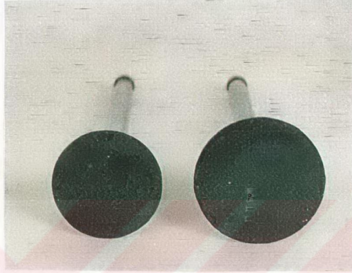
Resim 5.75. %75 Pamuk Yağı + %25 Motorin ile 100 Saatlik Çalışma Sonunda Emme ve Egzoz Supabının Görünüşü.
