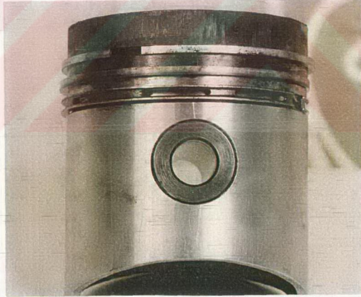
Resim 5.72. %75 Pamuk Yağı + %25 Motorin ile 100 Saatlik Çalışma Sonunda Pistonun Görünüşü.
