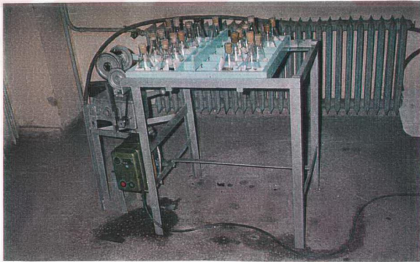
Resim 5.2. Sıvanma Deneyinde Kullanılan Hareketli Sehpa.
