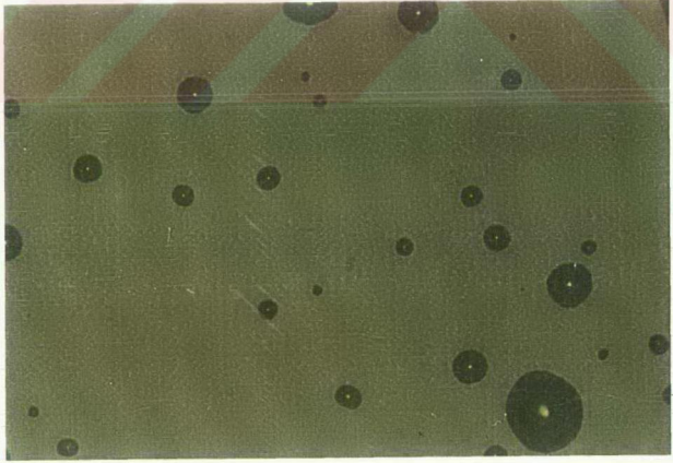
Resim 5.17. İsli Cam Üzerine Püskürtülen Motorin Damlacıklarının Görüntüsü. ( Püskürtme Açıklığı 50 cm. )
