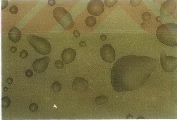
Resim 5.21. İsli Cam Üzerine Püskürtülen %25 Pamuk Yağı + %75 Motorin Karışımı Damlacıklarının Görüntüsü. ( Püskürtme Açıklığı 50 cm. )
