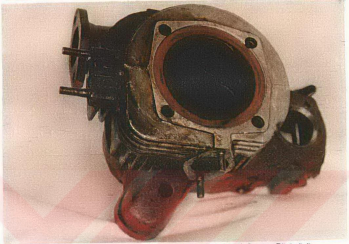
Resim 5.41. Motorin ile 100 Saatlik Çalışma Sonunda Silindir Kafasının Görünüşü.
