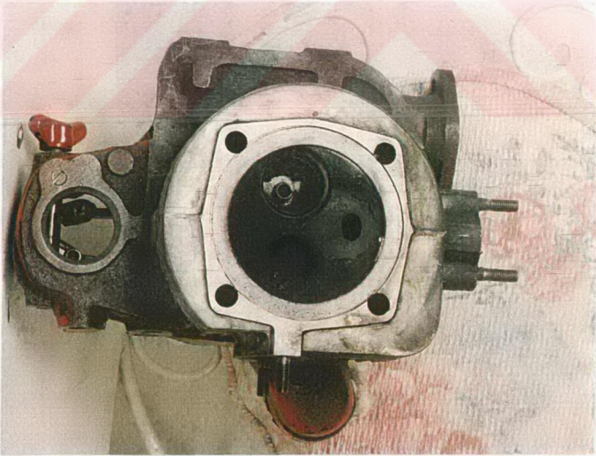
Resim 5.70. %75 Pamuk Yağı + %25 Motorin ile 100 Saatlik alıřma Sonunda Yanma Odası ve Supap Yuvalarının Grnř.
