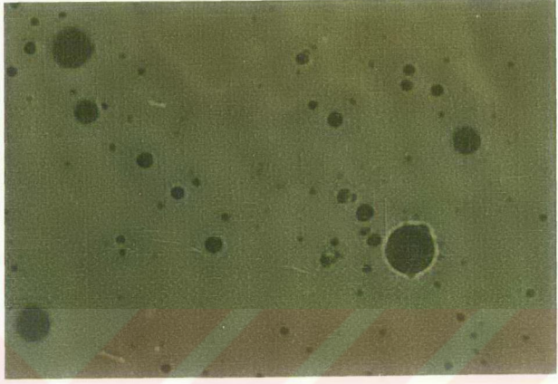
Resim 5.16. İsli Cam Üzerine Püskürtülen Motorin Damlacıklarının Görüntüsü. (Püskürtme Açıklığı 20 cm.)
