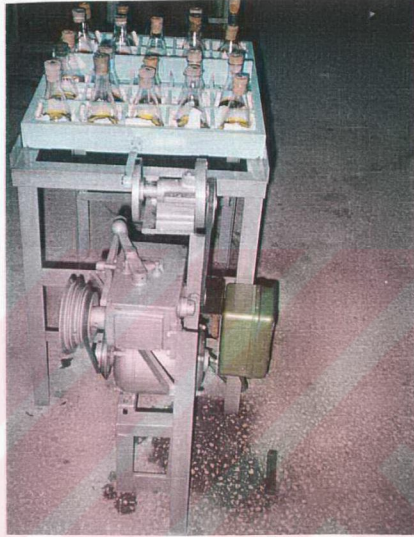
Resim 5.1. Sıvanma Deneyinde Kullanılan Hareketli Sehpa.
