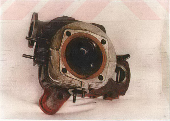
Resim 5.40. Motorin ile 100 Saatlik Çalışma Sonunda Silindir Kafasının Görünüşü.
