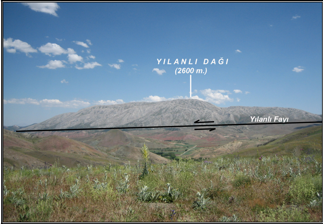
Foto 8: Kangal Havzası'nın (Sivas) kuzeyinde KD-GB doğrultusunda uzanan ve Mesozoyik yaşlı kireçtaşlarından oluşan Yılanlı Dağı.
