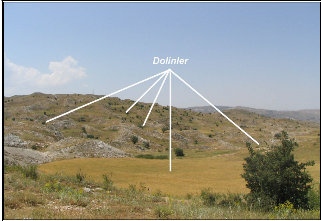
Foto 58: Karabel Çayı Havzası'nın doğusundaki Karakale güneyinde jipsler üzerinde oluşan erime dolinleri
