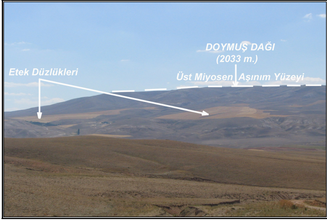
Foto 17: Kangal Havzası'nın batısında Mesozoyik yaşlı kireçtaşlarından oluşan Doymuş Dağı ve kuzey yamaçlarında görülen etek düzlükleri
