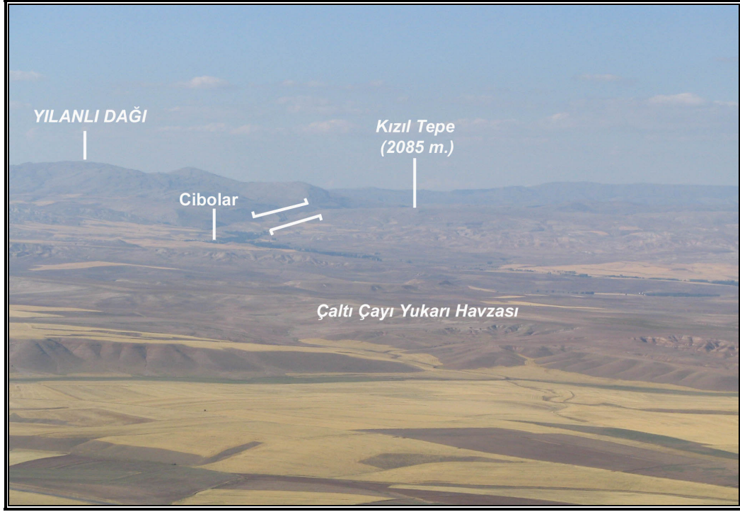
Foto 36: Yılanlı Dağı güneyinde Boğaz Dere üzerinde görülen Cibolar Boğazı
