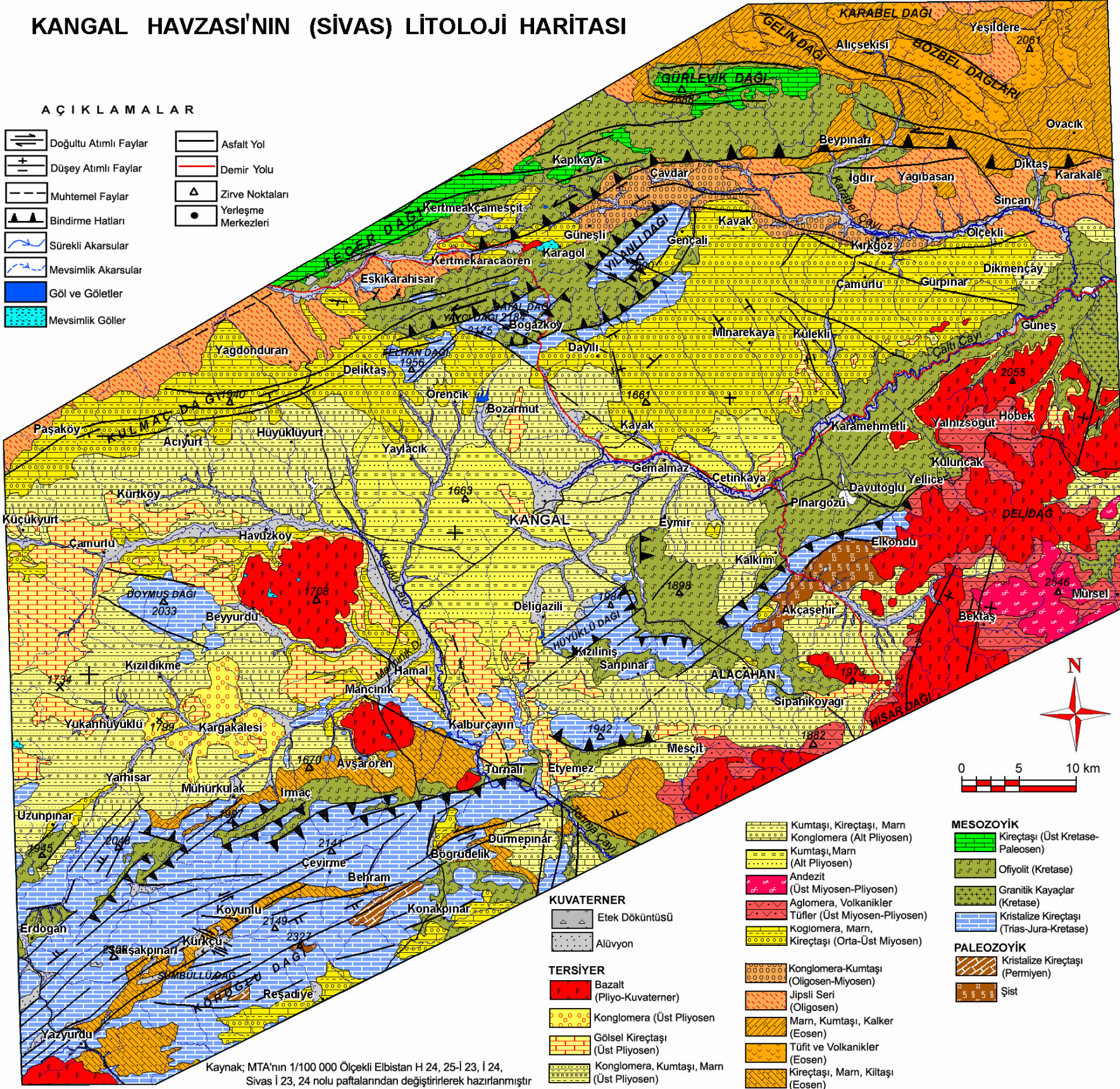
Şekil 7: Kangal Havzası'nın (Sivas) litoloji haritası
