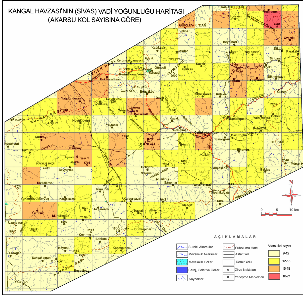
Şekil 29: Kangal Havzası'nın (Sivas) vadi yoğunluğu haritası
