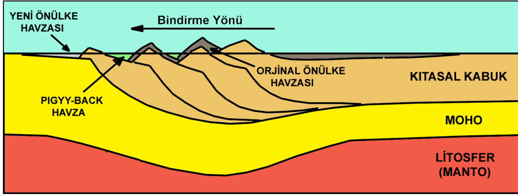
Şekil 18: Bindirme cephesinde oluşan Piggy-back havzası ( http://www.geolsoc.org.uk )
