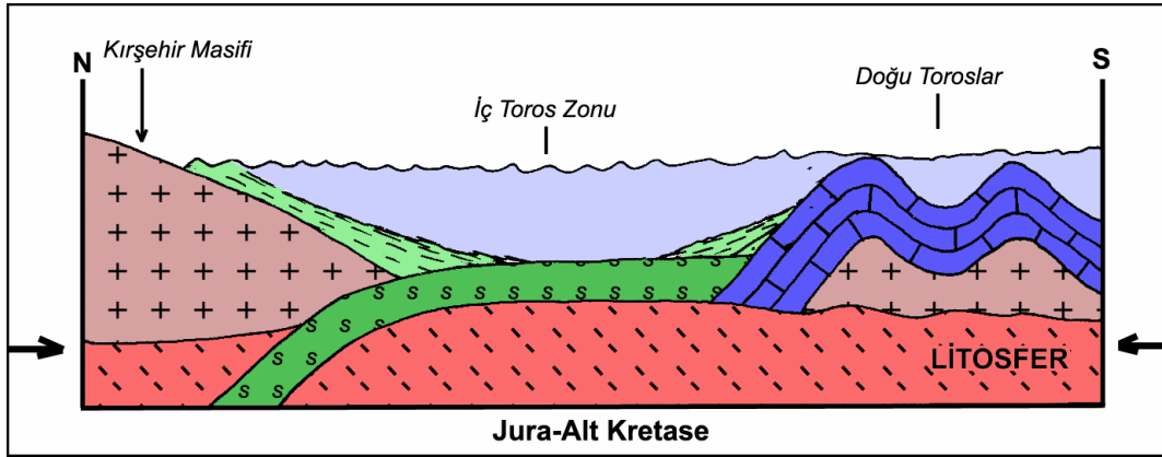
Şekil 43: Jura-Alt Kretase döneminde inceleme alanının genel tektonik yapısını gösterir şematik kesit
