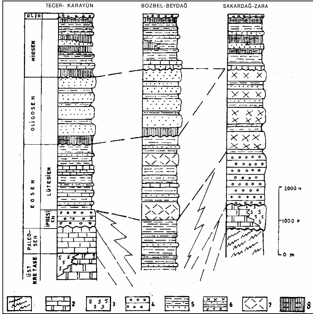
Şekil 11: İnceleme alanının kuzeyinde Tecer Dağları ve kuzeybatıda Bozbel Dağları çevresinde yüzeyleyen birimlerin stratigafik kesiti, 1- Kristalin, 2- Kalker, 3- Ofiyolit, 4- Konglomera, 5- Marn, siltaşı, 6- Andezit, kumtaşı, marn, 7- Tüfit, 8- Jips (Kurtman, 1973)
