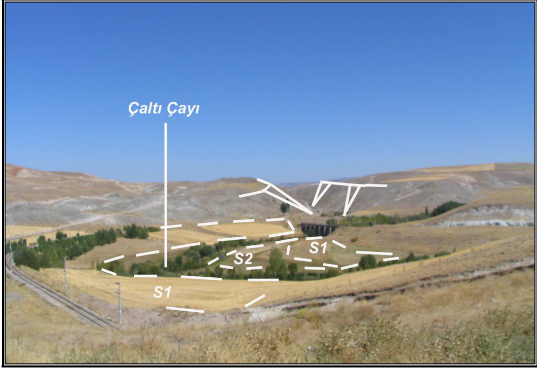
Foto 32: Çetinkaya doğusunda Çaltı Çayı Vadisi'ne karşılık gelen Karaboğaz, menderes yeniği sekileri ve Sivas-Divriği demir yolu
