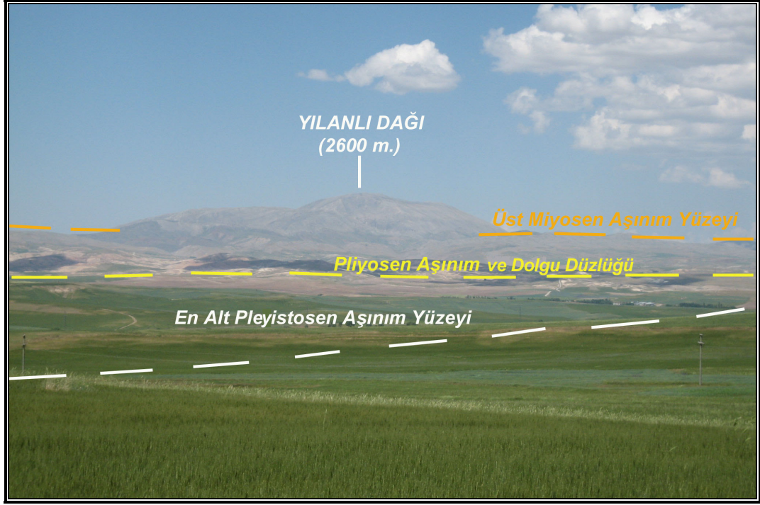
Foto 18: Yılanlı Dağı'nın güneyinde görülen Üst Miyosen aşınım yüzeyleri
