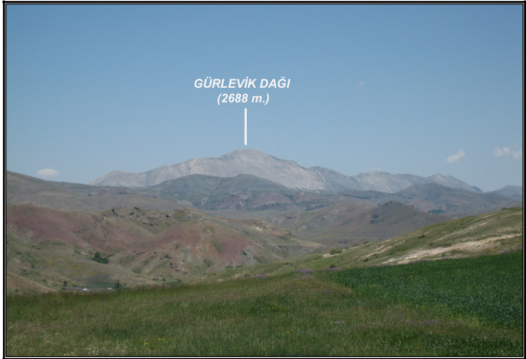
Foto 10: Tecer Dağları'nın doğuya devamında Gürlevik Kireçtaşları'ndan oluşan Gürlevik Dağı
