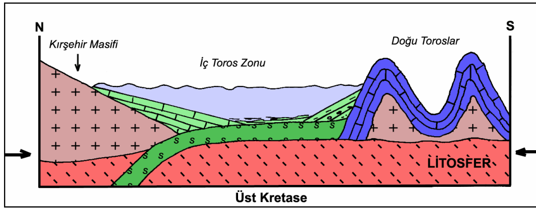
Şekil 44: Üst Kretase döneminde inceleme alanının genel tektonik yapısını gösterir şematik kesit
