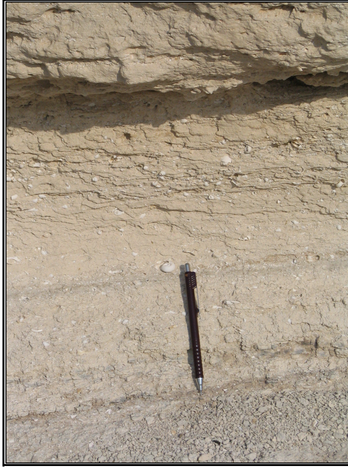
Foto 2: Hamal doğusunda Etyemez Üyesi'nin üst düzeylerinde gözlenen gastropod kavkaları
