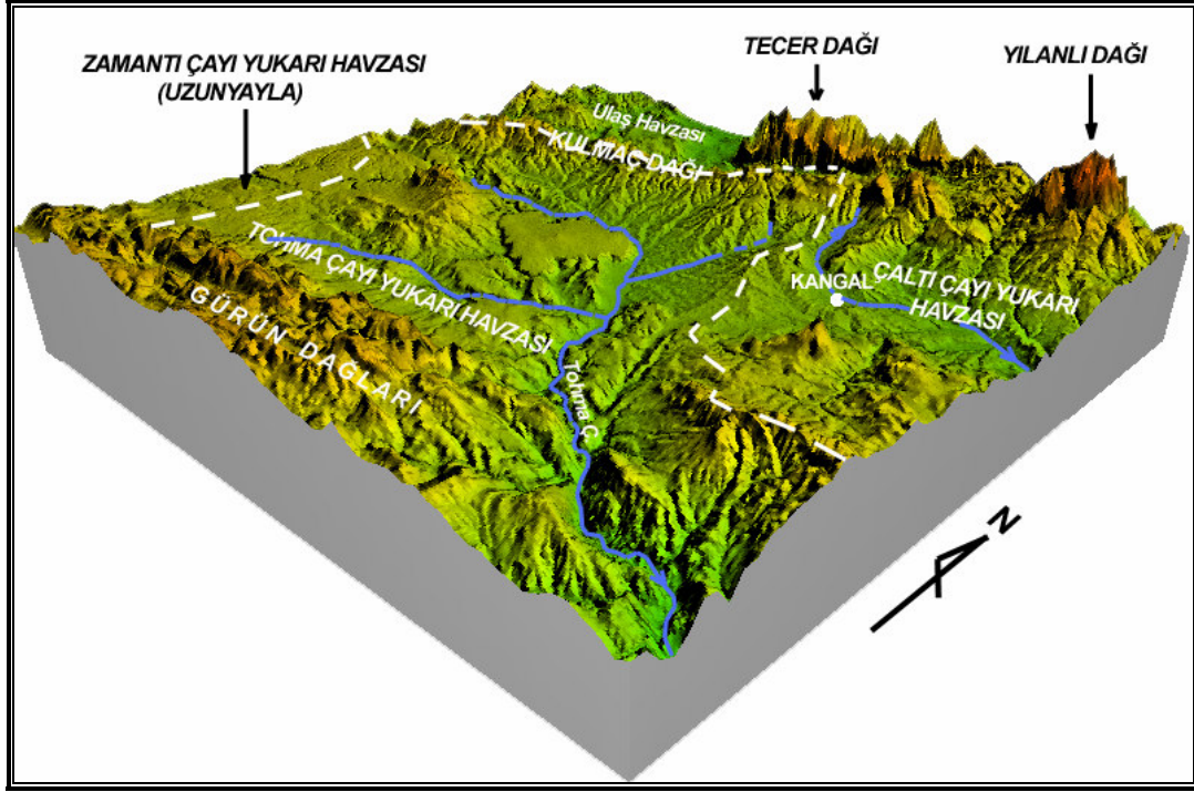
Şekil 32: Tohma Çayı Yukarı Havzası'nı (Kangal batısı) gösteren blokdiagramı (Sayısal yükselti modeline göre)
