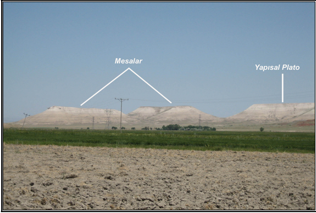
Foto 79: Tohma Çayı Vadisi'nde Ötegeçe Mahallesi doğusunda görülen mesalar
