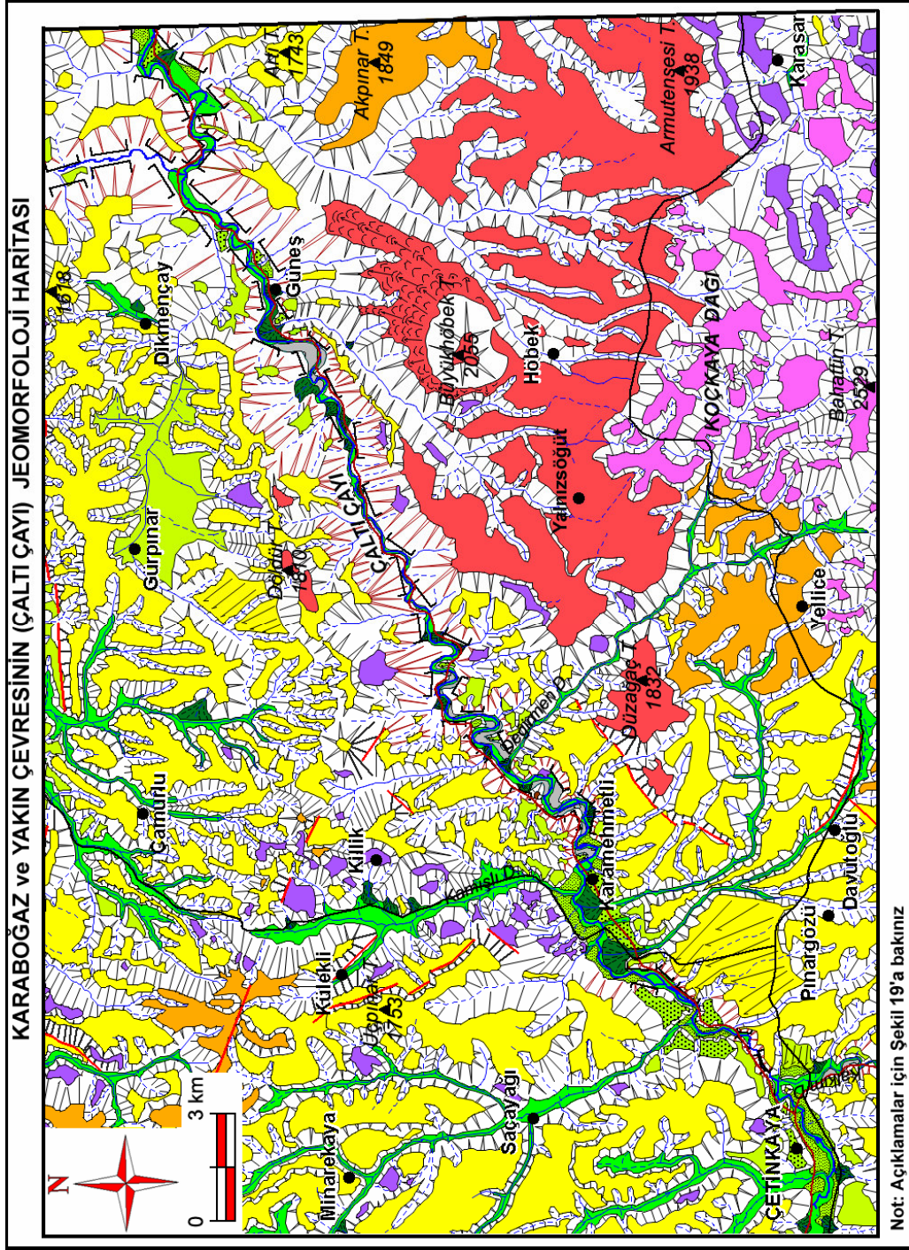
Şekil 39: Karaboğaz ve yakın çevresinin (Çaltı Çayı) jeomorfoloji haritası
