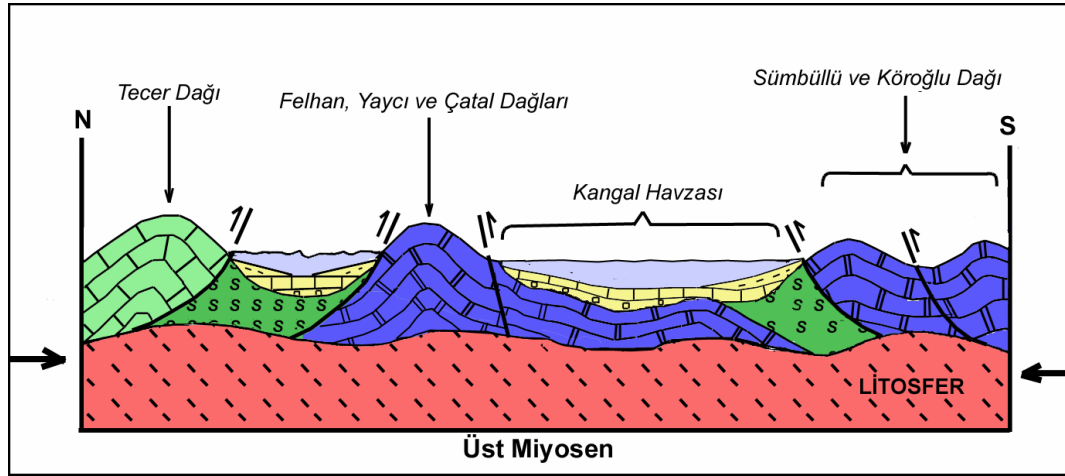
Şekil 47: Üst Miyosen'de inceleme alanının genel tektonik yapısını gösterir şematik kesit
