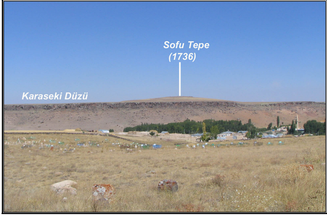
Foto 51: Mancınık güneyindeki Karaseki Düzü'nün batı yamaçlarında görülen kaya düşmeleri, minyatür bir volkan konisine karşılık gelen Sofu Tepe (1736 m) ve bazaltlara bağılı oluşan kornişler
