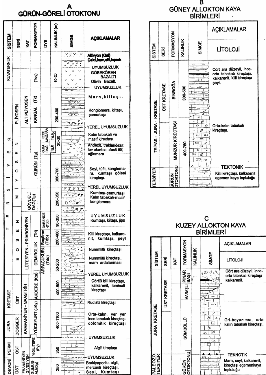
Şekil 8: Kangal Havzası'nın güneybatısında otokton ve allokton kaya birimlerine ait dikme kesitler (Atabey ve diğ., 1997)
