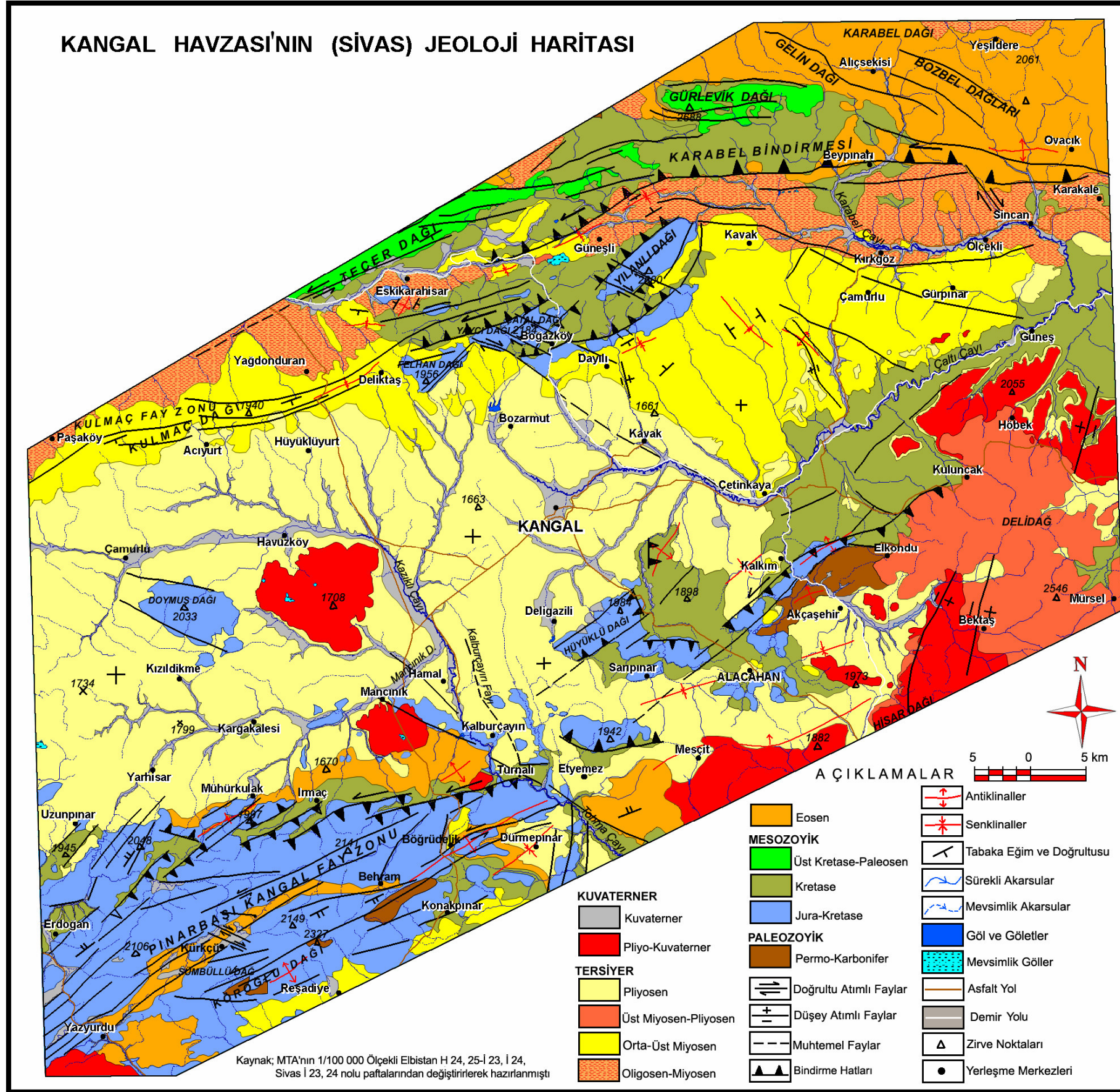
Şekil 6: Kangal Havzası'nın (Sivas) jeoloji haritası
