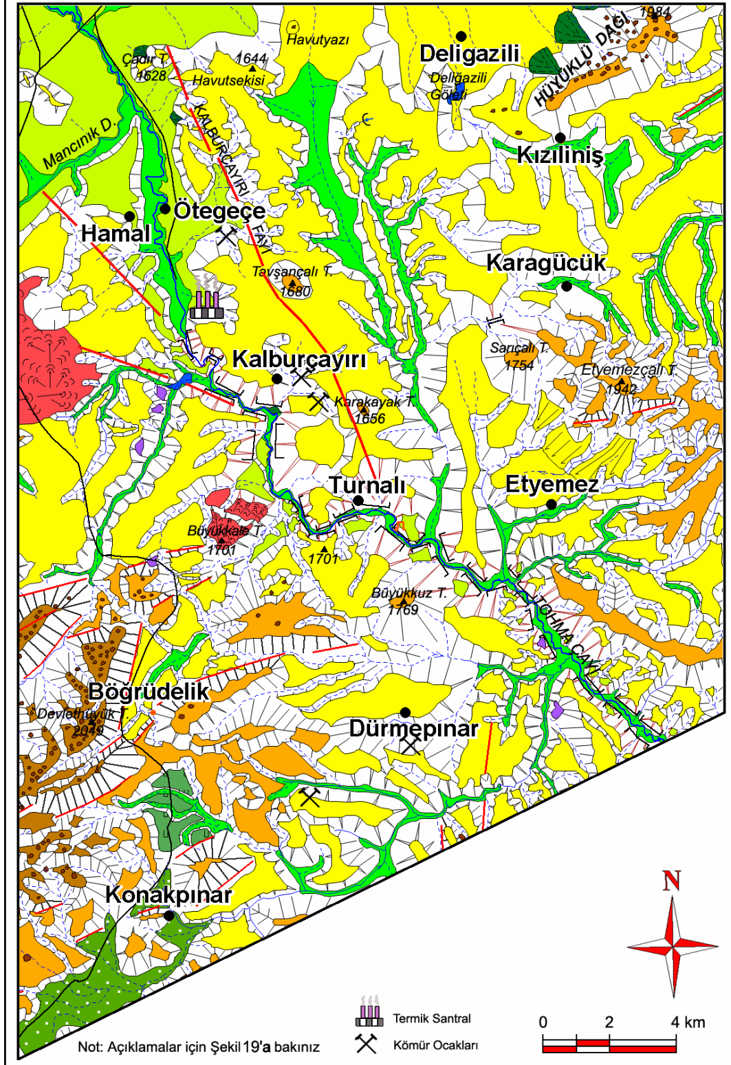
Şekil 38: Sarıyolak Boğazi ve Kalburçayırı Linyit Havzası'nın (Kangal) jeomorfoloji haritası
