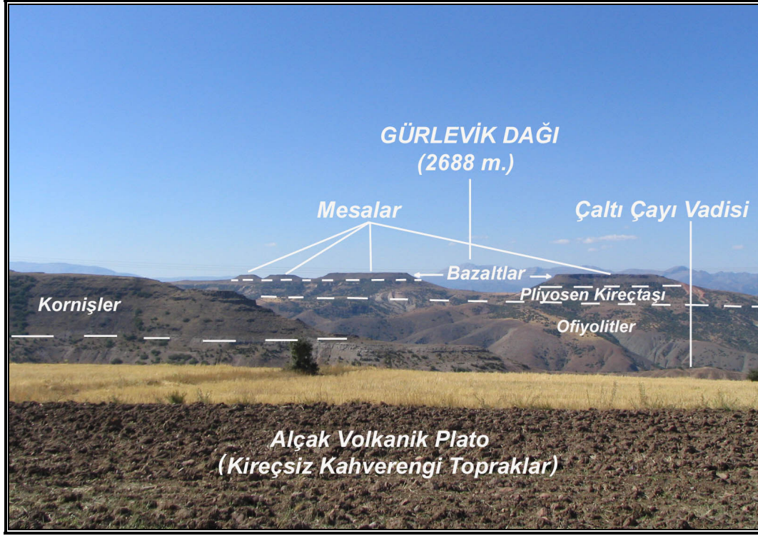
Foto 25: Yalnızsöğüt ve Höbek kuzeyinde Çaltı Çayı tarafından yarılmış olan bazaltlar ve kuzey yamaçtaki parçalarına karşılık gelen mesa yapılı şahit tepeler
