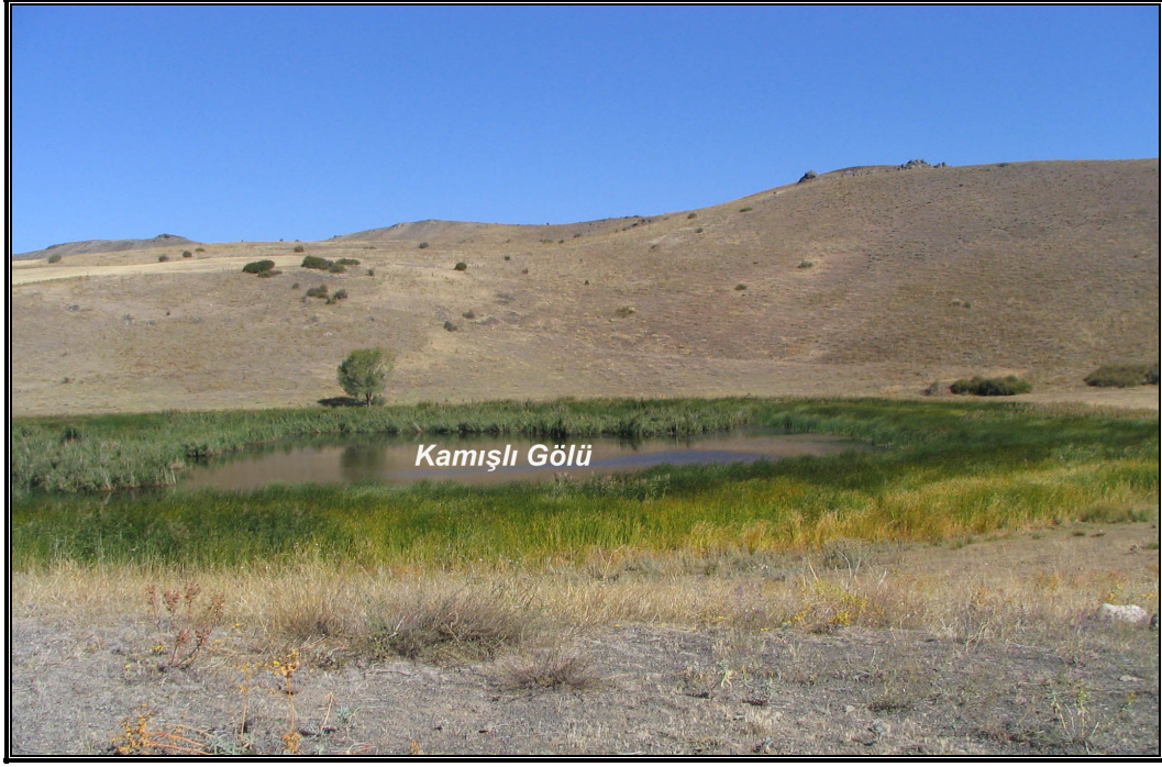
Foto 85: Aygır Gölü doğusunda, Pliyo-Kuvaterner volkanitleri üzerinde oluşan Kamışlı Gölü
