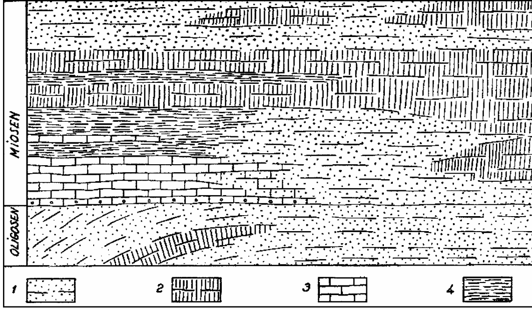
Şekil 13: Oligosen-Miyosen sedimantasyonuna ait şematik dikine kesit, 1- Alacalı Gre, 2- Jips, 3- Kalker (Bürdigaliyen), 4- Marn (Orta Miyosen) (Kurtman,1961)
