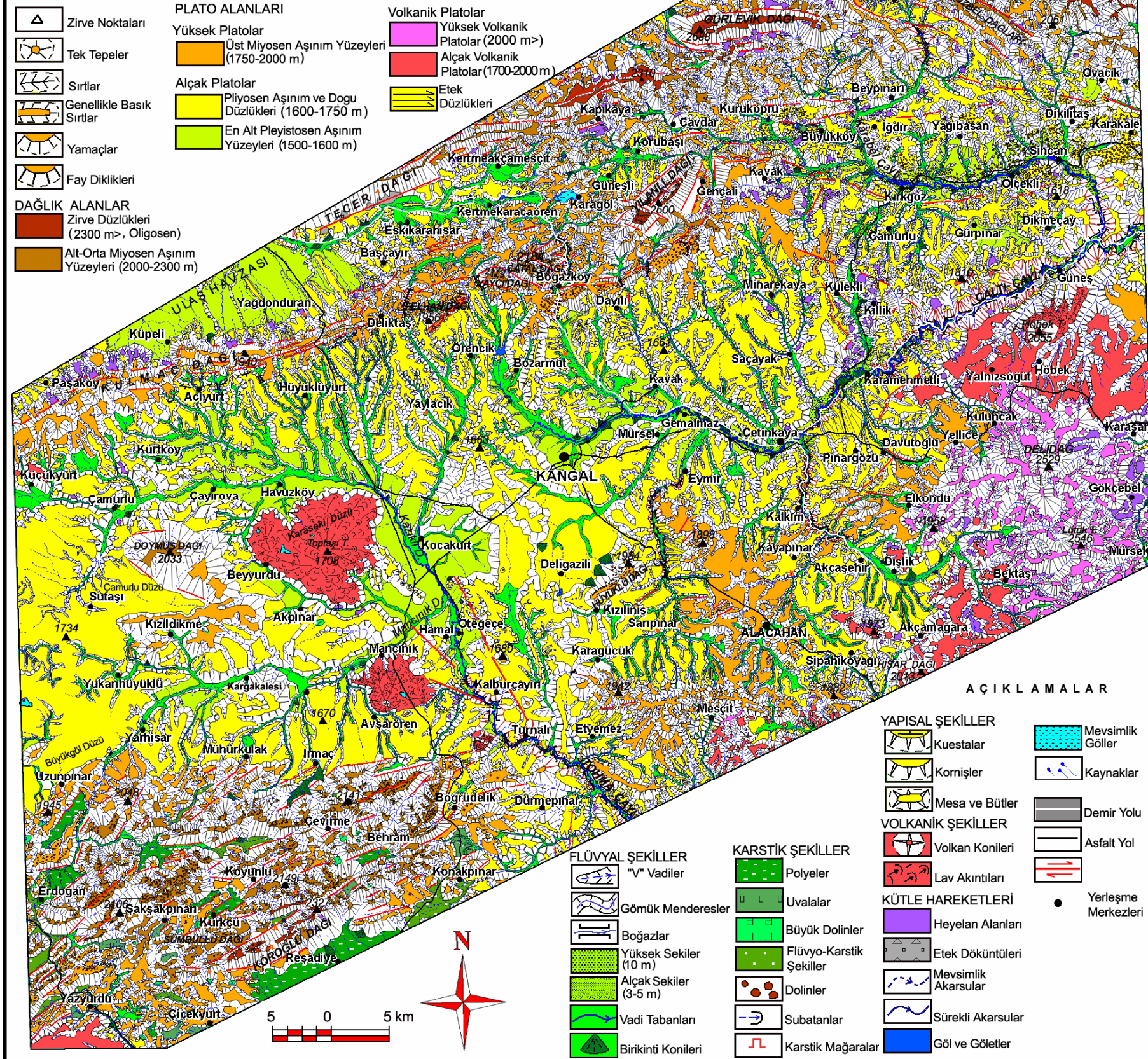
Şekil 19: Kangal Havzası'nın (Sivas) jeomorfoloji haritası
