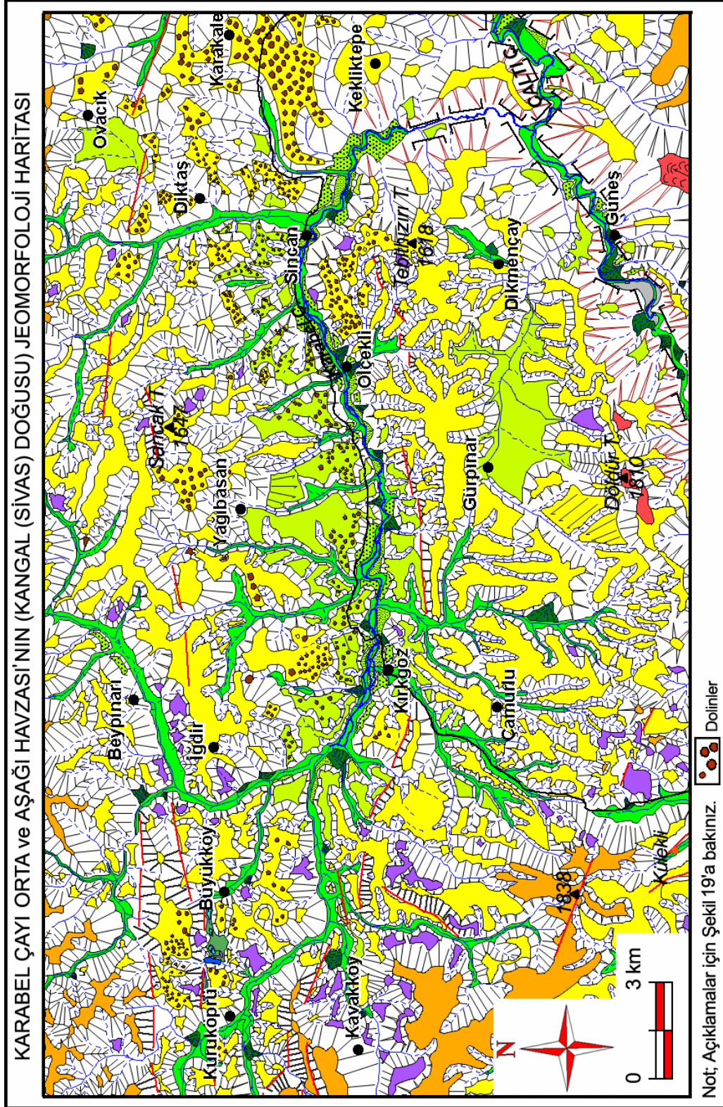
Şekil 41: Karabel Çayı Orta ve Aşağı Havzası'nın (Kangal (Sivas) doğusu) jeomorfoloji haritası
