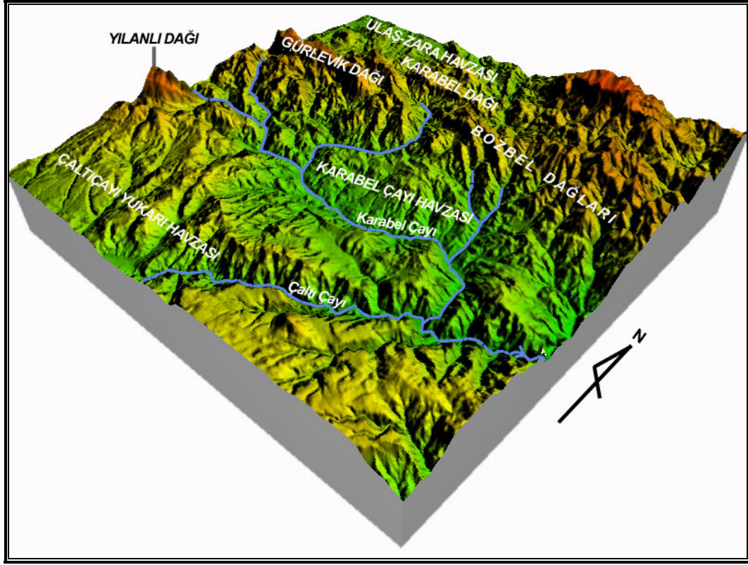
Şekil 35: Karabel Çayı Havzası'nın (Kangal) blokdiagramı (Sayısal yükselti modeline göre).
