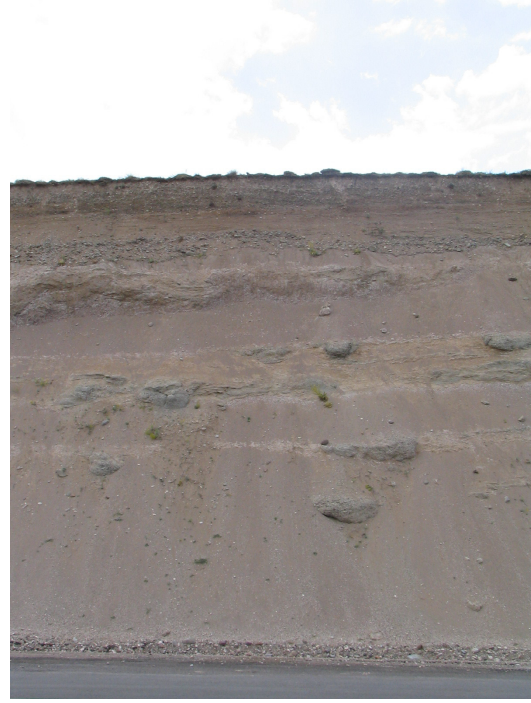
Foto 3: Çetinkaya doğusunda, Kabakçevliği güneyinde yol yarmasında Kangal Formasyonu'na ait zayıf tutturulmuş akarsu oluşukları
