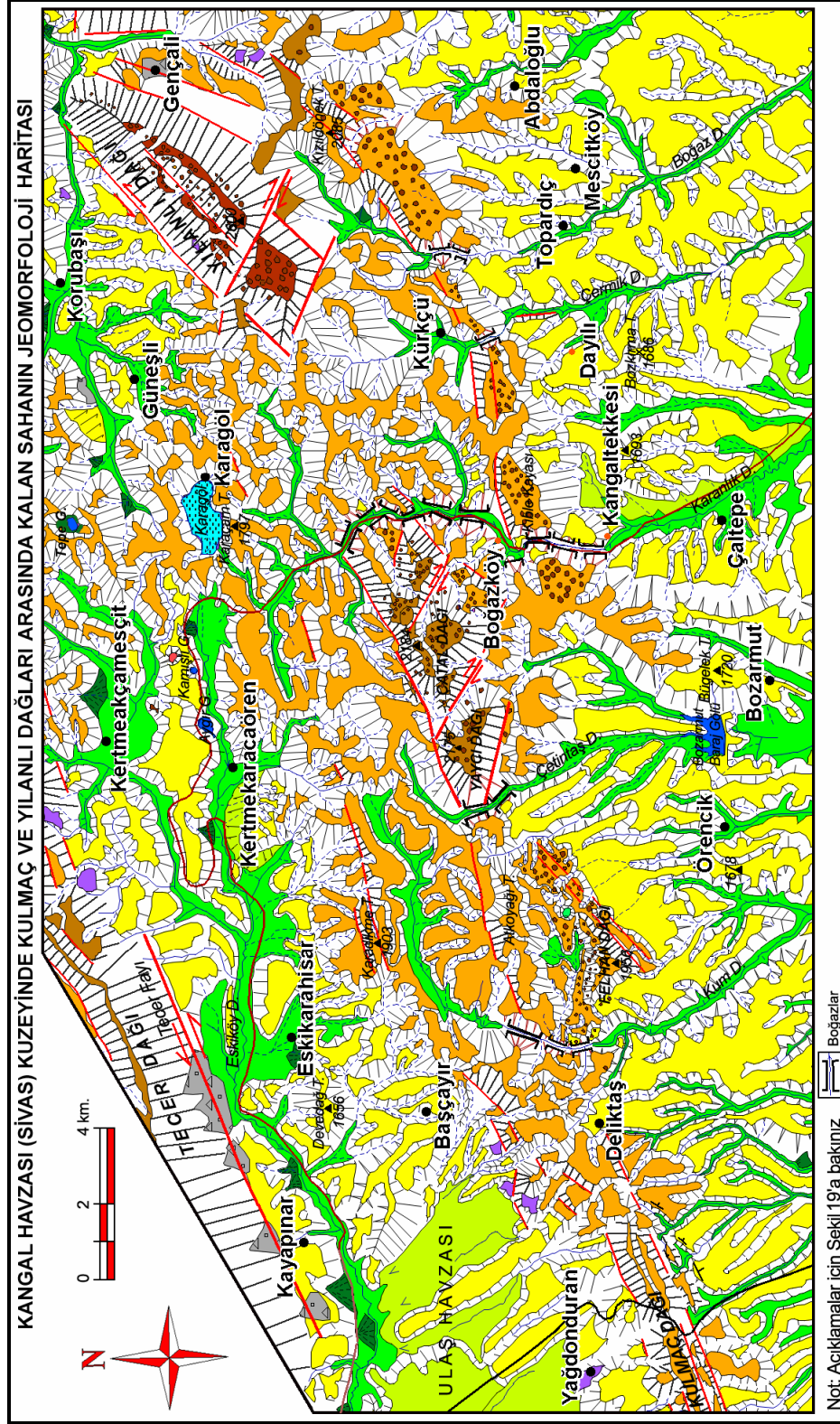
Şekil 40: Kangal Havzası'nın (Sivas) kuzeyinde Kulmaç ve Yılanlı dağları arasında kalan sahanın jeomorfoloji haritası.
