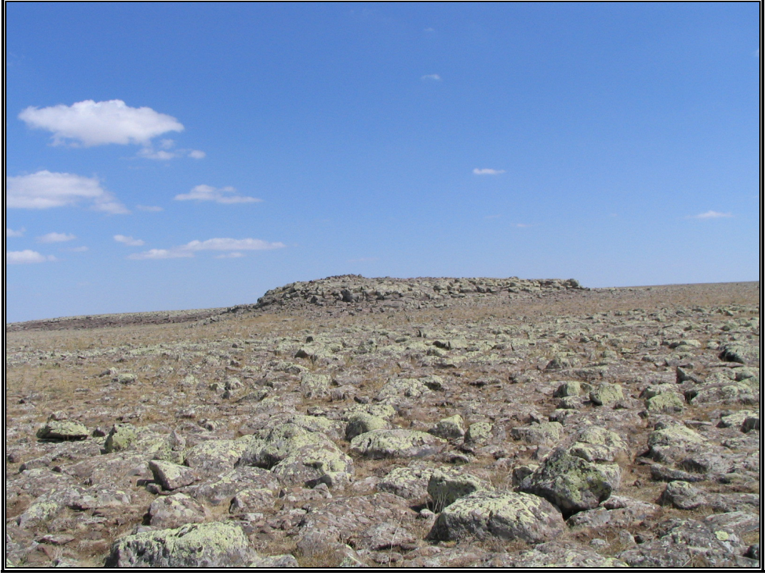
Foto 23: Mancınık kuzeyindeki Karaseki üzerinde son bazalt çıkışları sonucu oluşan Toptaşı Tepe (1708 m)
