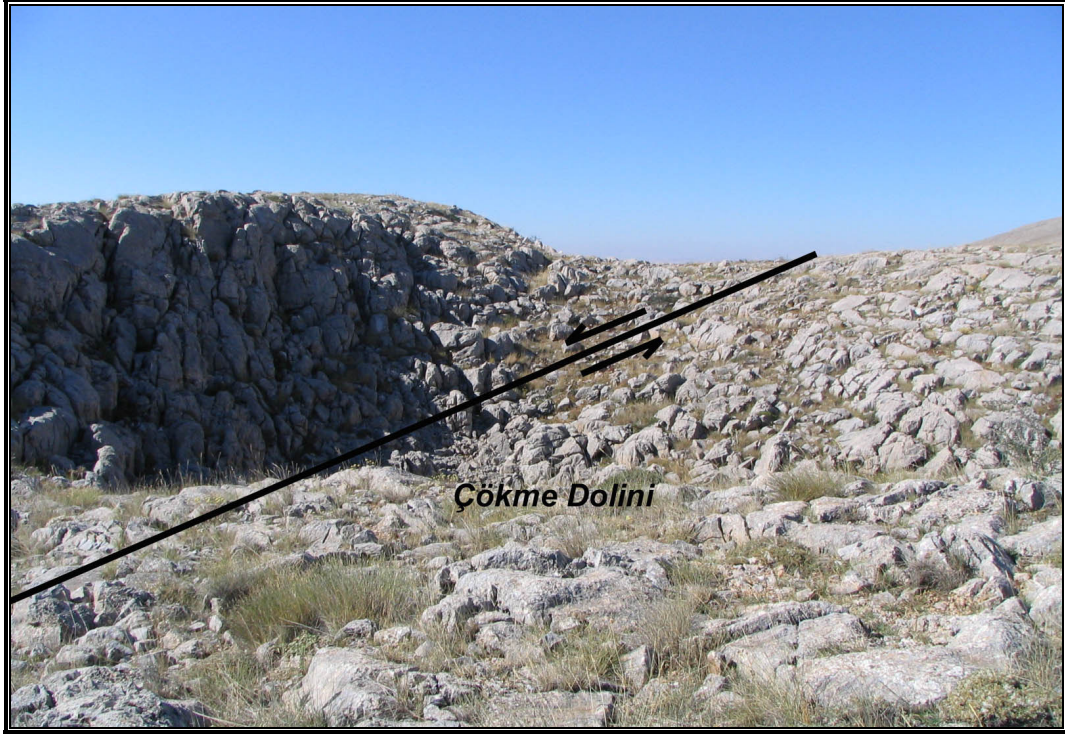
Foto 60: Atçukuru dolini güneyinde fay hattı üzerinde görülmekte olan çökme dolini
