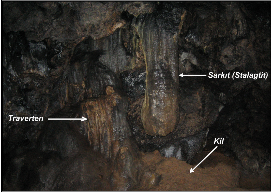
Foto 70: Damla Mağarası'nda oluşan sarkıt ve travertenler
