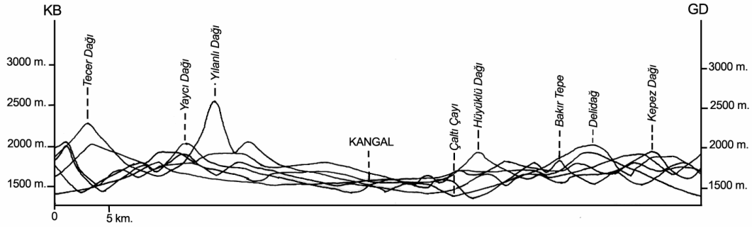
Şekil 21: Çaltı Çayı Yukarı Havzası'nda KB-GD doğrultusunda profil serilerinden oluşturulmuş enine süperimpoze (Çakıştırılmış) profilleri.
