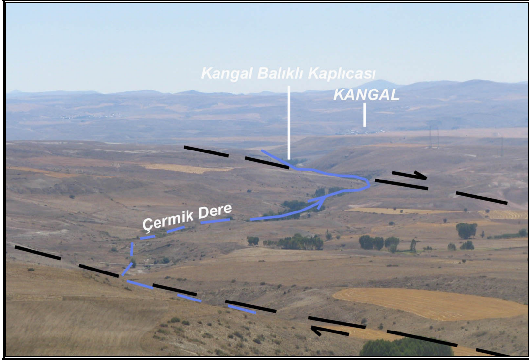
Foto 27: Dayılı doğusunda Çermik Dere Vadisi'nde görülen sağ yanal ötelenme
