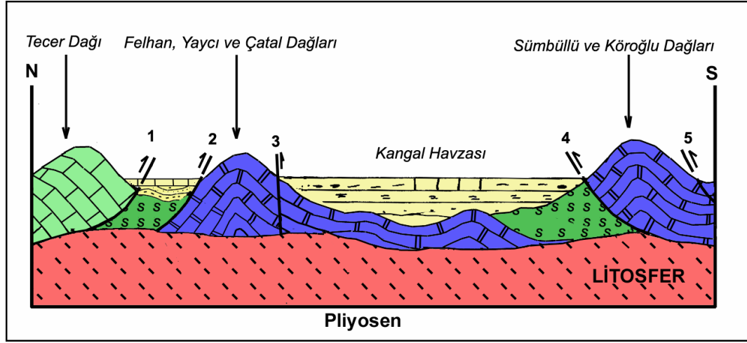
Şekil 48: Pliyosen döneminde inceleme alanının genel tektonik yapısını gösterir şematik kesit: 1-Tecer Fayı (Bindirmesi), 2-İtiran Fayı, 3-Yılanlı Fayı, 4-Kangal Fayı, 5-Demirtaş ve Reşadiye fayları
