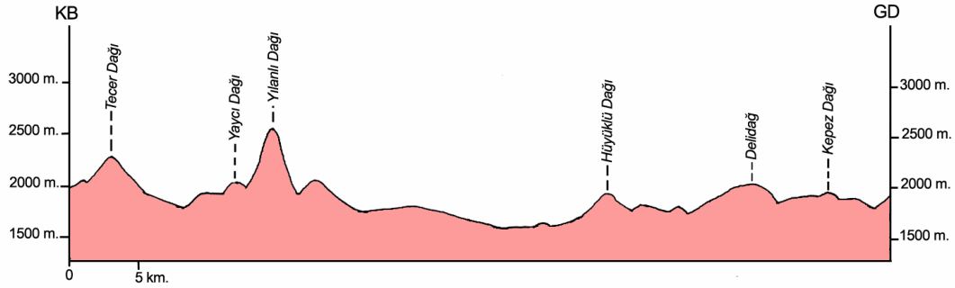
Şekil 22: Çaltı Çayı Yukarı Havzası'nın KB-GD doğrultusunda oluşturulmuş enine bileşik profili.
