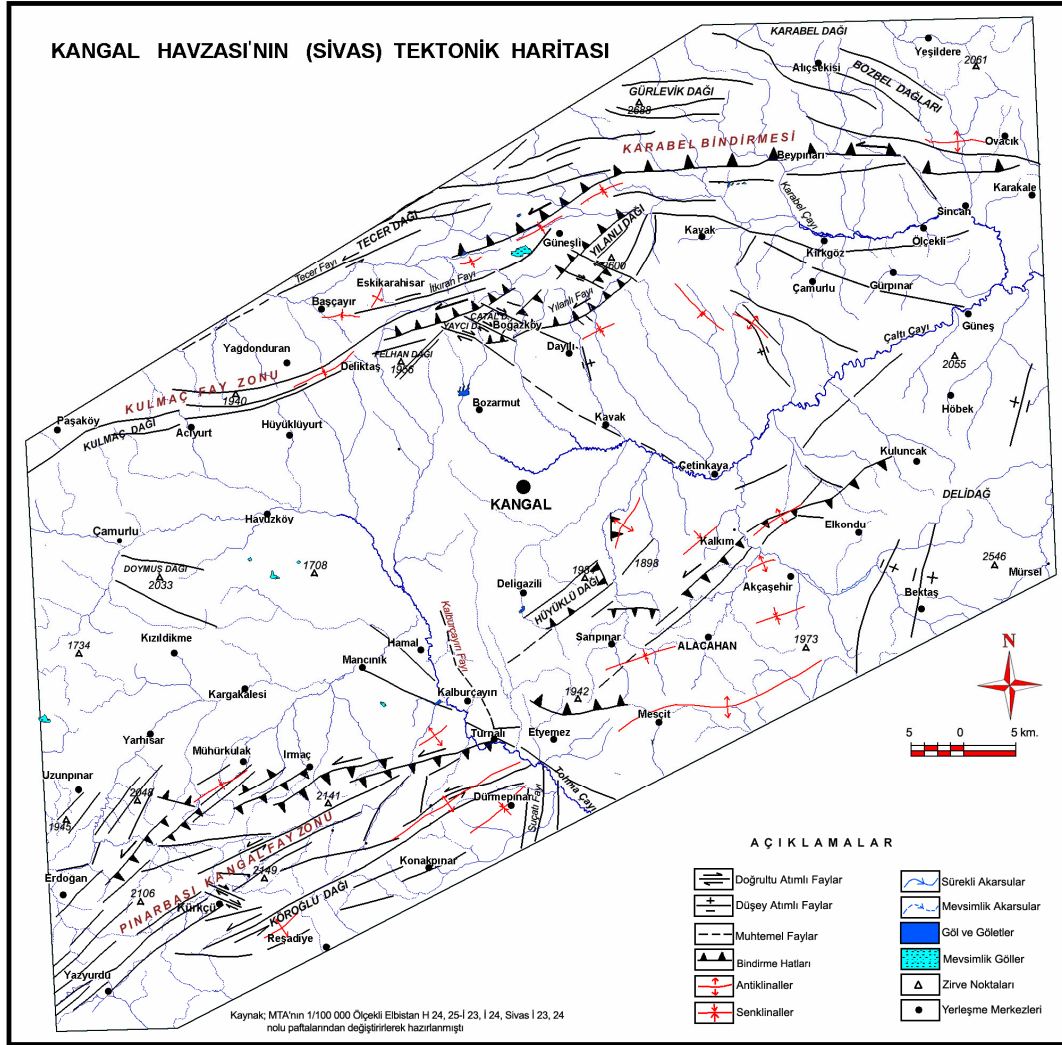
Şekil 16: Kangal Havzası'nın (Sivas) tektonik haritası
