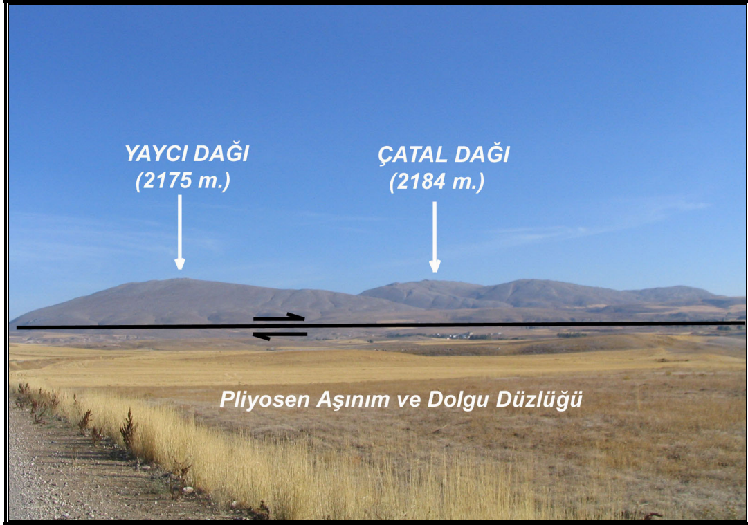
Foto 7: Kangal'ın kuzeyinde Yılanlı ve Felhan dağları arasında Mesozoyik yaşlı kireçtaşlarından oluşan Yaycı ve Çatal dağları (2175 m)
