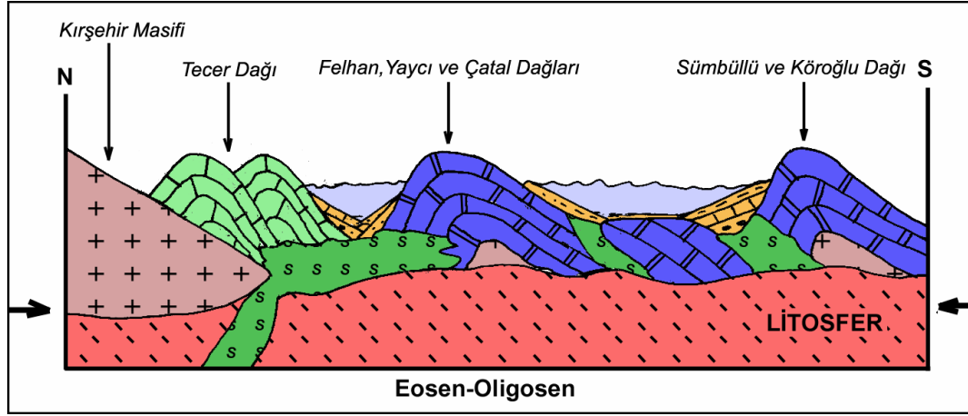
Şekil 46: Eosen-Oligosen döneminde inceleme alanının genel tektonik yapısını gösterir şematik kesit
