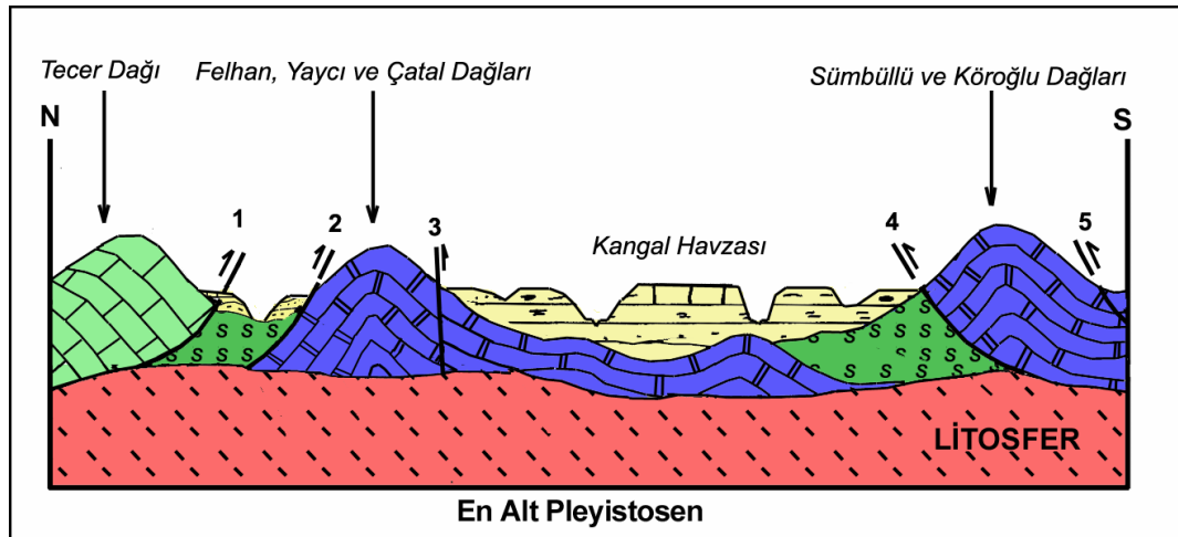
Şekil 49: En Alt Pleyistosen döneminde inceleme alanının genel tektonik yapısını gösterir şematik kesit: 1-Tecer Fayı (Bindirmesi), 2-İtkıran Fayı,3-Yılanlı Fayı, 4-Kangal Fayı,5-Demirtaş ve Reşadiye fayları
