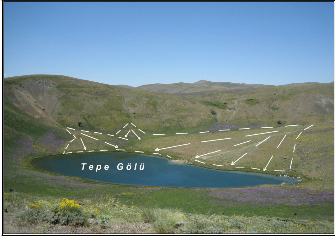
Foto 86: İtkıran batısında, İtkıran Fayı üzerinde Üst Kretase yaşlı ofiyolitler içerisinde oluşan Tepe Gölü ve çevresindeki birikinti konileri
