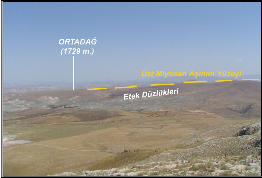
Foto 19: Kangal'ın güneyinde Hüyükli Dağı doğusunda, Mesozoyik yaşlı kireçtaşı ve ofiyolitler üzerinde görülen Üst Miyosen yaşlı aşınım yüzeyleri ve etek düzlükleri
