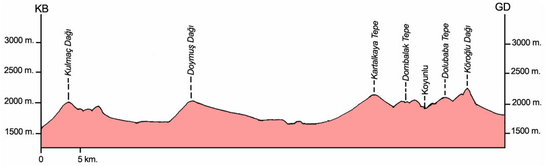
Şekil 25: Tohma Çayı Yukarı Havzası'nın KB-GD doğrultusunda oluşturulmuş enine bileşik profili.
