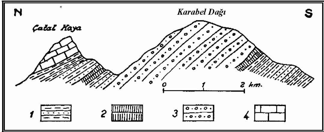
Şekil 30: Karabel Dağı'nın K-G doğrultusunda jeolojik kesiti, 1-Marn-gre (Fliş), 2-Jips (Fliş), 3- İri taneli gre (Fliş), 4- Kalker (Burdigaliyen) (Kurtman, 1961)
