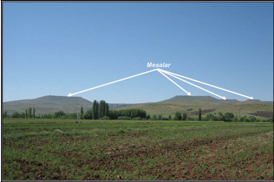
Foto 80: Karaboğaz'ın kuzey yamaçları üzerinde bazaltlara bağlı oluşan mesalar (Şahit tepeler)
