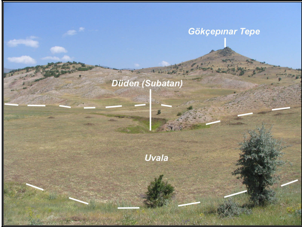
Foto 55: Karakale güneyinde, Gökçepınarı Tepe güneyinde Oligosen yaşlı jipsler üzerinde oluşan uvala tabanında görülen subatan
