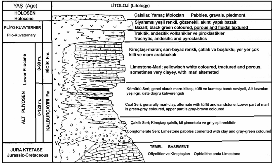
Şekil 60: Kangal-Kalburçayırı Linyit Havzası'nın stratigrafi kesiti (Narin ve Kavuşan, 1993) (ölçeksizdir)
