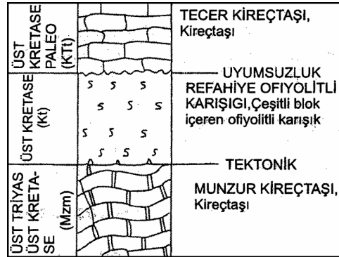
Şekil 9: Kangal Havzası'nın kuzeyinde Munzur Kireçtaşları ile diğer birimler arasındaki tektonik ilişki (Atabey ve Aktimur, 1997)
