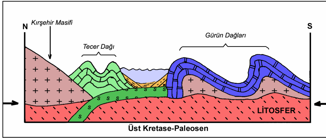
Şekil 45: Üst Kretase-Paleosen döneminde inceleme alanının genel tektonik yapısını gösterir şematik kesit
