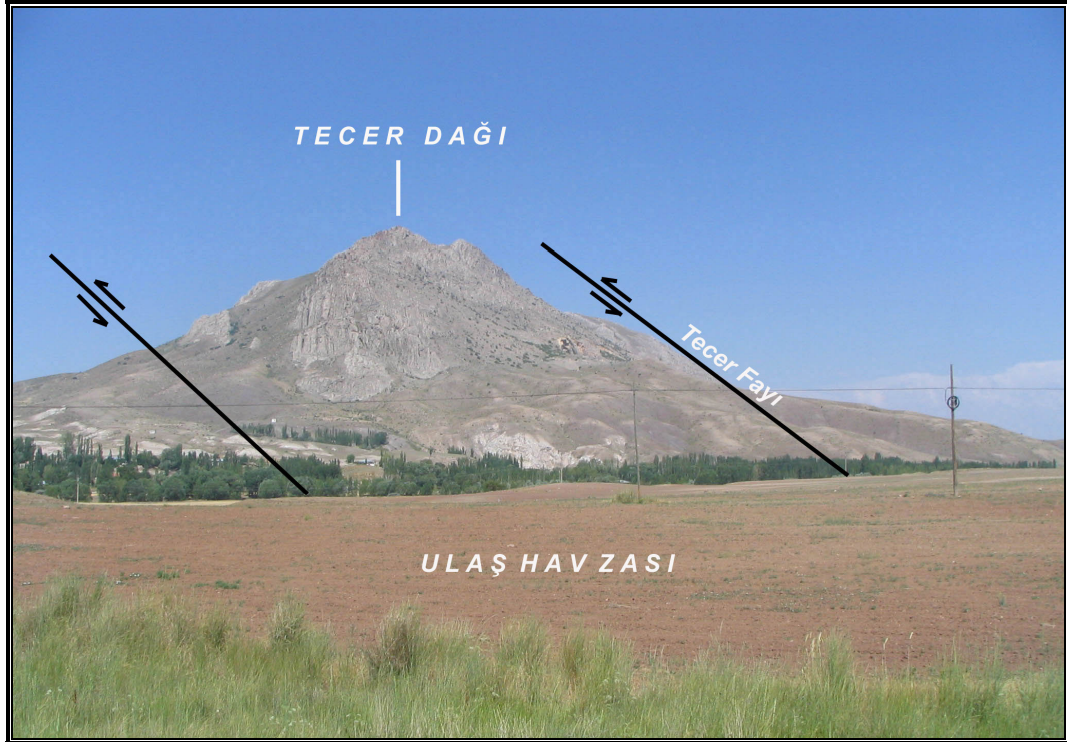
Foto 9: İnceleme alanının kuzeyinde Ulaş Havzası ile Kangal Havzası'nı birbirinden ayıran Tecer Dağları ve Tecer Fayı (Bindirmesi)
