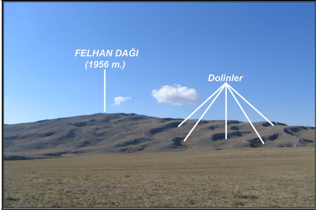
Foto 57: Kangal’ın kuzeyinde Mesozoyik yaşlı kireçtaşlarından oluşan Felhan Dağı kuzey yamaçlarında görülen erime dolinleri
