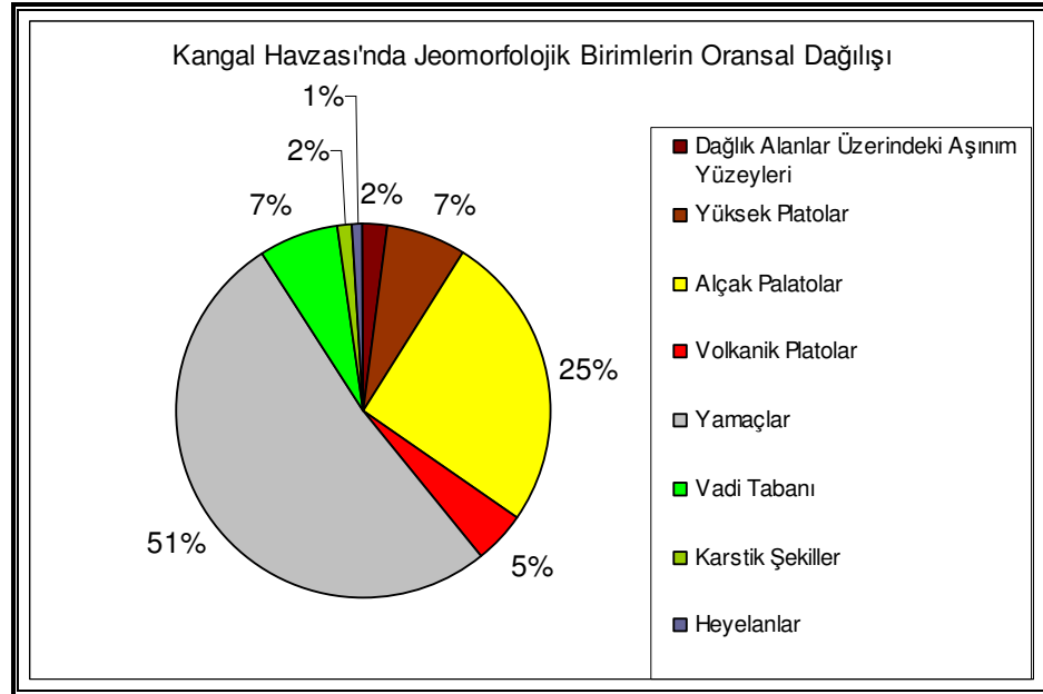
Şekil 20: Kangal Havzası'nda jeomorfolojik birimlerin oransal dağılışı
