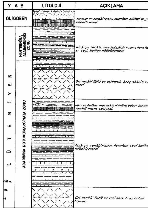
Şekil 12: Karabel Çayı Havzası'nın kuzey ve kuzeydoğusunda Karabel ve Bozbel dağlarında yüzeyleyen Bozbel Formasyonu'nun stratigrafik kesiti (Kurtman, 1973)
