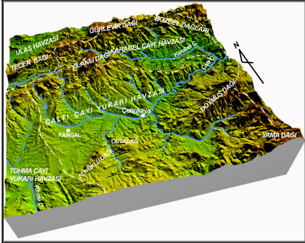
Şekil 34: Çaltı Çayı Yukarı Havzası (Kangal) ile Karabel Çayı Havzası'nın blokdiagramı (Sayısal yükselti modeline göre)
