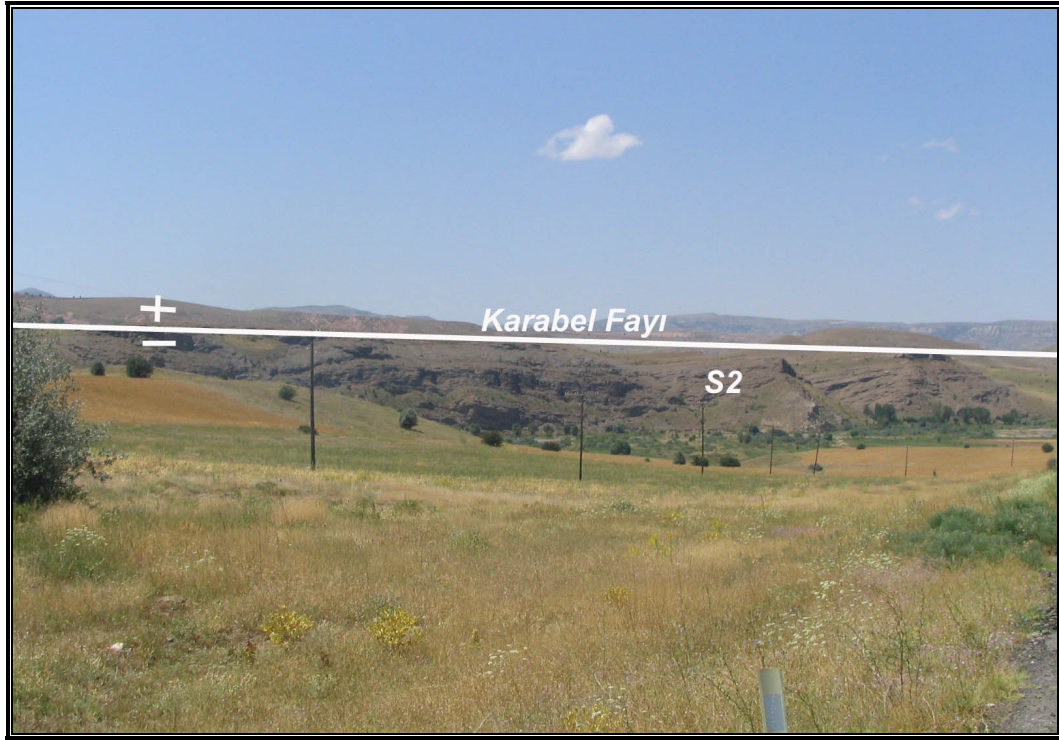
Foto 42: Gürpınar kuzeyinde Karabel Çayı Vadisi'nde çarpılmış yüksek sekiler
