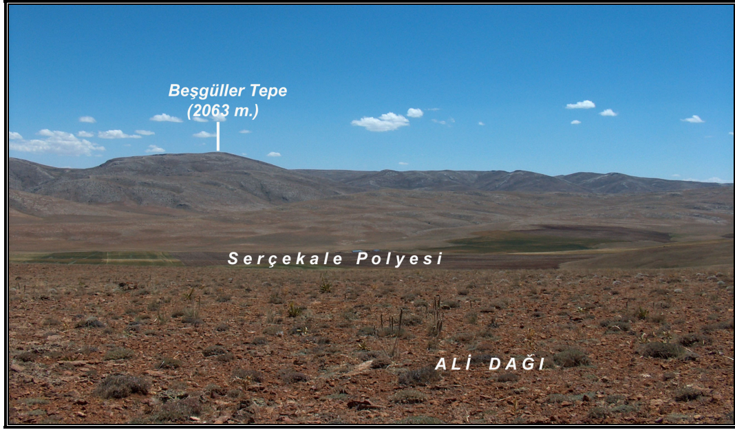
Foto 62: Uzunpınar güneyinde KD-GB doğrultusunda uzanan Serçekale Polyesi
