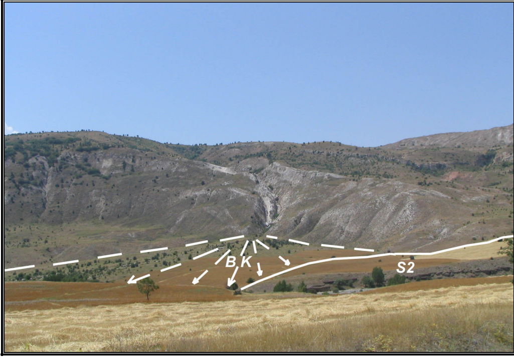
Foto 44: Sincan güneydoğusunda Karabel Çayı üzerinde görülen birikinti konisi sekisi ve alçak seki
