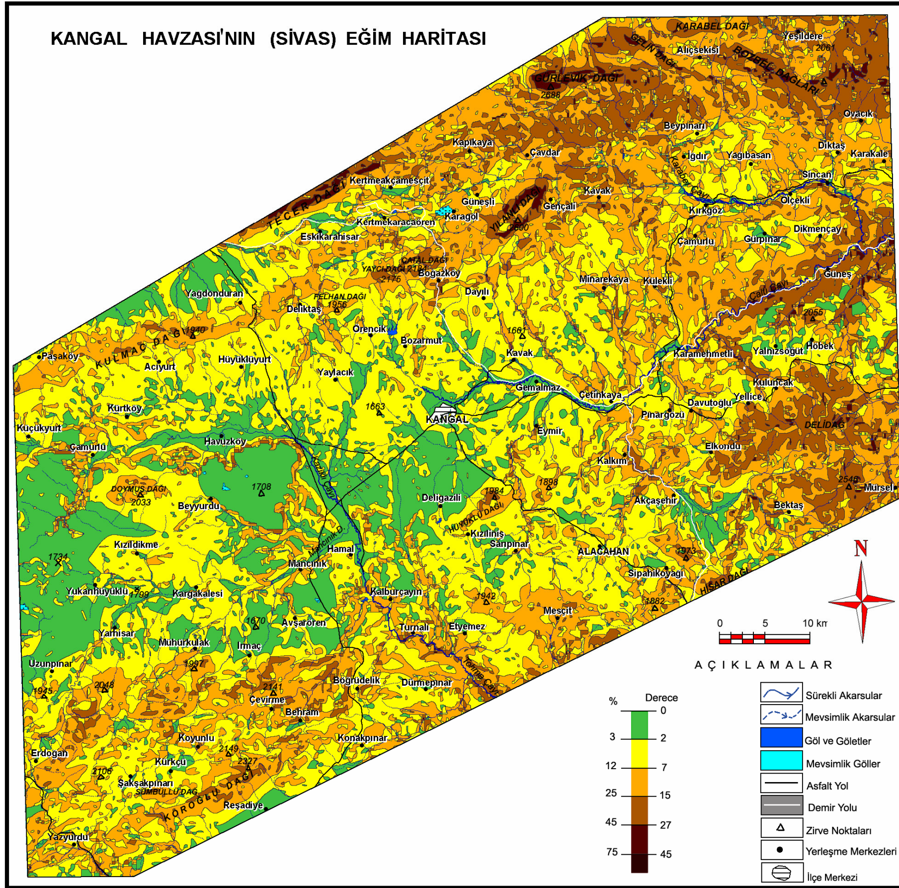
Şekil 27: Kangal Havzası'nın (Sivas) eğim haritası
