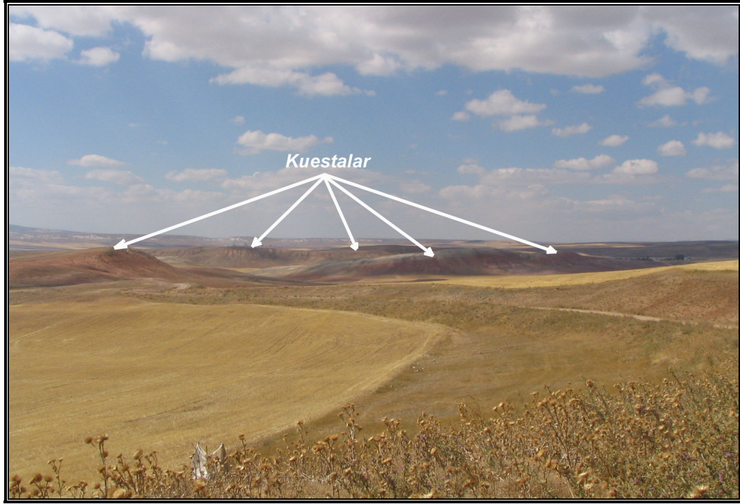
Foto 75: Acıyurt doğusunda havza tabanına geçişte görülen kuestalar
