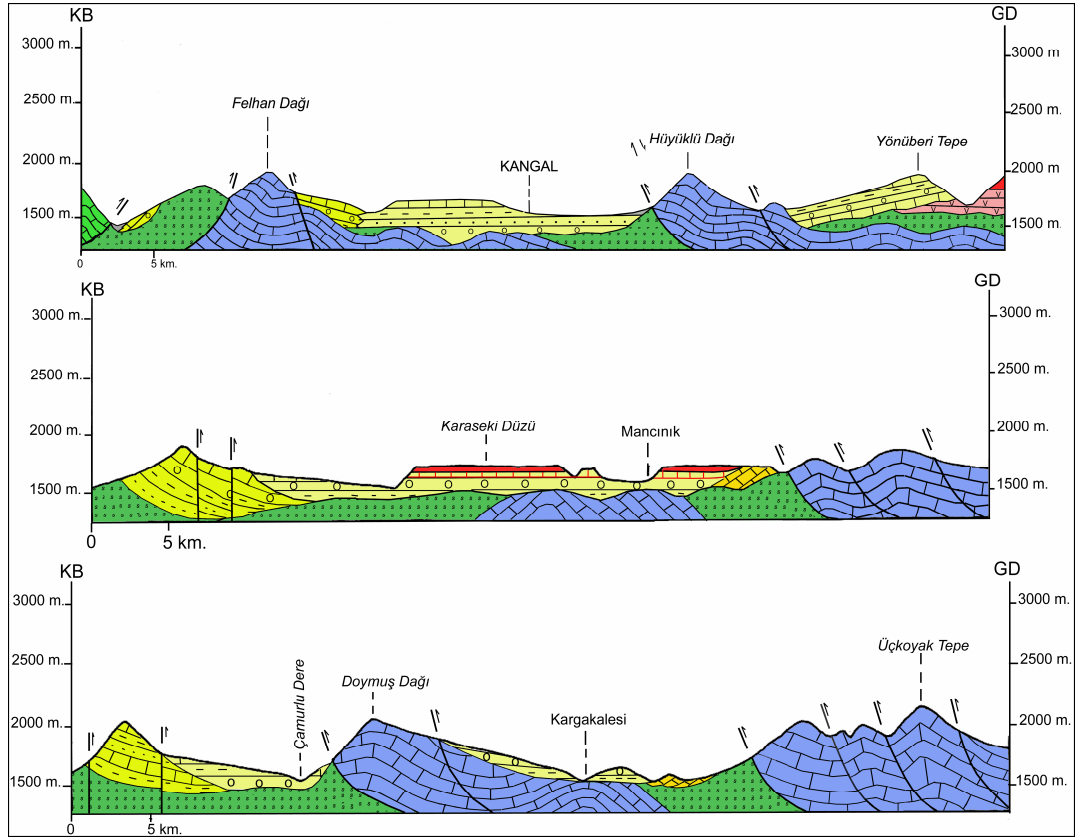
Şekil 17: Kangal Havzası’na ait KB-GD doğrultulu jeolojik kesitler (Açıklamalar için Şekil 7’ye bakınız)
