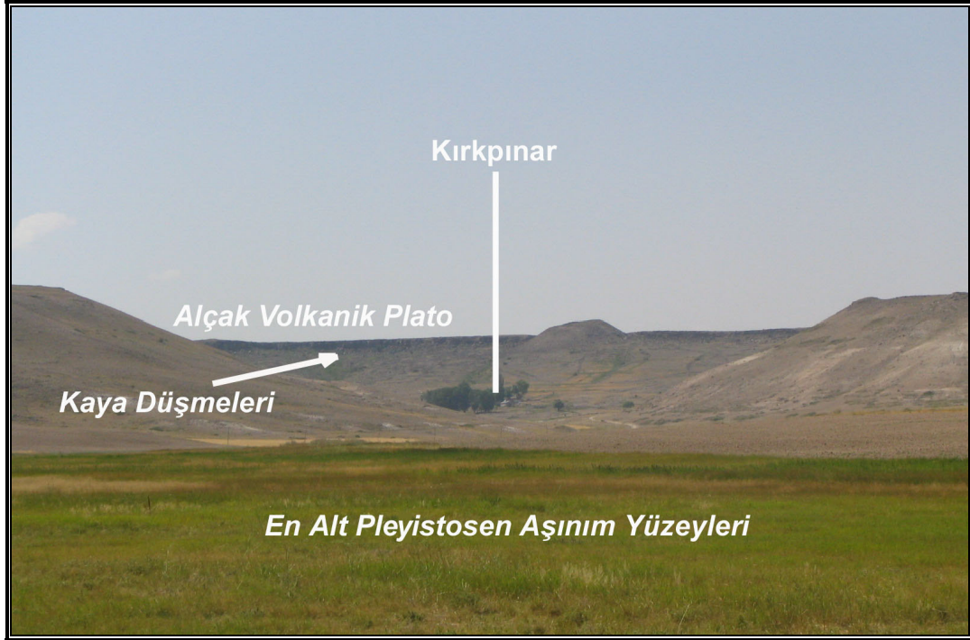
Foto 50: Mancınık kuzeyinde Kırkpınar çevresinde yerleşme alanlarının terk edilmesine neden olan kaya düşmeleri
