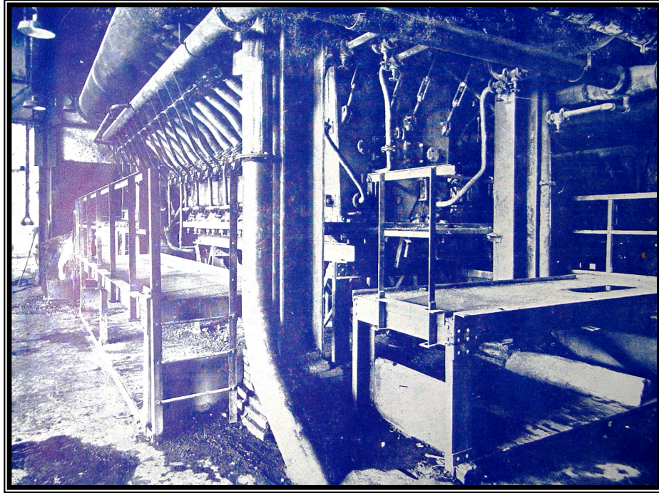
Resim 21 – Water-Jacket fırınının boşaltış kısmı ( Bakır 1949 adlı eserden alınmıştır.)
