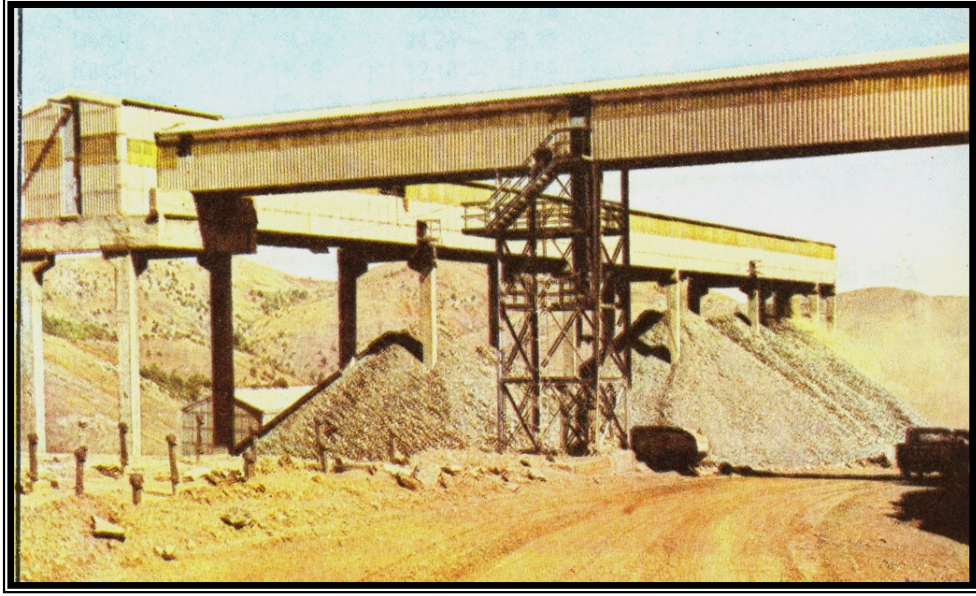
Resim 16 – Kaba kırmadan geçen cevher stok alanında ( Maden 1986 İlçe Yıllığı adlı eserden alınmıştır.)
