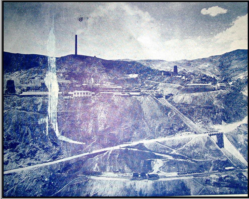
Resim 8 – Ergani Bakır İşletmesi’nin 1940’lardaki genel görünümü ( Bakır 1949 adlı eserden alınmıştır.)
