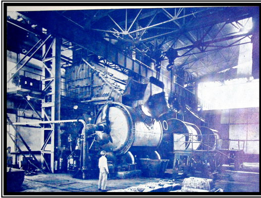
Resim 11 – Konverterler (Bakır 1949 adlı eserden alınmıştır.)
