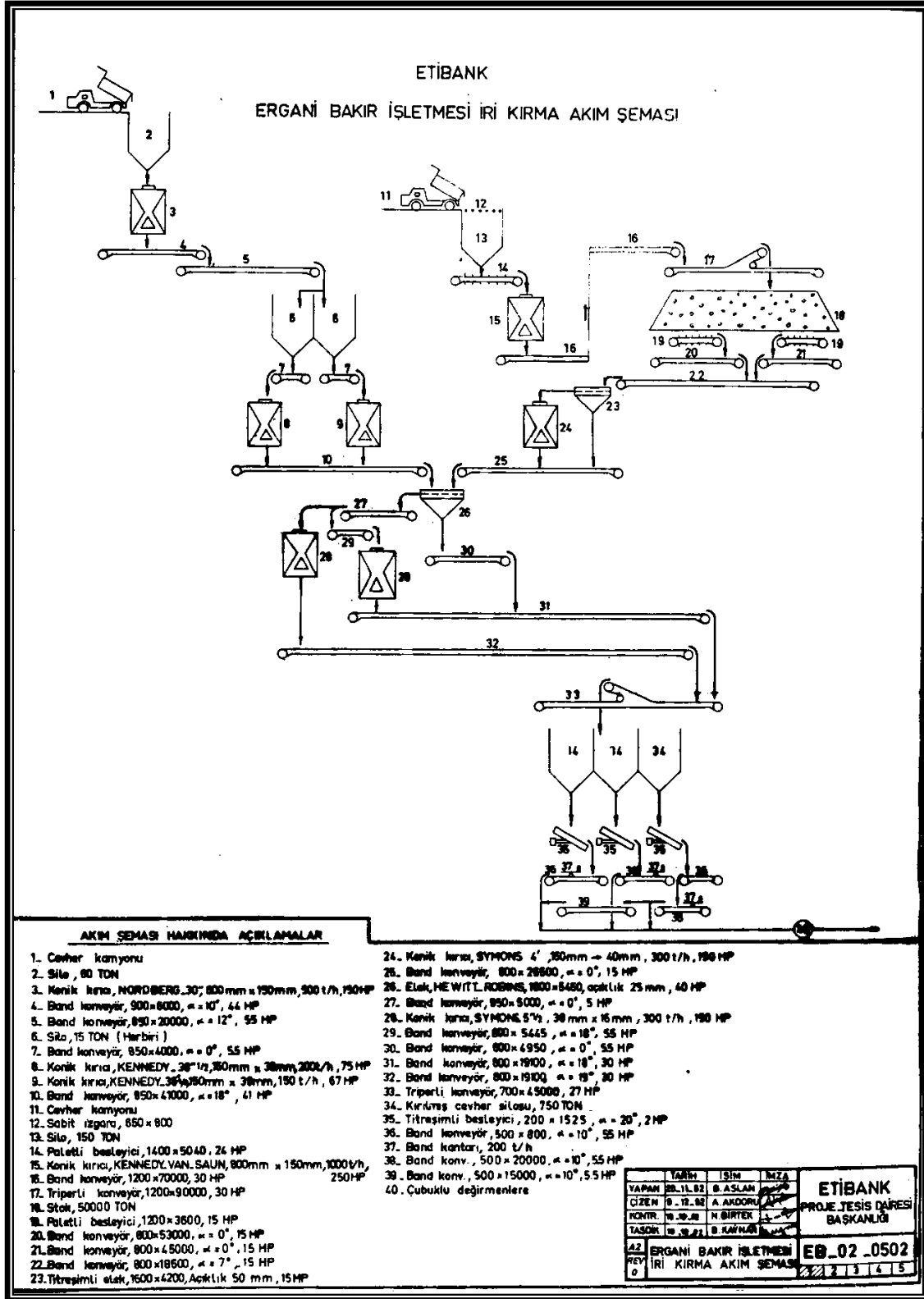
Şema 2 – EBI İri Kırma Akım Şeması (Etibank Bülteni dergisinden alınmıştır.)
