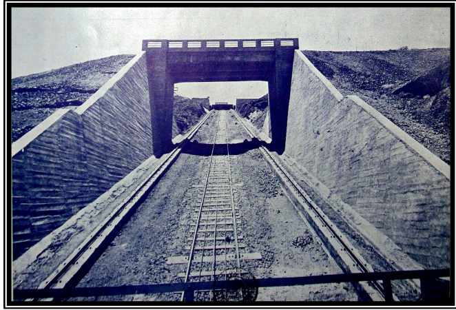
Resim 6 - Vagonların taşınması için yaptırılan asansör
