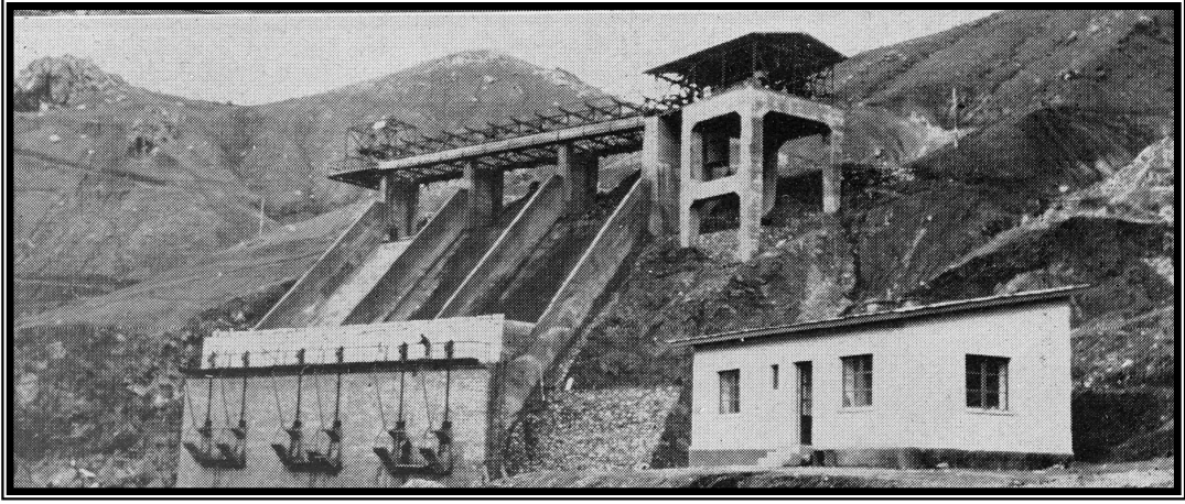
Resim 30 – Guleman’dan hava hattı ile gelen Guleman kromlarının boşaltılması için Maden’de yaptırılan bölüm (Halk arasında burası Boşaltma diye bilinmektedir) (Bayındırlık İşleri Dergisi’nden alınmıştır.)
