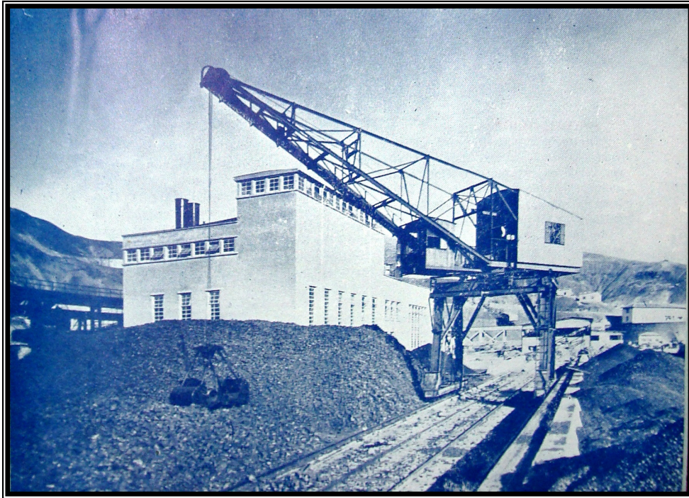
Resim 34 – İşletme alanındaki çalışmalardan bazı görüntüler (Bakır 1949 adlı eserden alınmıştır.)
