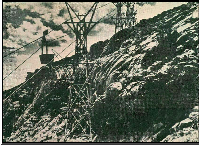
Resim 8 - Guleman kromlarını Ergani'ye getiren hava hattından yüksek bir nokta (MTA Enstitüsü Dergisi'nden alınmıştır.)
