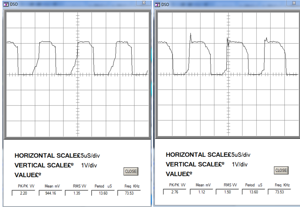
Şekil 6.18. V_G=200V giriş gerilimi için Q_A anahtarı V_{CE} gerilimi (solda) ve Q_B anahtarı V_{CE} gerilimi (sağda).
