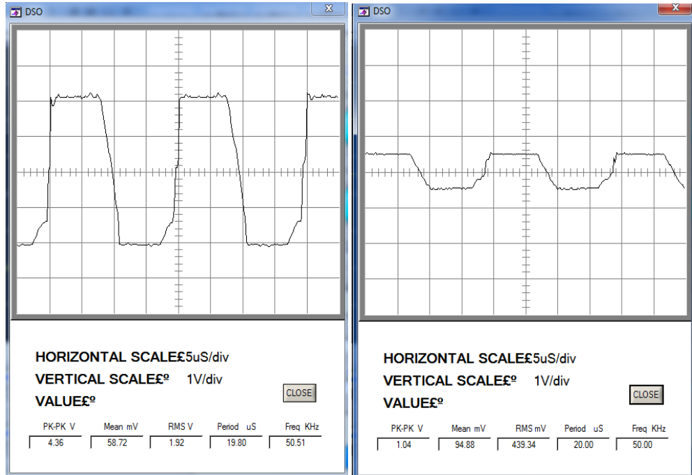
Şekil 6.13. V_G=200V giriş gerilimi için primer (solda) ve sekonder gerilimi (sağda).
