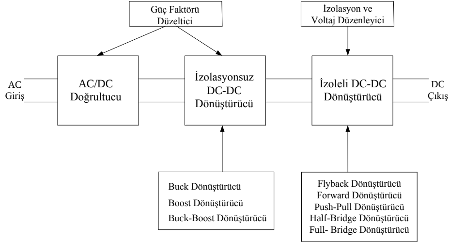
Şekil 2.3. SMPS 'lerin sistem yapıları [18].
