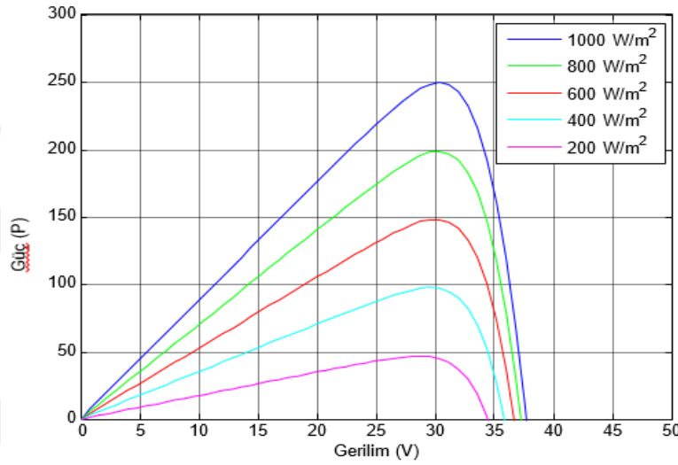
Şekil 2.17. Farklı ışınlma miktarları altında elde edilen güç-gerilim grafiği
