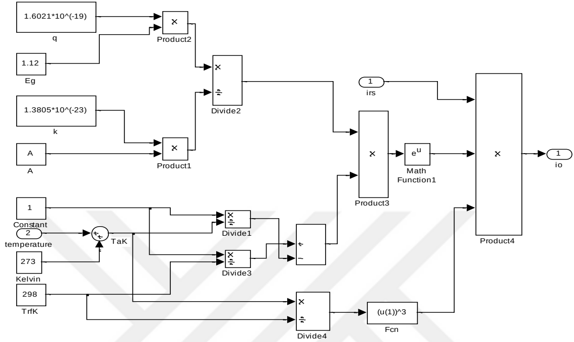
Şekil 2.13. I_0 'a ait Matlab Simulink modeli
