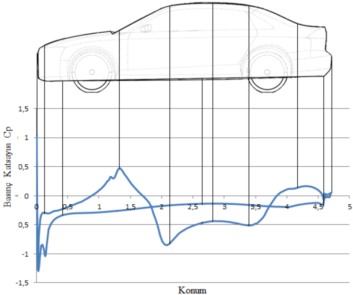
Şekil 3. 21. X=0, simetri eksenini boyuncaya orijinal aracın tüm gövdesinde oluşan basınç dağılımı
