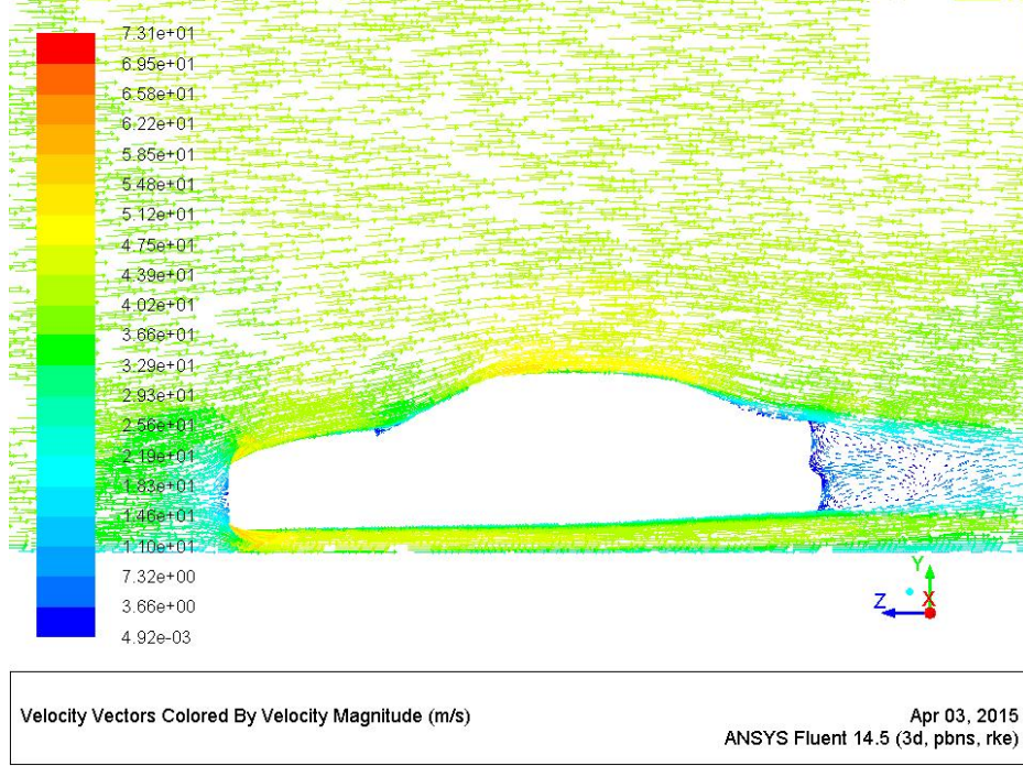
Şekil 3. 19. X=0, simetri ekseni boyunca yeniden tasarlanan araç üzerinde oluşan hız vektörleri
