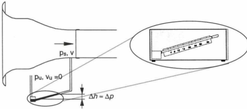
Şekil 2. 8. Akış hızı ölçme sistemi
