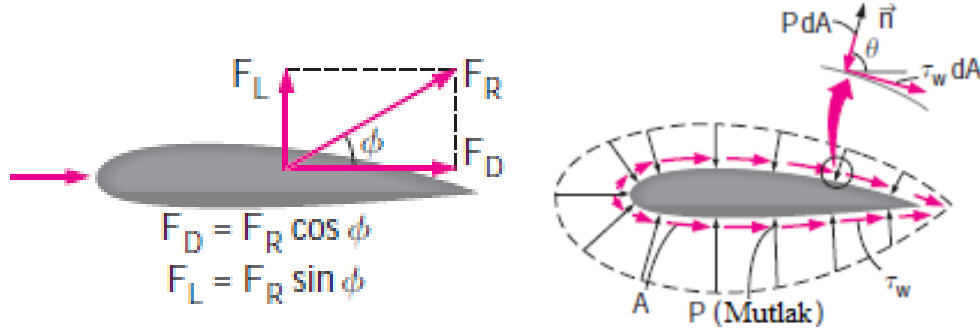
Şekil 1. 10. İki boyutlu bir cisim üzerine etki eden basınç kuvveti ve viskoz kuvvet ile bileşke, kaldırma ve direnç kuvvetleri [19].
