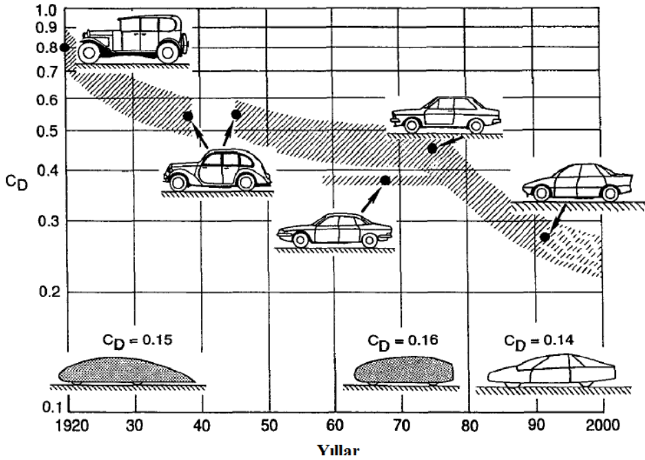
Şekil 1. 1. Araçların aerodinamik direnç katsayısının tarihçesi [16].
