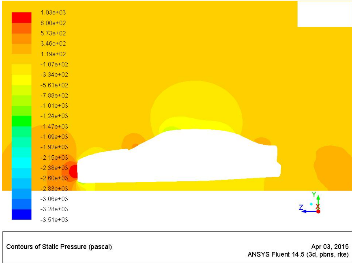
Şekil 3. 12. X=0, simetri eksenini boyuncu yeniden tasarlanan araç üzerinde oluşan basınç konturları
