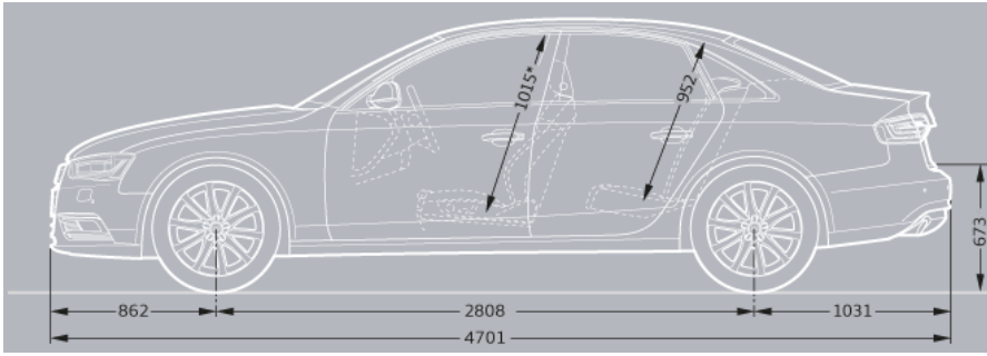
Şekil 1.2. Audi A4 modelinin yan görünüşü
