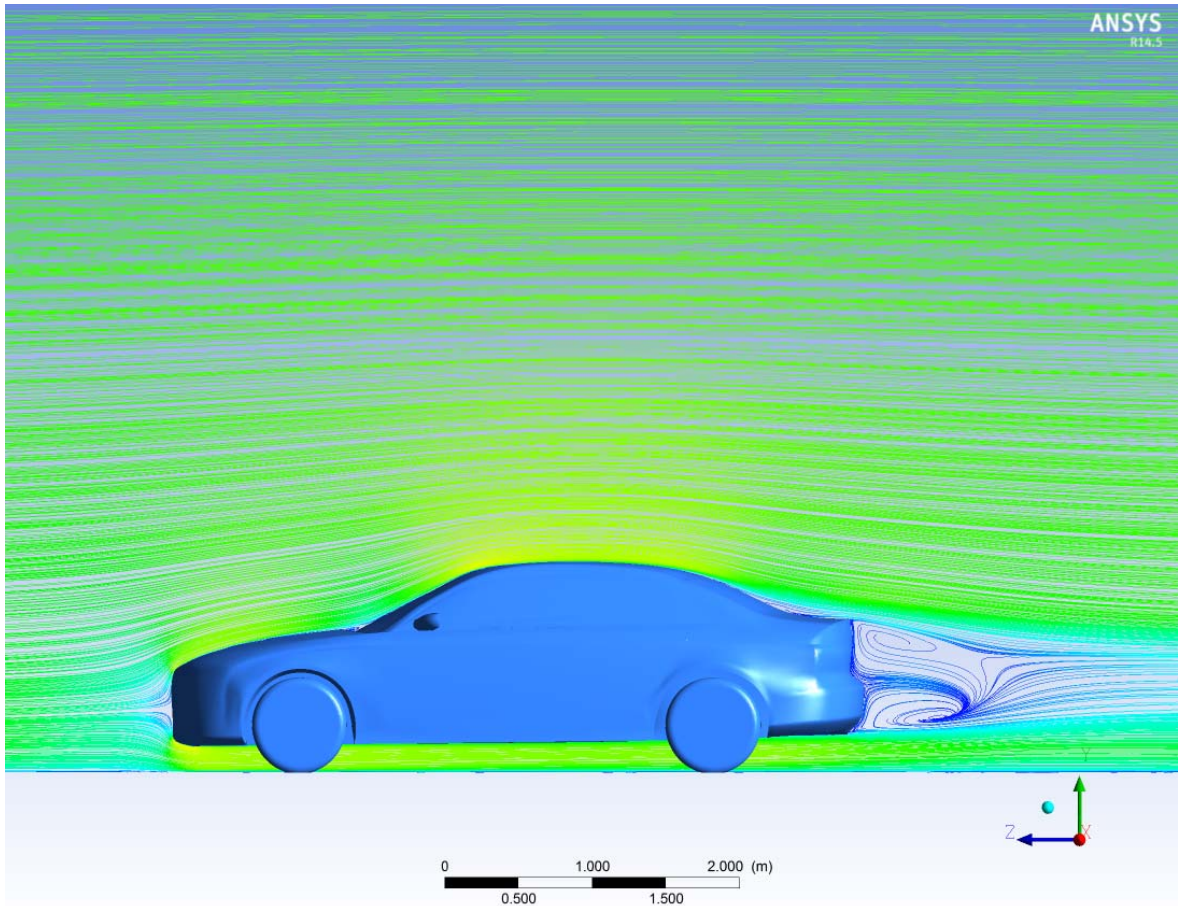
Şekil 3. 15. X=0, simetri eksenini boyunda orijinal araç üzerinde oluşan akım çizgileri
