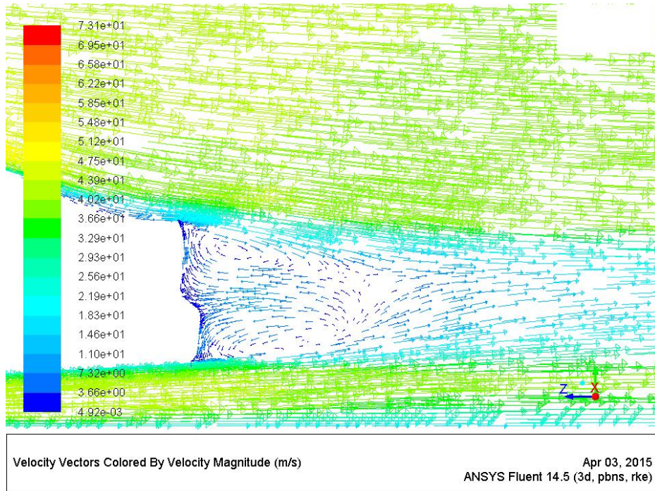
Şekil 3. 20. X=0, simetri ekseni boyunca yeniden tasarlanan aracın arka tarafında oluşan art izi bölgesi
