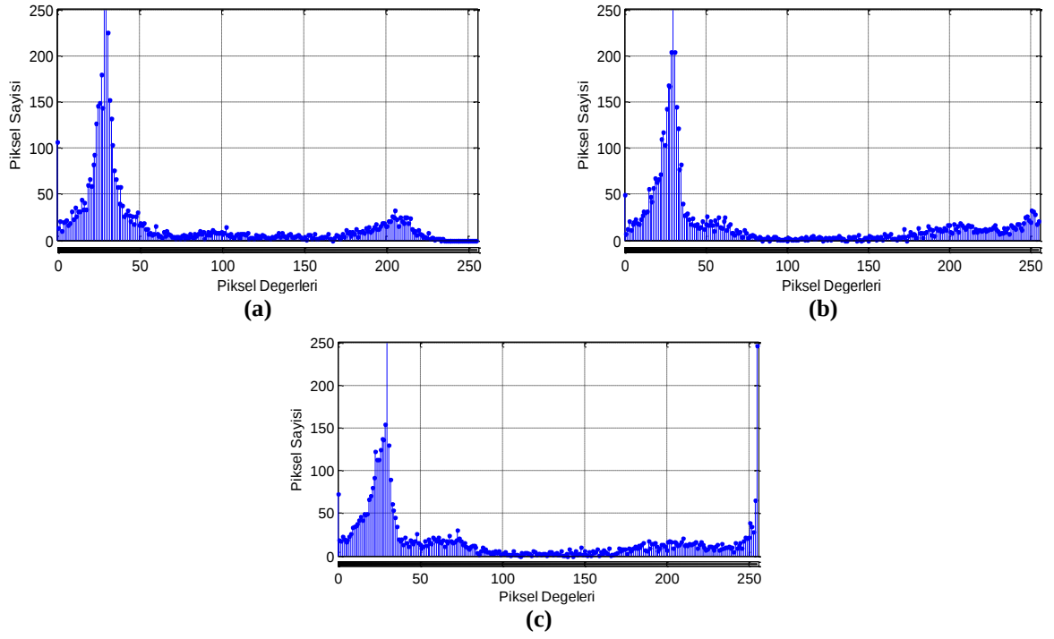
Şekil 4.18. Temas noktasında sağlam ve ark oluşmuş termal görüntülerin kesit alanlarının histogramı (a) Sağlam termal görüntünün kesit alanının histogramı (b) Temas noktası ısınan termal görüntünün kesit alanının histogramı (c) Ark oluşmuş termal görüntünün kesit alanının histogramı
