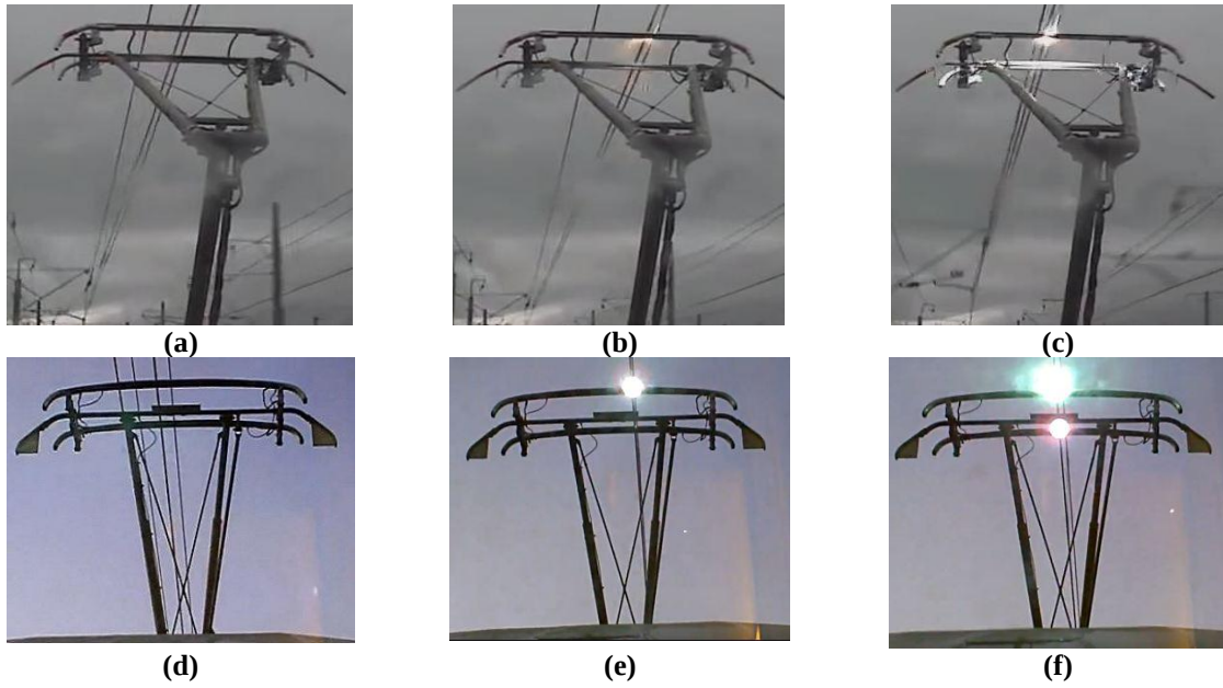
Şekil 3.29. Pantograf ark tespiti için kullanılan farklı videolardan farklı durumlarda alınan pantograf görüntüleri (a) Video 1, Frame = 1 (b) Video 1, Frame = 50 (c) Video 1, Frame = 100 (d) Video 2, Frame = 1 (e) Video 2, Frame = 50 (f) Video 2, Frame = 100
