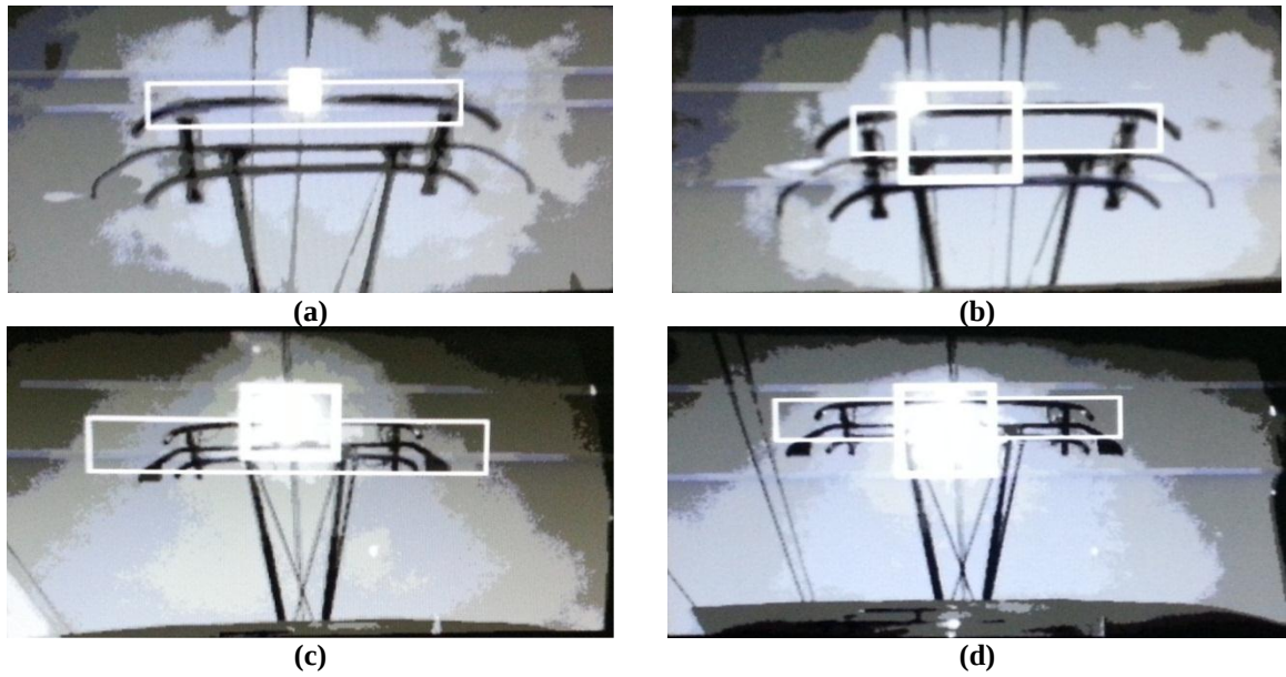
řekil 5.15. rnek bir pantograf katener grntsnde FPGA ile elde edilen sonular (a) Bir yerde oluřan ark grnts (b) Birden fazla yerde oluřan ark grnts (c) Farklı bir grntde bir yerde oluřan ark grnts, (d) Farklı bir grntde birden fazla yerde oluřan ark grnts
