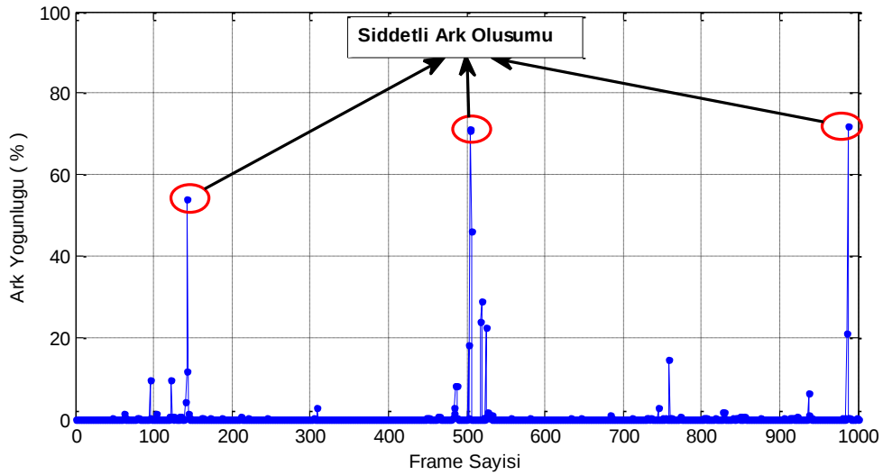
Şekil 3.35. Önerilen ark tespiti yönteminin 1000 Frame için uygulanması
