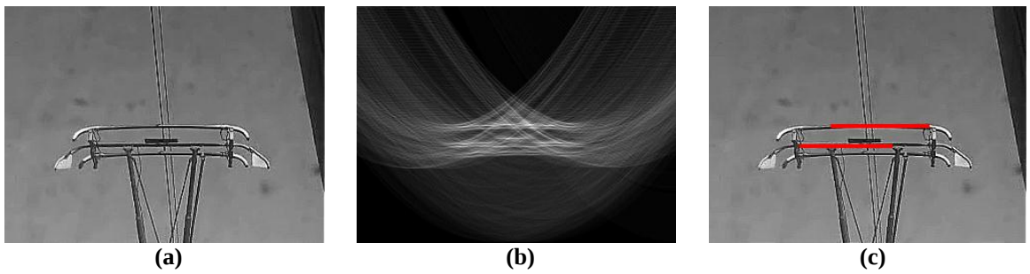
Şekil 3.16. Pantograf ve katener sistemin Hough dönüşümünün uygulanması (a) Gri görüntü (b) Hough dönüşümü (c) Görüntüdeki doğruların elde edilmesi
