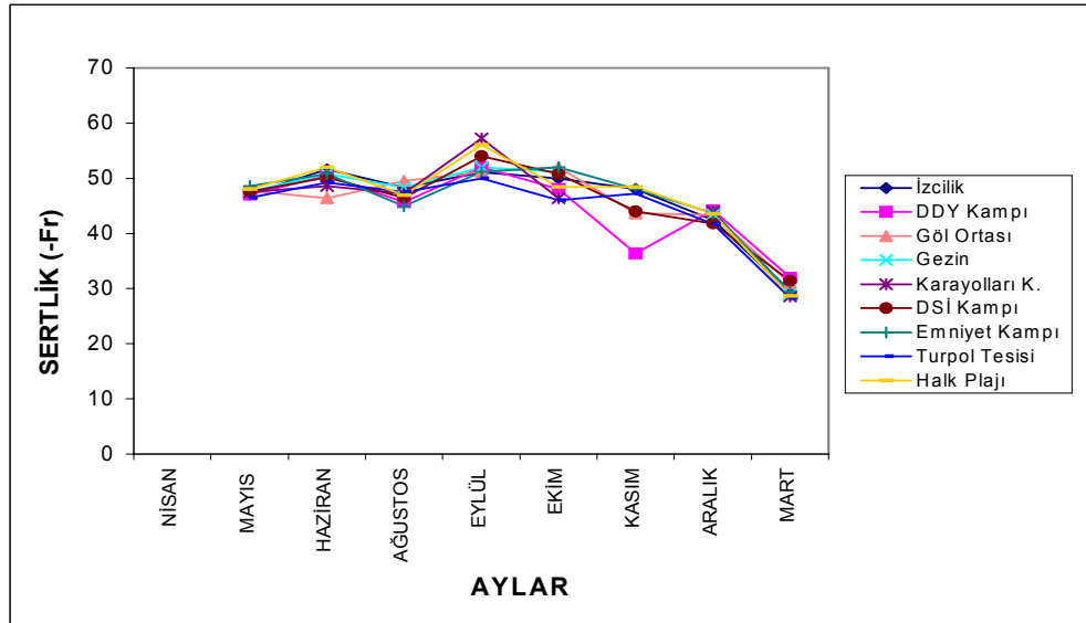
Şekil 4.10 Hazar Gölü'nde Ölçülen Sertlik Değerlerinin Zamana Bađlı Deđişimleri
