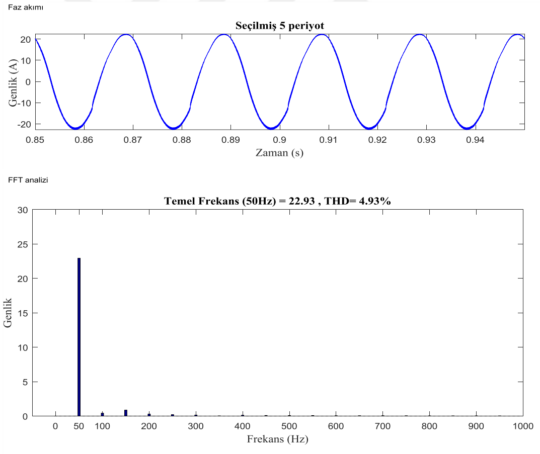
Şekil 5.23. Yüken bir fazına ait a) Çıkış hat akımı b) Harmonik spektrumu
