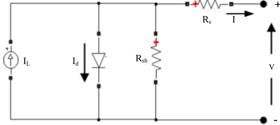
Şekil 5.12. FV hücrenin eşdeğer devresi [23]
