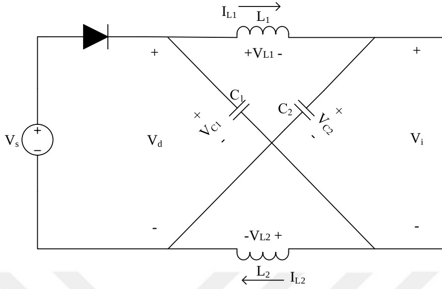
Şekil 4.4. DA baradan bakıldığında empedans kaynaklı eviriciye ait eşdeğer devre
