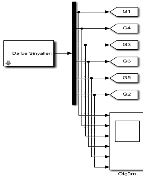
Şekil 5.2. Z-kaynak evirici için anahtarlama sinyallerinin benzetim modeli
