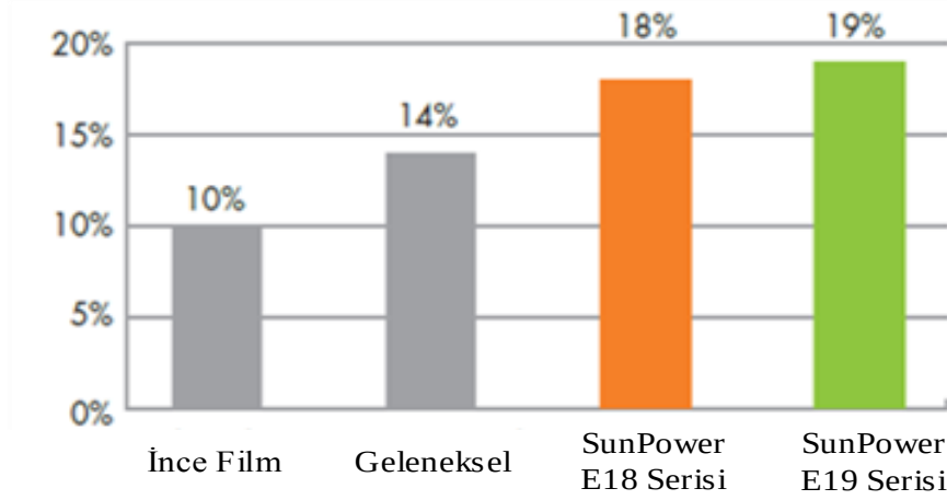
Şekil 5.15. SunPower SPR-305E-WHT-D tipi FV panelin verimlilik grafiği
