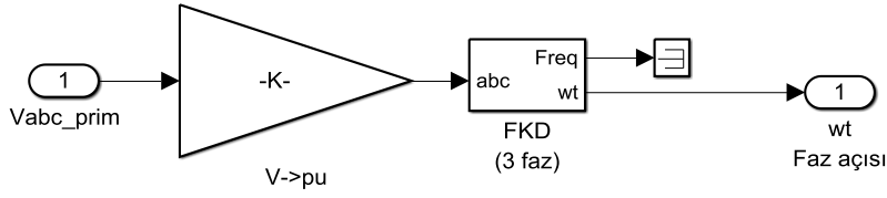
Şekil 5.17. FKD ölçüm bloğu
