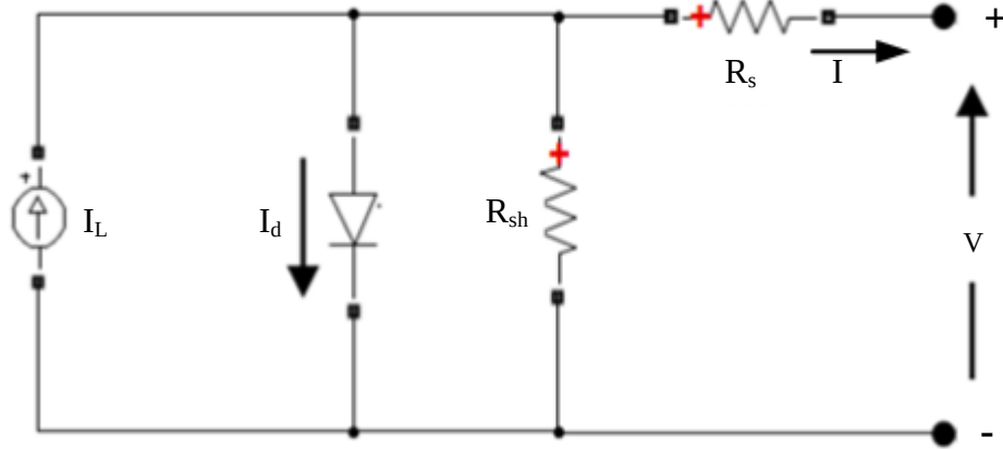
Şekil 2.7. FV panel eşdeğer devresi [23].
