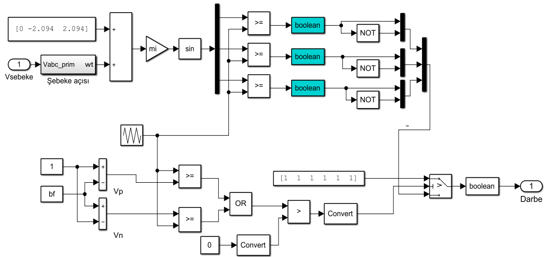
Şekil 5.18. FKD ölçüm bloğu eklenmiş SDGM anahtarlama modeli
