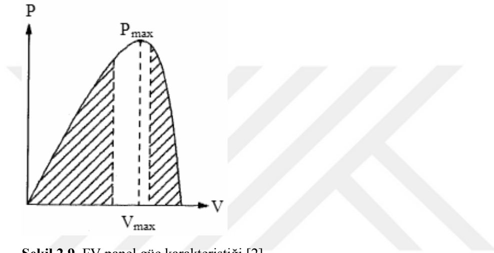
Şekil 2.9. FV panel güç karakteristiėi [2].
