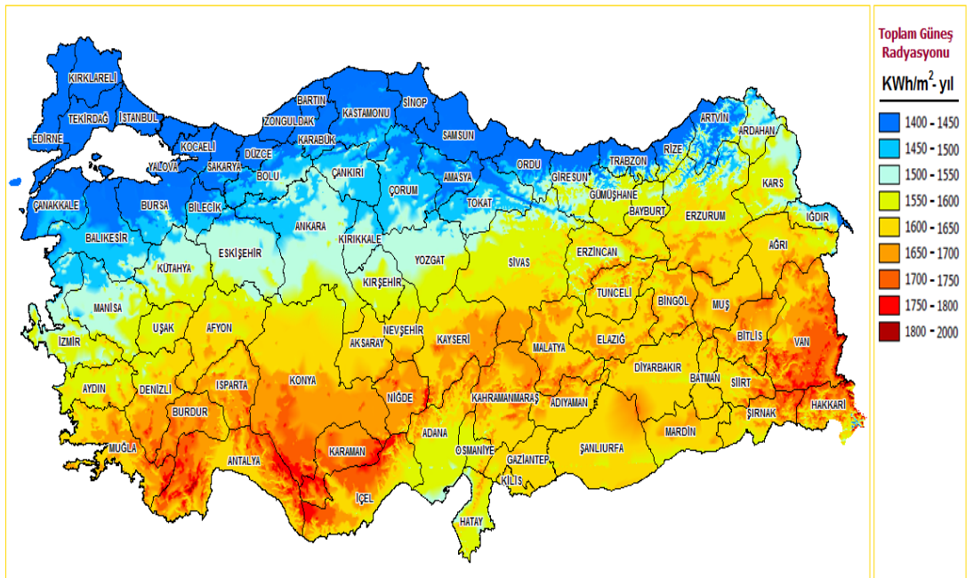
Şekil 2.1. Güneş enerjisi potansiyel atlası [20].
