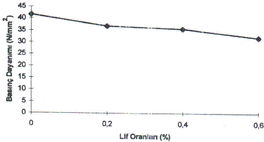
Şekil 5. Lif Oranlarına Bağlı Olarak Basınç Dayanımlarının Değişimi
