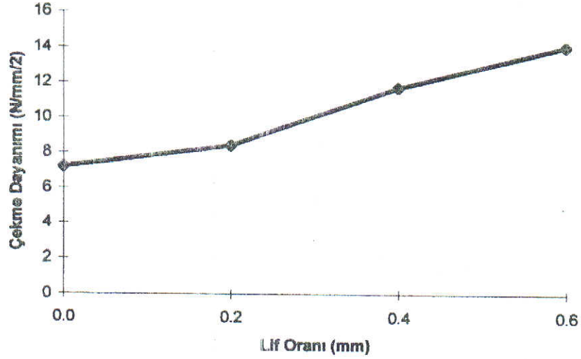
Şekil 4. Lif Oranlarına Bağlı Olarak Çekme Dayanımının Değişimi
