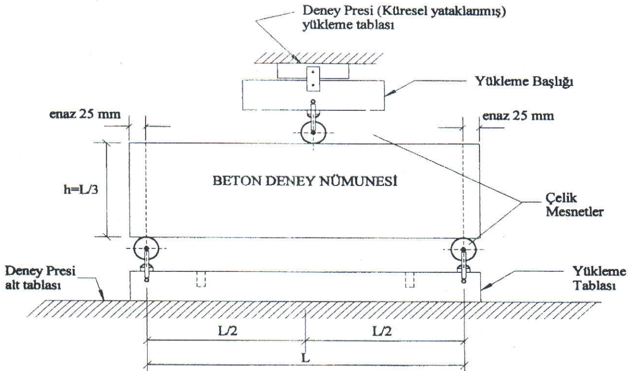
Şekil 2. Kırılma Dayanımında Üç Noktadan Yüklenmiş Basit Kirişin Yükleme Başlığı ve Yükleme Tablası Durumu
