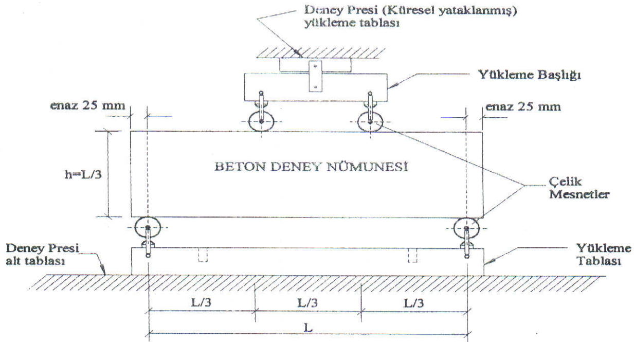
Şekil 3. Kırılma Dayanımında Dört Noktadan Yüklənmiş Basit Kirişin Yükleme Başlığı ve Yükleme Tablası Durumu
