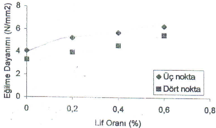
Şekil 6. Lif Oranlarına Bağlı Olarak Eğilme Dayanımlarının Değişimi
