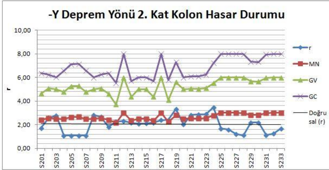
Şekil 4.14. -Y Deprem Yönü 2. Kat Kolon Hasar Durumu
