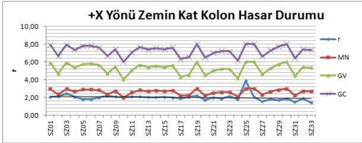
Şekil 4.5. +X Deprem Yönü Zemin Kat Kolon Hasar Durumu
