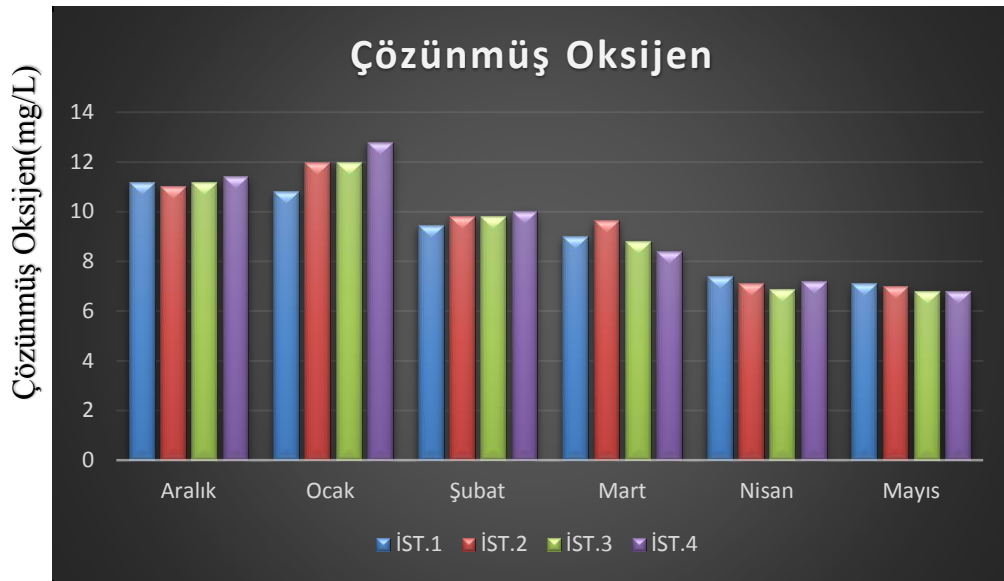
Şekil 3.4. Garzan Baraj Gölü'nün çözülmüş oksijen konsantrasyonlarının (mg/L) istasyonlara ve aylara göre değişimi.
