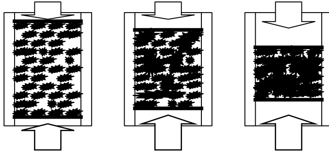
Şekil 2.6. Toz sıkıştırma kademeleri (Koç, 2002).
