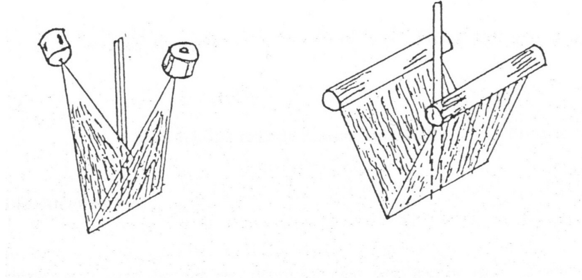
Şekil 2.2. Yassı Hüzmeli V Jetleri (Kurt, 1994).
