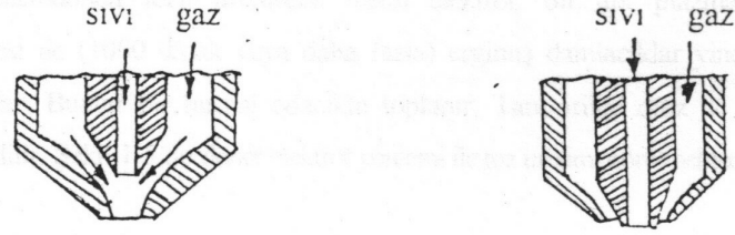
Şekil 2.3. İçte ve dışta karışma (Kurt, 1994; Koç, 2002).
