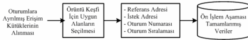
Şekil 5.4. Özellik indirgeme akış şeması
