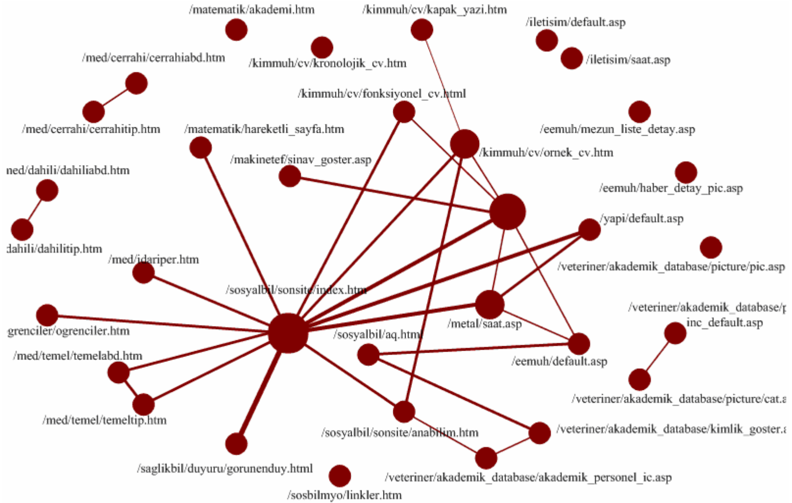
Şekil 7.5. Köprü bağlantı grafiği
