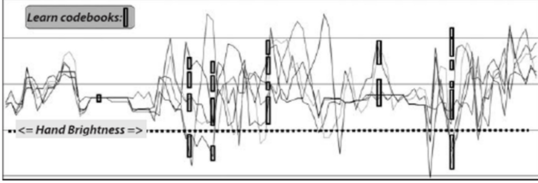
Şekil 4.27. Seçilmiş altı piksel (dikey kutular olarak gösterilmiştir) ağaç yaprağındaki dalgalanmalar için öğrenilen kod çizelgesi girdilerinin yoğunluk paylarıdır. Kod çizelgesi kutuları çoklu ayrık değerleri alır. Böylece kesikli dağıtımları daha iyi bir şekilde modelleyebilen pikselleri içerir; böylece ortalama değeri arkaplan piksellerinin alabileceği değerler arasında olan bir önplan elini (noktalı çizgideki değeri) algılayabilirler. Bu durumda kod çizelgeleri, tek boyutlu olup sadece yoğunlukta meydana gelen değişiklikleri temsil eder.
