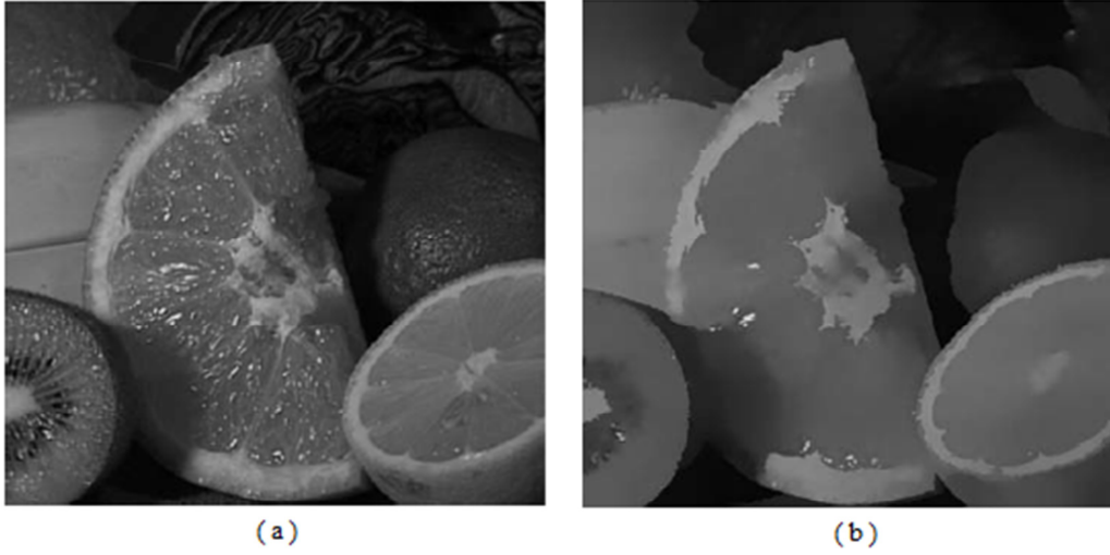
Şekil 4.34. Mean-Shift (Ortalama-Kayma) Bölütlemesi: \text{max\_level}=2 , \text{spatialRadius}=20 , ve \text{colorRadius}=40 parametreleriyle cvPyrMeanShift Filtering() kullanılarak ölçekle yapılan mean-shift bölütlemesi; şimdi benzer alanlarda benzer değerler mevcut olup böylelikle süper piksel olarak işlenebilir. Bu da ardından yapılan işlemi hızlandırabilir.(a) ham resim. (b) işlenmiş resim
