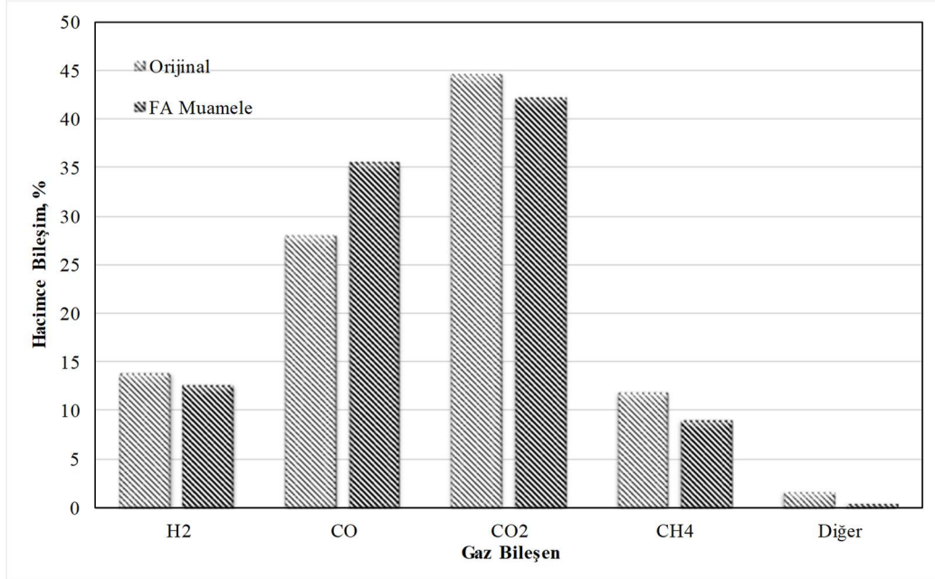
Şekil 4.10. Orijinal ve fosforik asitle muamele edilmiş MDF tozlarının 400 °C’de pirolizi sırasında elde edilen kondense olmayan gazın bileşimi
