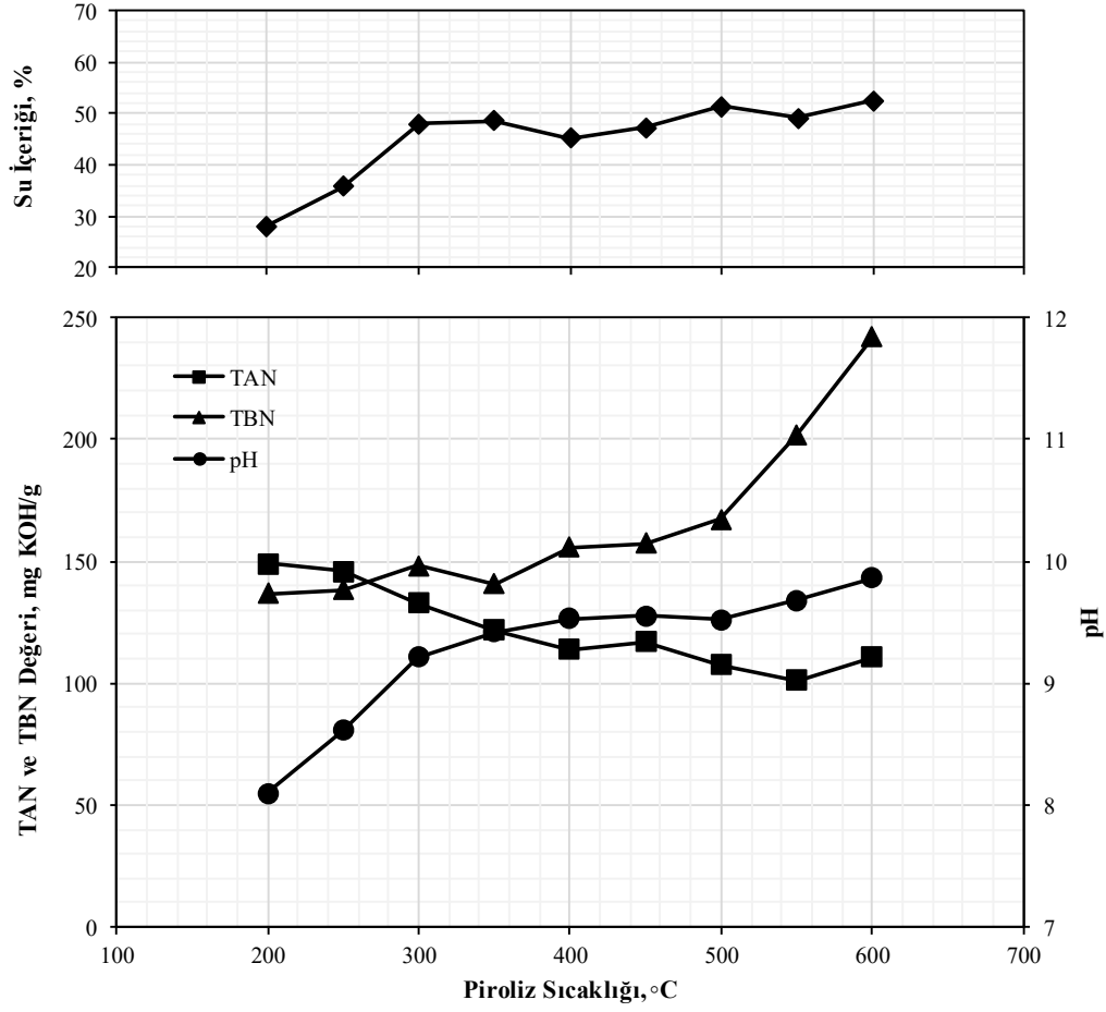
Şekil 4.5. Orjinal MDF tozunun farklı sıcaklıklarda pirolizi ile elde edilen sıvı piroliz ürünlerinin, su içeriği, pH, TAN ve TBN değerleri
