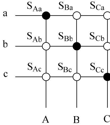
Şekil 3.9. Matris çeviricinin verilen anahtarlama durumuna göre bağlantı şekli. ( I. grup 1. nolu)
