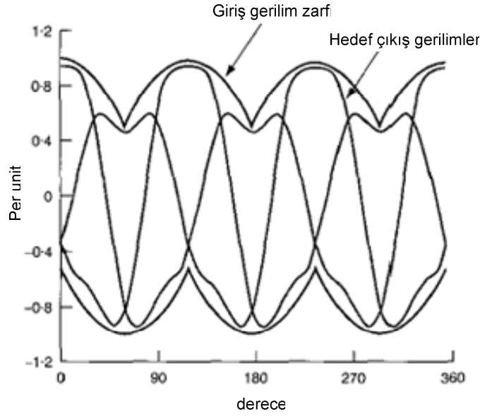
Şekil 3. 6. Matris çeviricinin üç faz giriş geriliminden elde edilen çıkış gerilimi ( q \leq 0.866 )
