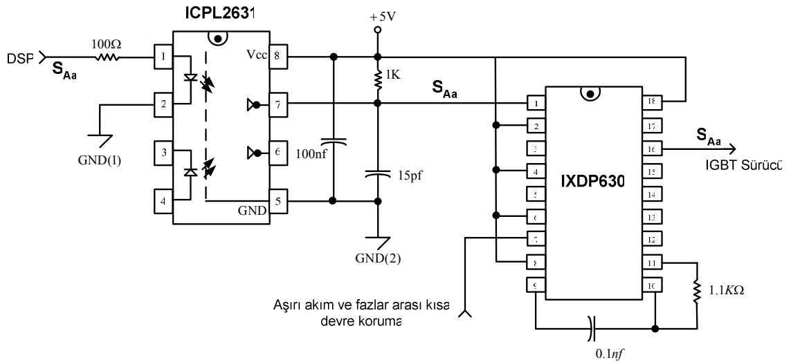
Şekil 4.5. Yalıtım ve ölü zaman ekleme devresi
