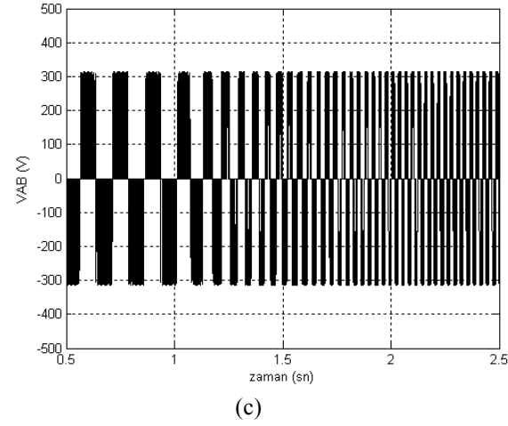
Şekil 6.15. Açık çevrim V/f kontrollü asenkron motorun benzetim sonuçları ( T_y=0 )
