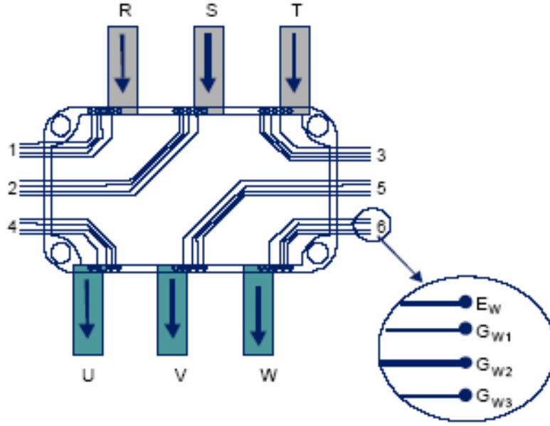
Şekil 4.4. Matris çevirici modülünün tasarım şeması
