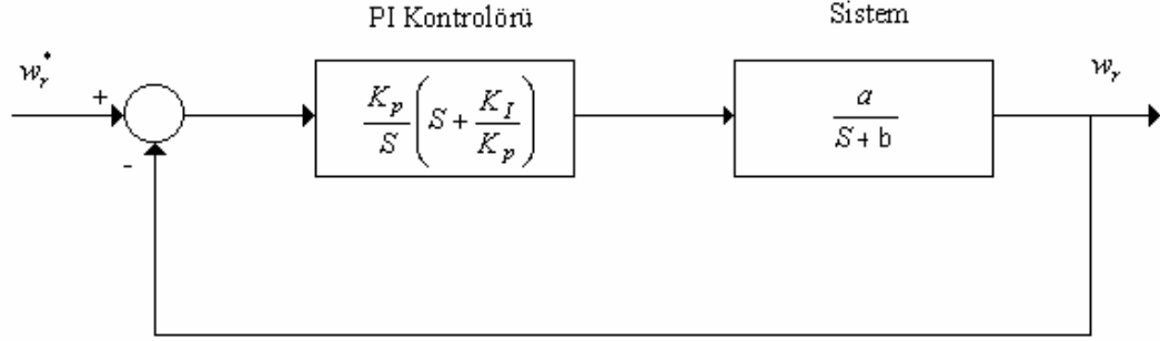
Şekil EK.8.1. Kontrol döngüsü
