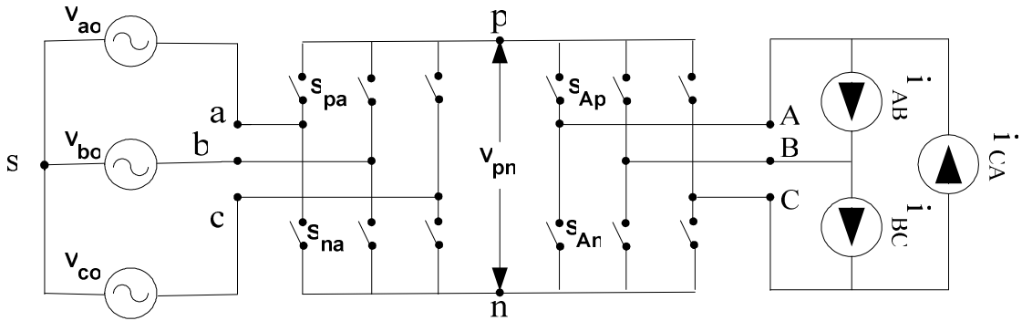
Şekil 3. 7. Matris çevirici için gerilim beslemeli evirici ve doğrultucunun gösterilimi
