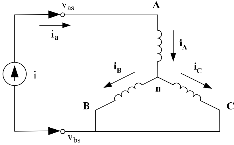
Şekil 3.12. Matris çeviricinin yüklü durumda giriş ve çıkışı arasındaki bağlantı şekli. ( IIa. grup +1 nolu)
