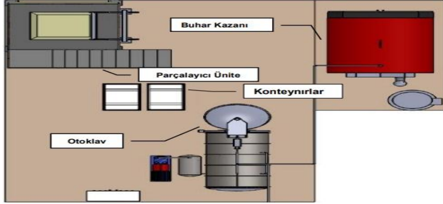
Şekil 3.12. Muş tıbbi atık tesisi ünitelerinin yerleşim planı
