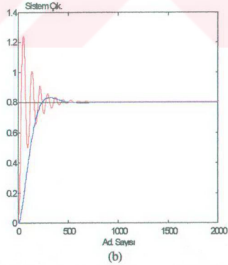
Şekil 4.6 Yapay sinir ağının 4:28'deki denklemleri genelleme yeteneği (a) Çıkış katmanındaki hareketlendirme fonksiyonu \tanh() , (b) Çıkış katmanında hareketlendirme fonksiyonu f(x)=x iken basamak giriş işaretine sistemin verdiği cevap. — referans giriş, — kontrol edilmemiş sistem çıkışı, — kontrol edilmiş sistem çıkışı
