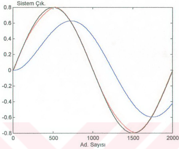
Şekil 4.9 Denklem 4.33'deki sistemin sinüzoidal referans giriş işaretine verdiği cevap. — referans giriş, — kontrol edilmemiş sistem çıkışı, — kontrol edilmiş sistem çıkışı
