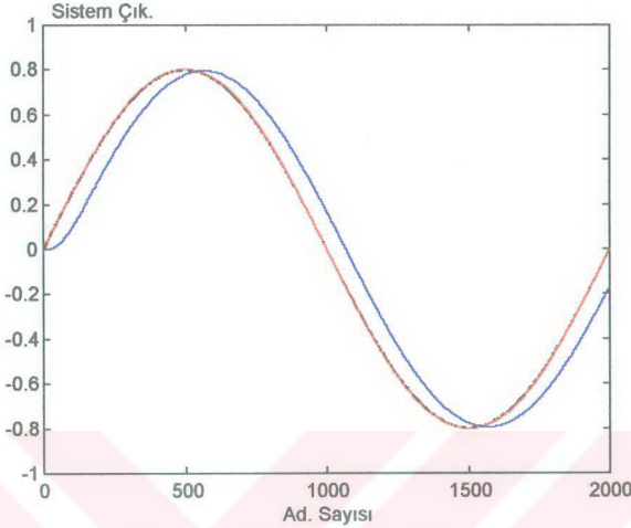
Şekil 4.34 Denklem 4.42'deki sistemin sinüzoidal referans giriş işaretine verdiği cevap. — referans giriş, — kontrol edilmemiş sistem çıkışı, — kontrol edilmiş sistem çıkışı
