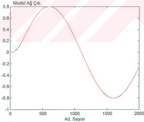
Şekil 4.22 Toplu öğrenme ile model ağın sistemi tanıması — Sistem çıkışı, — model ağ çıkışı
