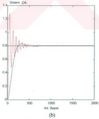
Şekil 4.24 Yapay sinir ağının 4.28'teki denklemleri genelleme yeteneği (a)Çıkış katmanındaki hareketlendirme fonksiyonu \tanh() , (b)Çıkış katmanında hareketlendirme fonksiyonu f(x)=x iken basamak giriş işaretine sistemin verdiği cevap. — referans giriş, — kontrol edilmemiş sistem çıkışı, — kontrol edilmiş sistem çıkışı
