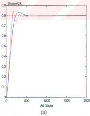
Şekil 4.6 Yapay sinir ağının 4:28'deki denklemleri genelleme yeteneği (a) Çıkış katmanındaki hareketlendirme fonksiyonu \tanh() , (b) Çıkış katmanında hareketlendirme fonksiyonu f(x)=x iken basamak giriş işaretine sistemin verdiği cevap. — referans giriş, — kontrol edilmemiş sistem çıkışı, — kontrol edilmiş sistem çıkışı
