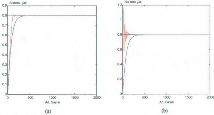
Şekil 4.16 Yapay sinir ağının 4.35'deki denklemleri genelleme yeteneği (a) Çıkış katmanındaki hareketlendirme fonksiyonu \tanh() , (b) Çıkış katmanında hareketlendirme fonksiyonu f(x)=x iken basamak giriş işaretine sistemin verdiği cevap. — referans giriş, — kontrol edilmemiş sistem çıkışı, — kontrol edilmiş sistem çıkışı
