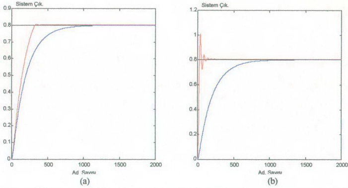
Şekil 4.28 Yapay sinir ağının 4.40'daki denklemleri genelleme yeteneği (a) Çıkış katmanındaki hareketlendirme fonksiyonu \tanh() , (b) Çıkış katmanında hareketlendirme fonksiyonu f(x)=x iken basamak giriş işaretine sistemin verdiği cevap. — referans giriş, — kontrol edilmemiş sistem çıkışı, — kontrol edilmiş sistem çıkışı
