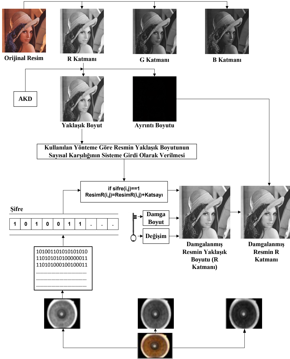
Şekil 7.6. AKD ve geliştirilen yöntem ile sisteminin blok diyagramı
