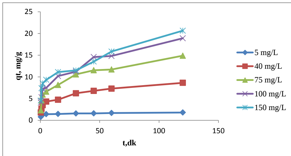
Şekil 6.1. Farklı başlangıç DR•243 konsantrasyonlarında adsorpsiyon değerlerinin zamana karşı değişim grafiği ( pH=5; T= 45 °C; X_0 =3.33 g/L; KH=150 rpm)
