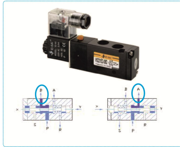
Şekil 4.21. E-MC marka pnömatis akış kontrol valf görünümü
