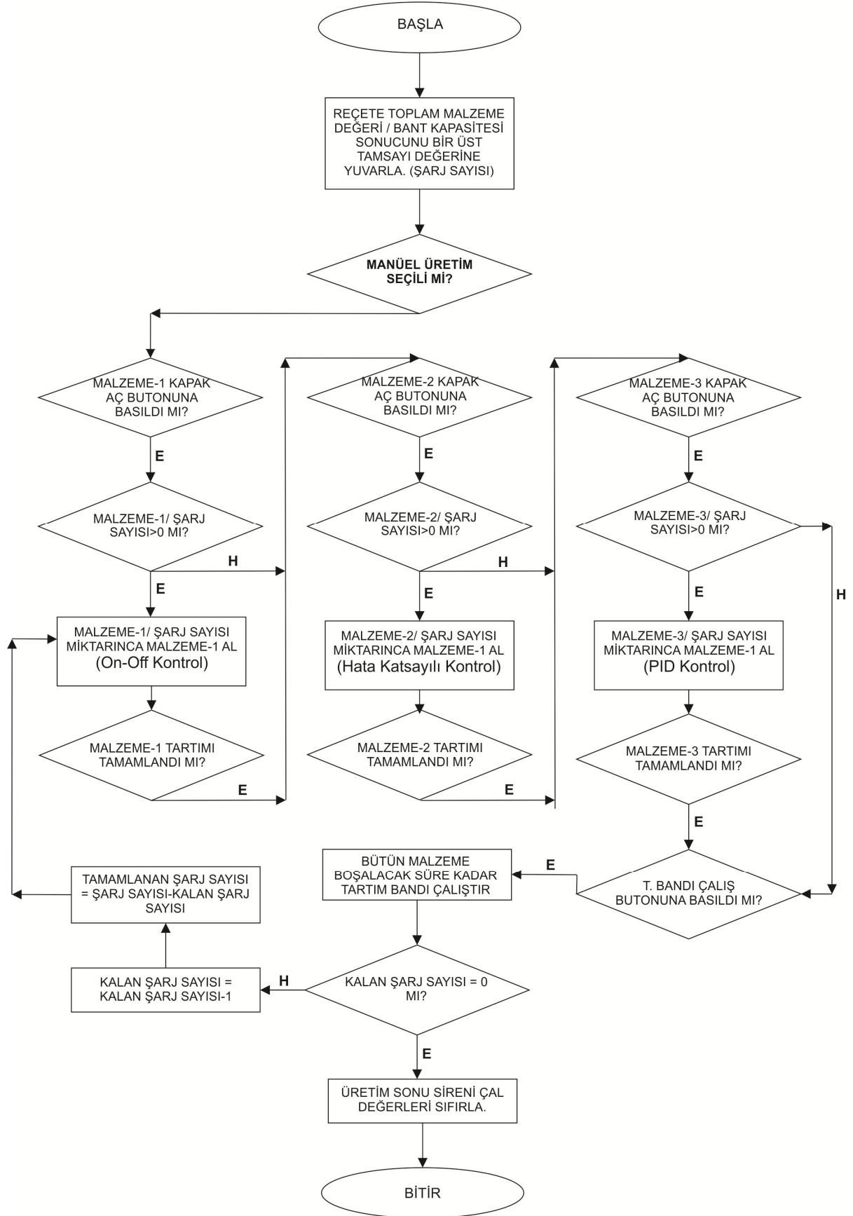
Şekil 4.3. Prototip sistem manüel üretim akış diyagramı
