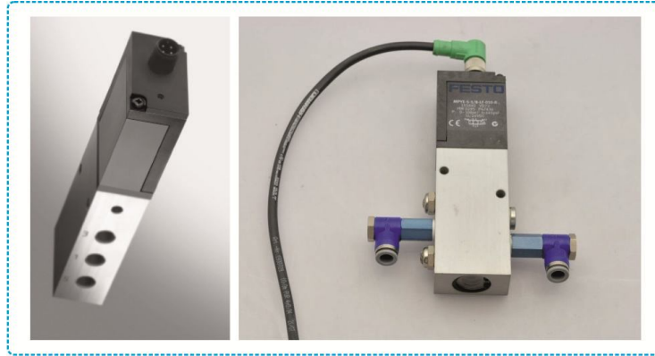
Şekil 4.17. Festo marka pnömatik oransal akış kontrol valf görünümü
