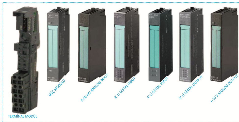
Şekil 4.12. Terminal modül ve PLC elektronik kart görünümleri
