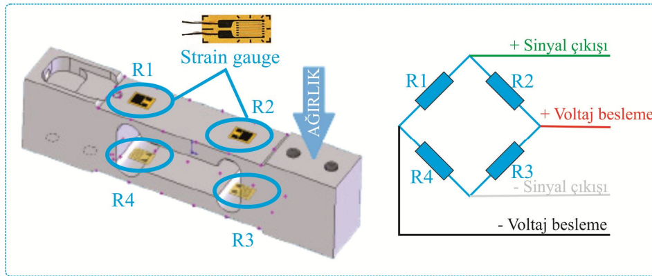
Şekil 4.14. Loadcell, Strain guage ve loadcell elektrik kablolarının renklere göre bağlantı gösterimi
