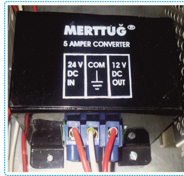
Şekil 4.25. Merttuğ marka 24 VdC – 12 VDC güç kaynağı görünümü
