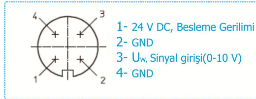
Şekil 4.20. Festo marka pnömatik oransal akış kontrol valfinin elektrik soketi bağlantı uçları ve görevleri
