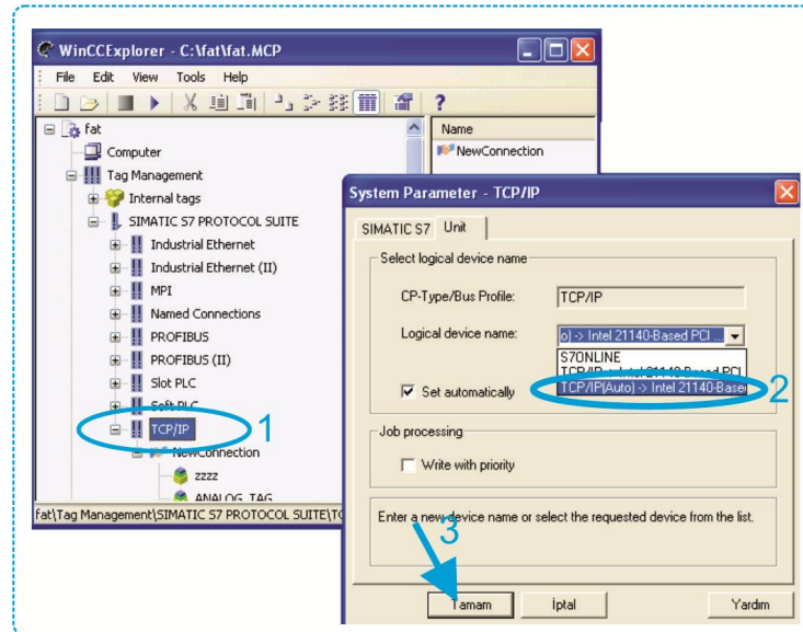
Şekil 7.7. WINCC programında PLC haberleşirme bilgisayar donanımının seçilme adımları
