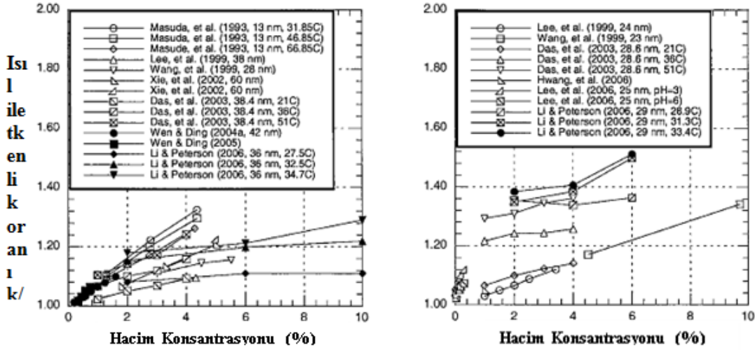
Şekil 1.2. ısı iletkenlik üzerinde hacimsel oran ve sıcaklığın etkisi
