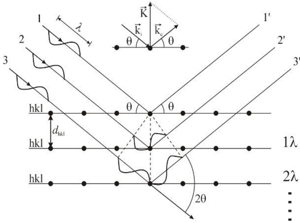
Şekil 3.12. Atomik ölçekli kristal yapı
