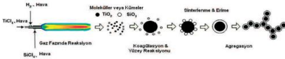
Şekil 2.8. Alev sentezi yöntemi ile nanomalzeme üretimi
