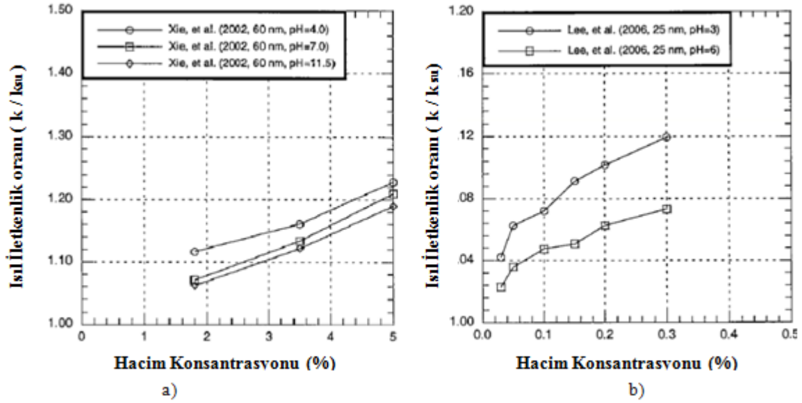
Şekil 2.20. a) \text{Al}_2\text{O}_3 -Su, b) \text{CuO} -Su nanoakışkanlarının değişik pH değerlerindeki, farklı hacim konsantrasyonlarına karşılık gelen ısıl iletkenlik oranı
