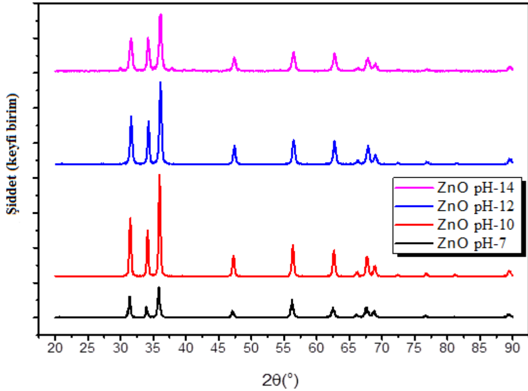
Şekil 4.10. XRD (X-ışını Kırınım) ZnO analizi sonuçları
