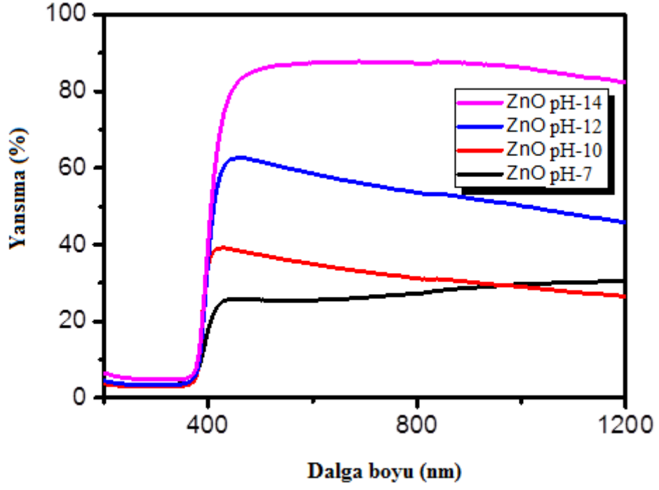
Şekil 4.15. Toz haline getirilmiş ZnO UV-görünür yansıtma spektrumları
