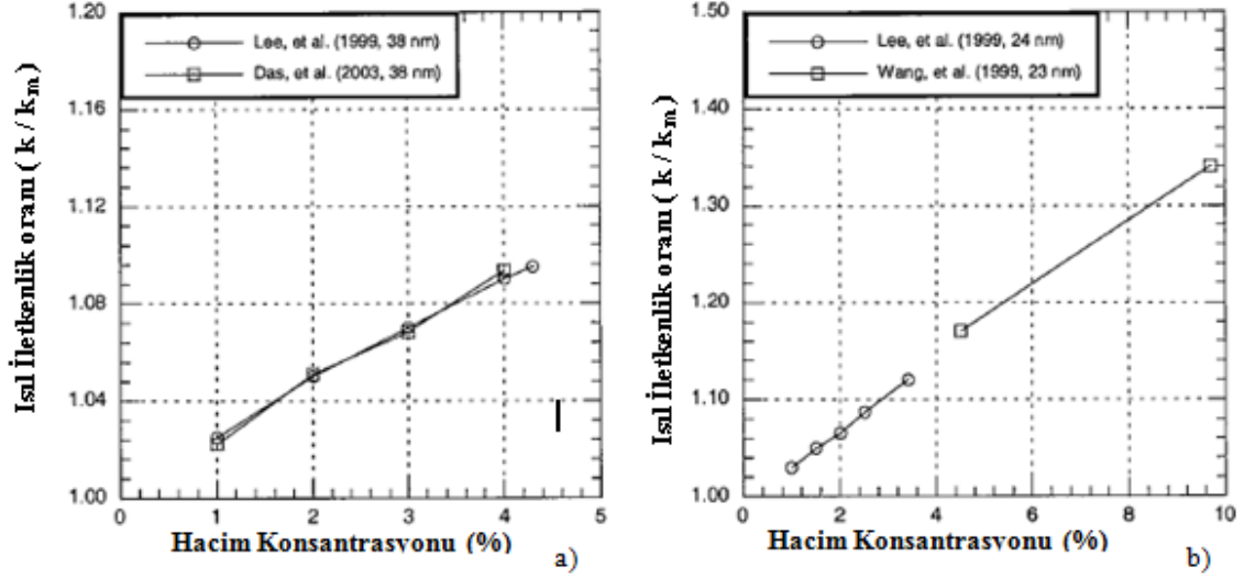
Şekil 2.19. a) \text{Al}_2\text{O}_3 -Su, b) \text{CuO} -Su değişik boyutlardaki nanoakışkanların, farklı hacim konsantrasyonlarında ısıl iletkenlik oranı
