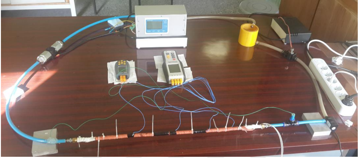
Şekil 3.16. Deney düzeneği
