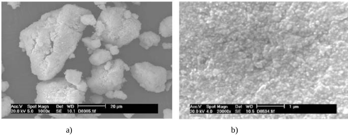
Şekil 2.15. a) Topaklanmış CuO partikülleri , b) homojene yakın dağılmış CuO partikülleri
