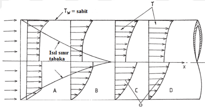
Şekil 2.28. Isıl sınır tabaka gelişimi
