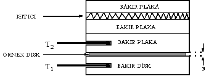
Şekil 2.17. Lee Disk yönteminin şematik gösterimi
