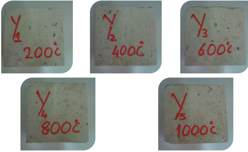
Resim 4.9. Sıcaklık Etkisi Deney Numuneleri
