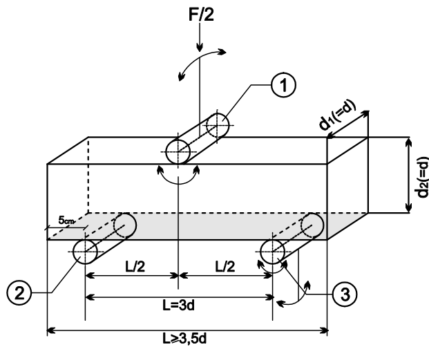
Şekil 4.2. Deney Numunesi Yükleme Düzenegi
