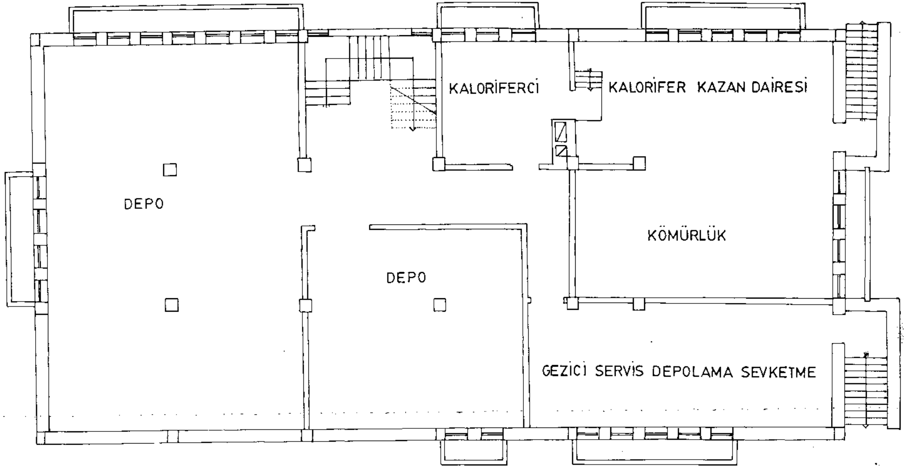
Elazığ İl Halk Kütüphanesi Yapısının Planı Bodurum Kat
