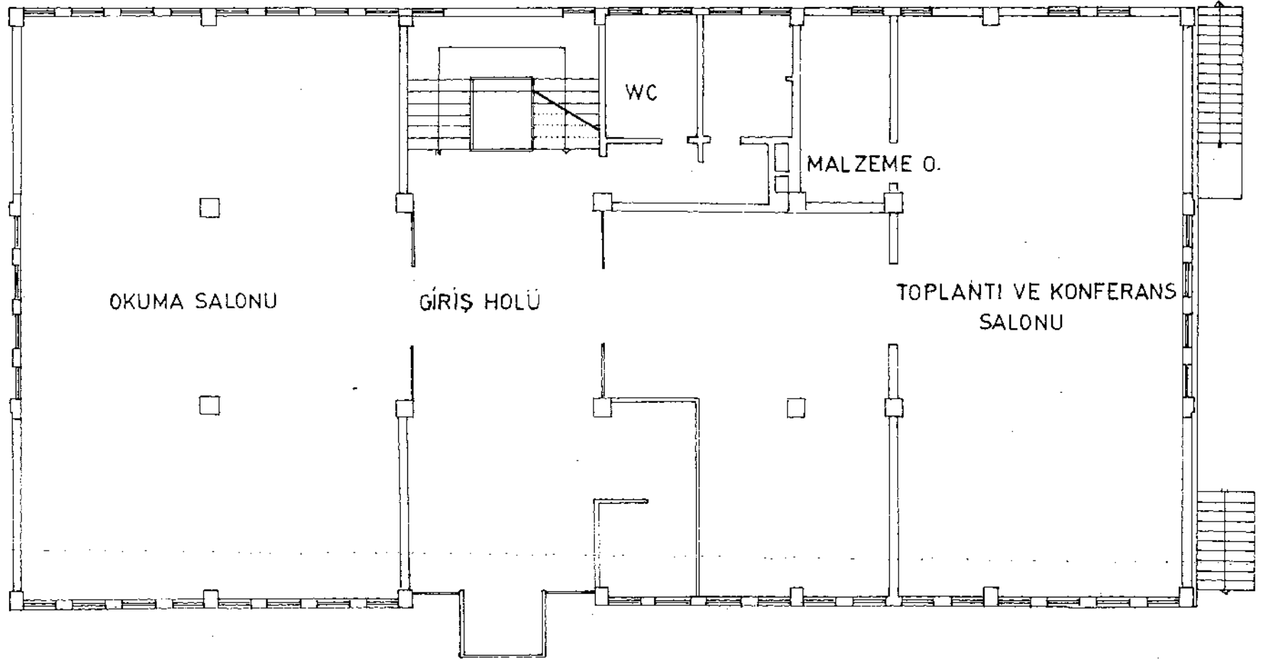
Elazığ İl Halk Kütüphanesi Yapısının Planı Zemin Kat
