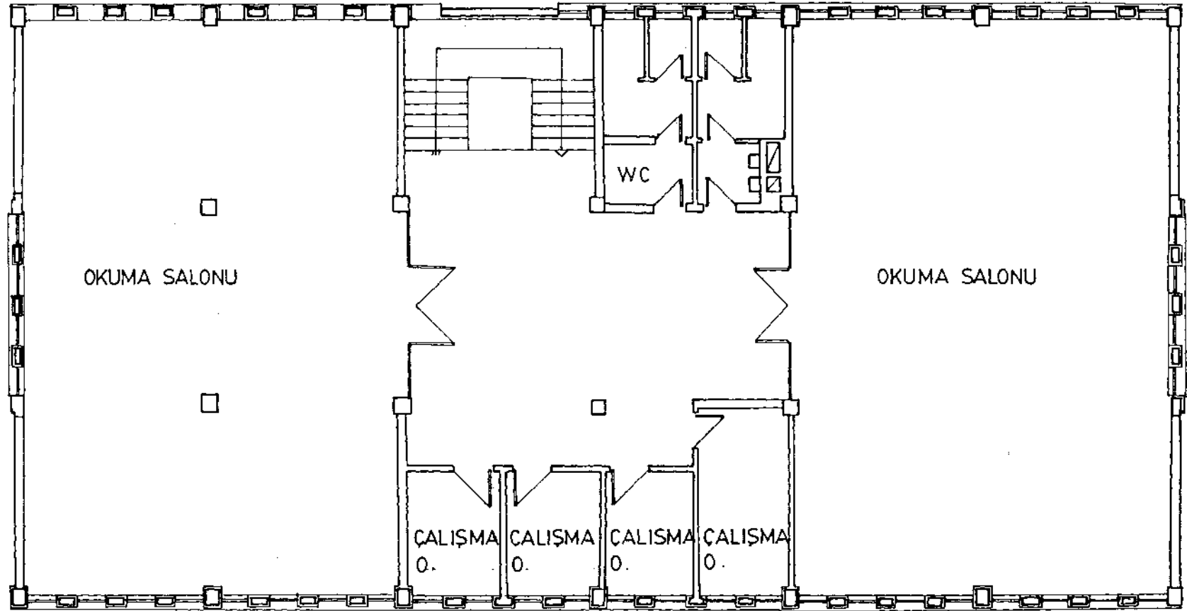
Elazığ İl Halk Kütüphanesi Yapısının Planı Birinci Kat
