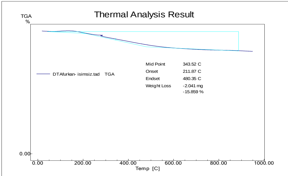
Şekil 6.8. TiO 2 numunesine ait TG eğrisi.
