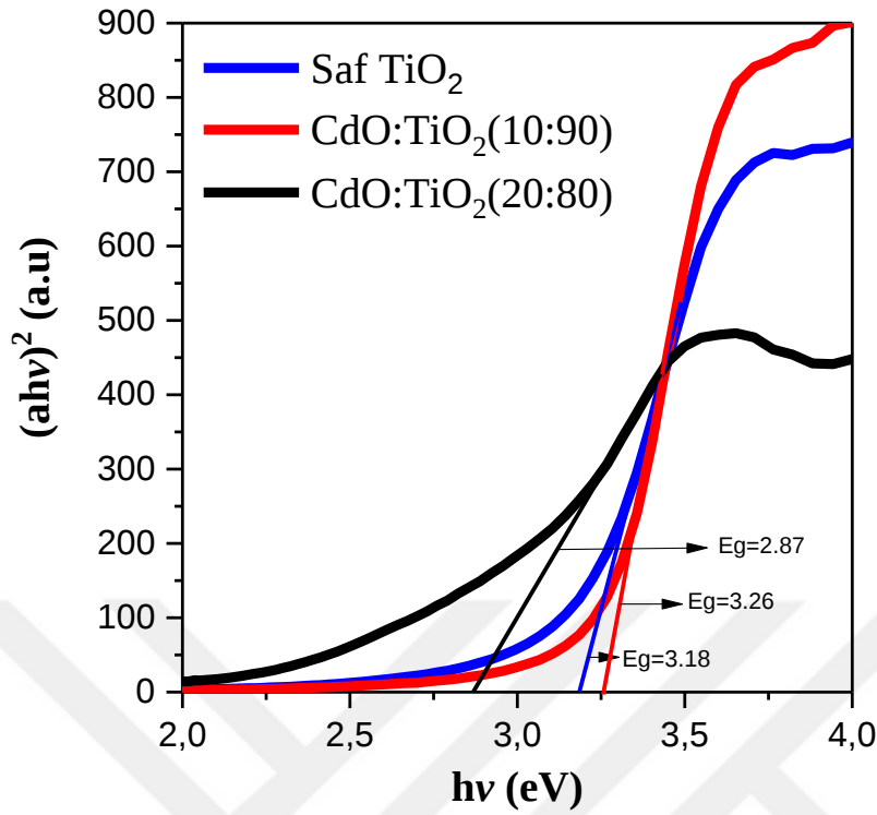
Şekil 6.4. Numunelerin (\alpha hv)^2-hv spektrumu
