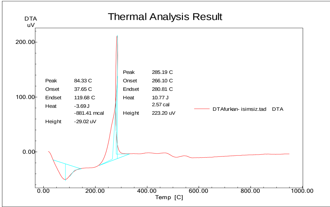
Şekil 6.7. TiO 2 numunesine ait DTA eğrisi.
