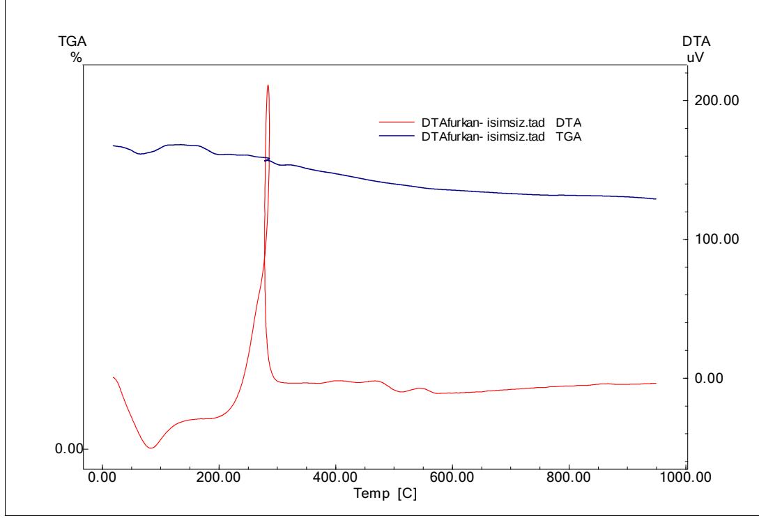
Şekil 6.6. TiO 2 numunesine ait TG/DTA eğrisi
