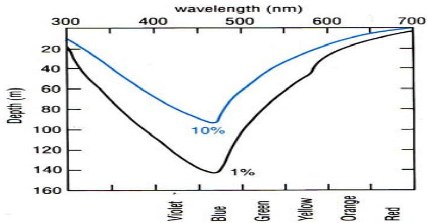
Şekil.1.1.1. Farklı derinliklerde görülen renkler ve dalga boyları
