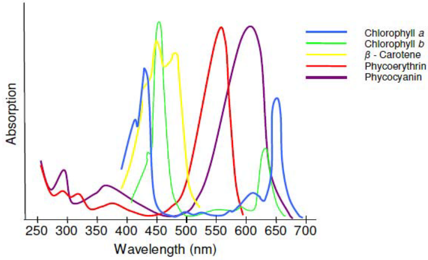
Şekil.1.4.1. Üç ana pigment sınıfının(Klorofil, Karotenoid ve Fikobilin) farklı spektrumlardaki absorpsiyon miktarları
