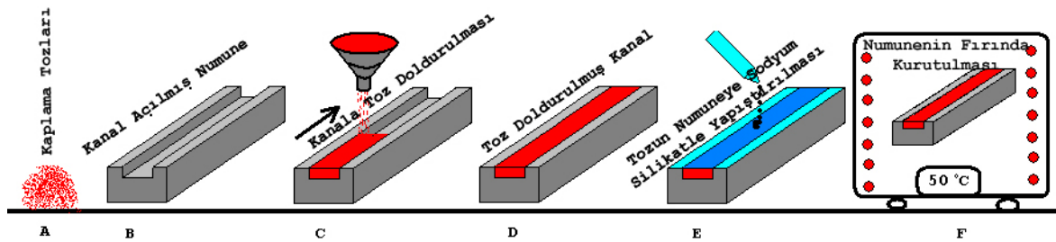
Şekil 8.4. Kaplama işlemi için numunelerin hazırlanma aşamasının şematik görünümü
