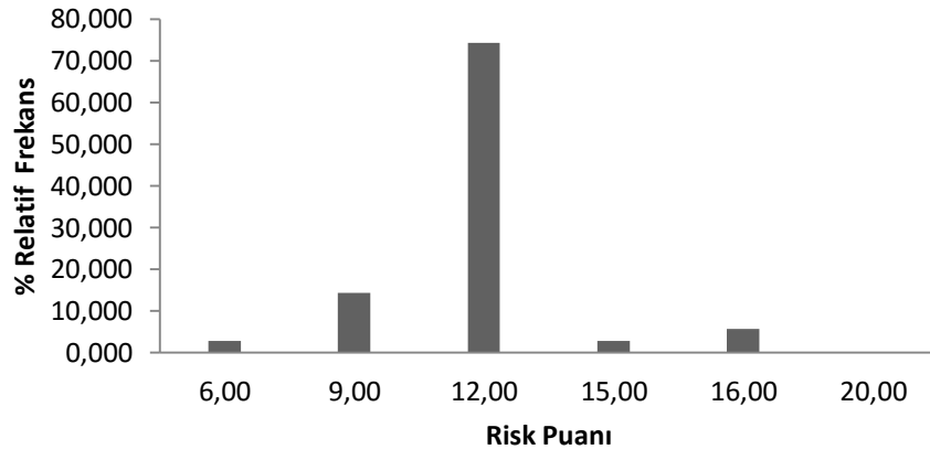
Şekil 6.10. Çimento değırmeni risk puanı - % relatif frekansı
