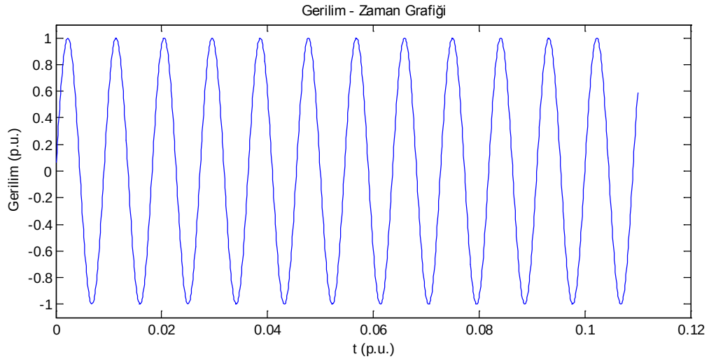
Şekil 6.55. 616 d/d için generatör çıkış geriliminin zaman ile değişimi (Benzetim sonucu)
