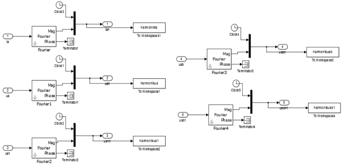
Şekil 6.8. Harmonik bilgisinin şeması
