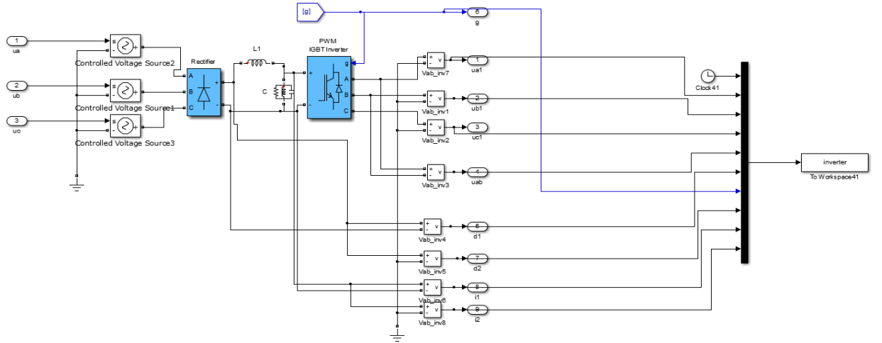
Şekil 6.9. İnverter şeması
