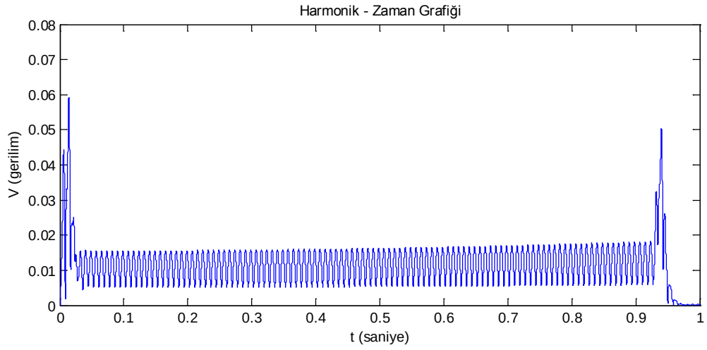
Şekil 6.32. Generatör çıkış 3. Harmoniğinin zaman ile değişimi
