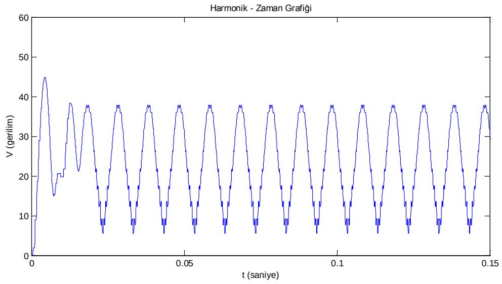
Şekil 6.37. İki seviyeli inverter çıkış 3.Harmoniğinin zaman ile değişimi
