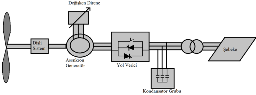
Şekil 5.1. Asenkron generatörlerin şebekeye bağlantı şeması [1]
