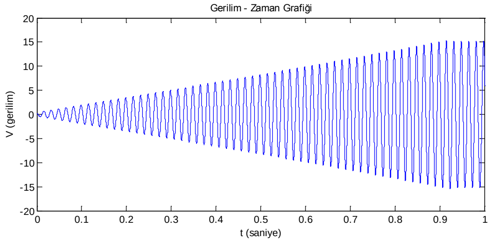
Şekil 6.30. Generatör çıkış geriliminin zaman ile değişimi
