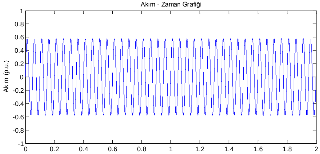
Şekil 6.60. 400 \Omega 'luk yük için akımın zaman ile değişimi (Benzetim sonucu)
