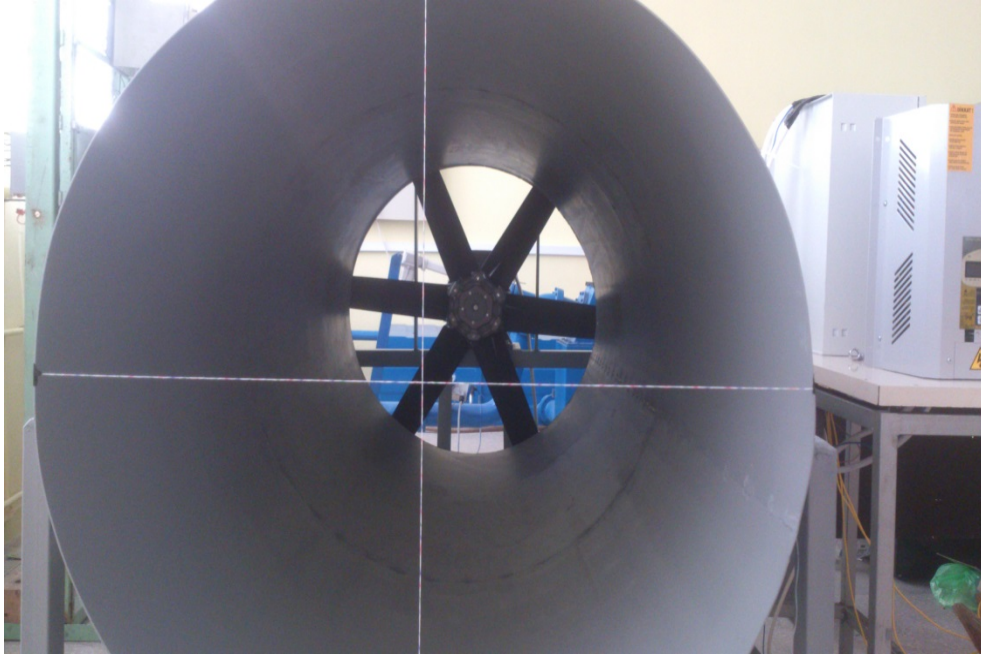
Resim 6-6. Sürekli mıknatıslı senkron generatörlü rüzgar türbininin montajının yapılacağı kısım
