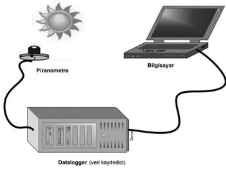
Resim 1. Güneş ışınlamı ölçüm düzeneğinin şematik görünümü
