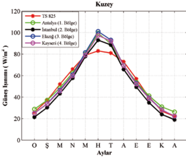
Resim 6. Kuzey yönü için hesaplanan güneş ışınlımlı değlerleri ile EK-C'de verilen değlerlerin karşılaştırılması.
