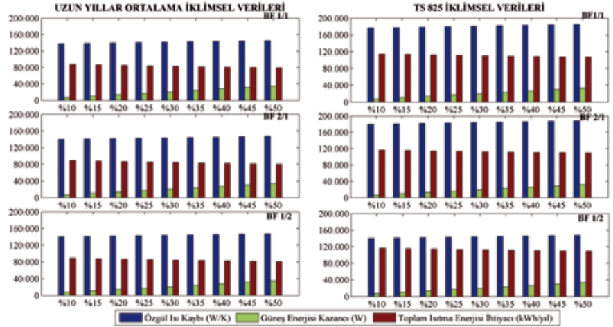
Resim 11. Kayseri İli Farklı Biçim Faktörü ve Saydamlık Oranları İçin Hesaplanan Özgül Isı Kaybı, Güneş Enerjisi Kazancı ve Yıllık Isıtma Enerjisi İhtiyaçları
