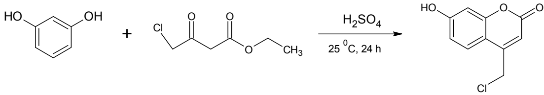
Şekil 2.1. KMHK 'in sentez reaksiyonu.
