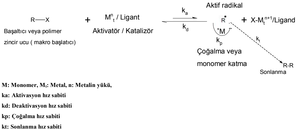
Şekil 1.1. ATRP'nin genel reaksiyon mekanizması
