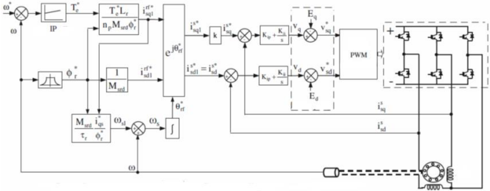
Şekil 4.7. Dolaylı rotor akı yönlendirmeli kontrolün kapsamlı blok şeması
