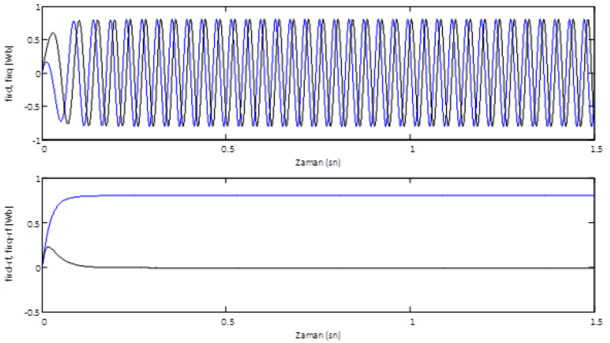
Şekil 5.9. Yüksüz durumda duran ve senkron dönen çatıda rotor akısının değişimleri
