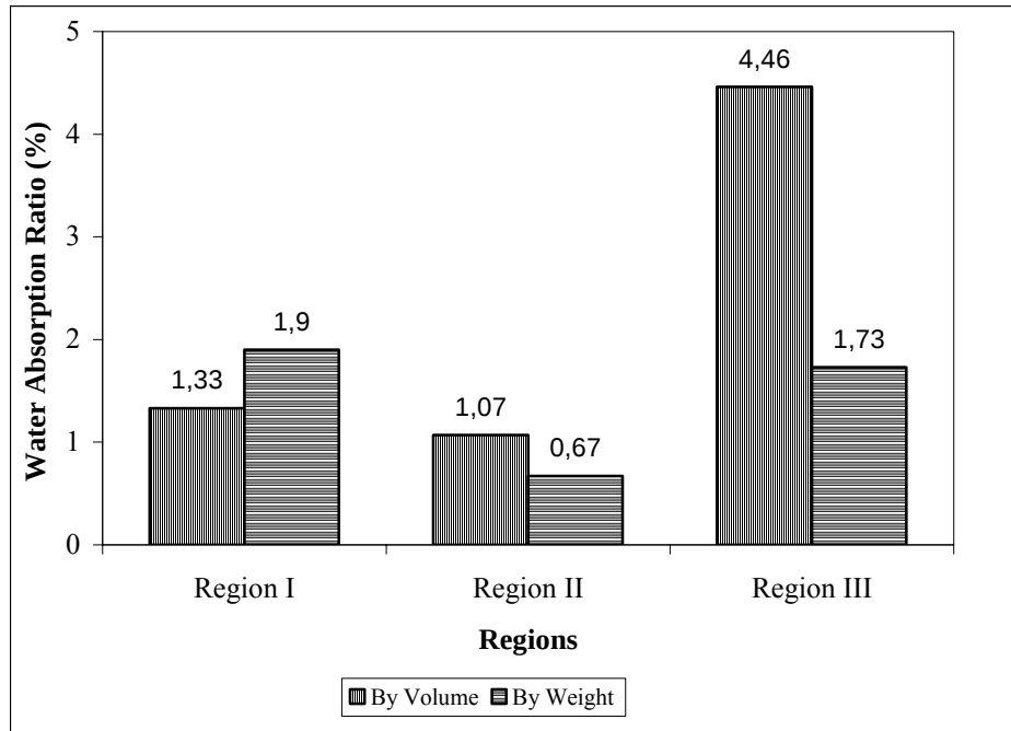
Figure 3. Water absorption ratios of the Basalt stones (Şekil 3. Bazalt taşlarının su emme oranları)
