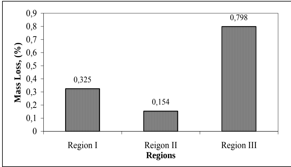
Figure 4. Mass loss variations of the specimens after freeze-thaw test (Şekil 4. Don tesiri deneyi sonrası numunelerin kütle kaybı değişimleri)
