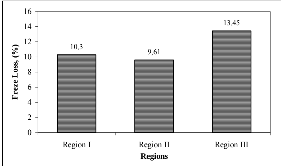
Figure 6. Freeze loss with sodium sulphate variations of the specimens (Şekil 6. Numunelerin sodyum sülfat don kaybı değişimleri)
