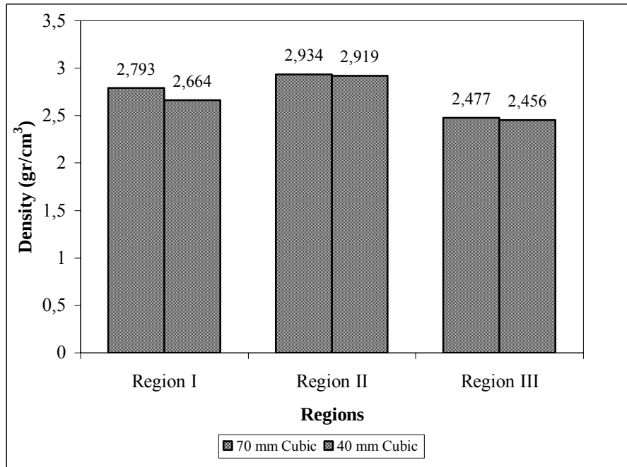
Figure 2. Density variations of the basalt stones (Şekil 2. Basalt taşlarının yoğunluk değişimleri)
