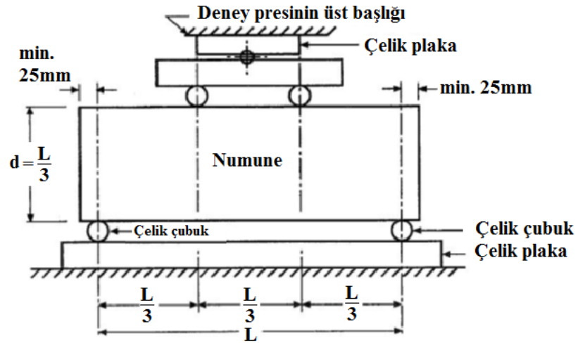
Şekil 3.6. Uzunluğu L olan irişin L/3 uzaklıktaki mesafelerde yüklenmesi deney düzeneği
