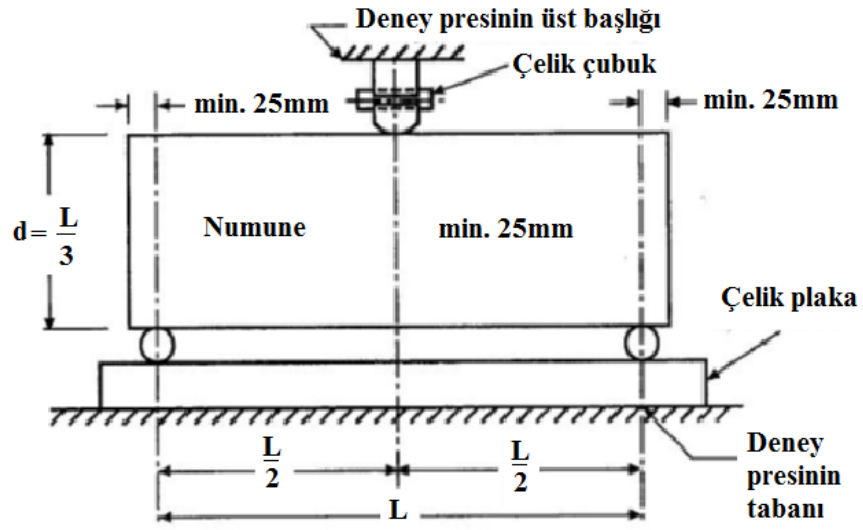
Şekil 3.5. Kirişin orta noktasından yüklenmesi durumunda deney düzeneği
