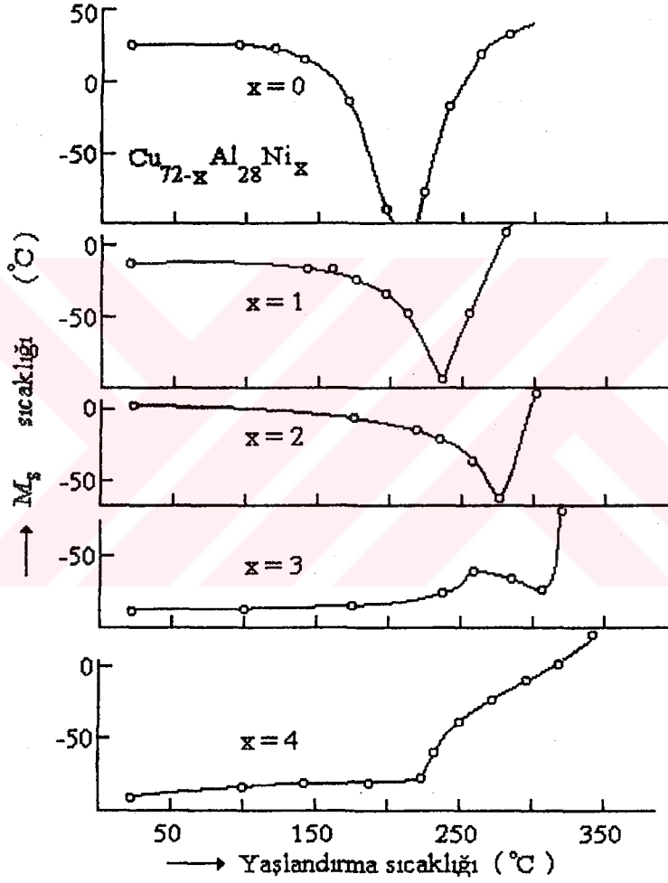
Şekil 4.4. CuAlNi alaşımlarında farklı Ni(x) konsantrasyonu için M s dönüşüm sıcaklığının yaşlandırma sıcaklığı ile değişimi (Funakubo, 1987).
