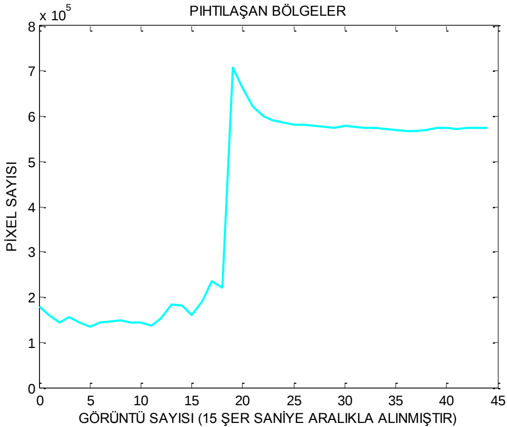
Şekil 4.2. Kan örneği alınan örnek bir kişiye ait pıhtılaşma görüntüsü
