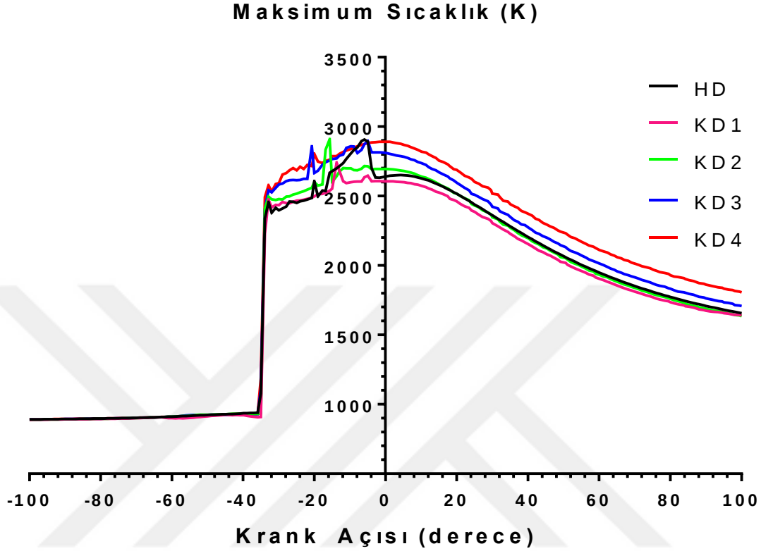
Şekil 3.12. Silindir içi maksimum sıcaklığın farklı püskürtme zamanlamalarına bağlı olarak değişimi
