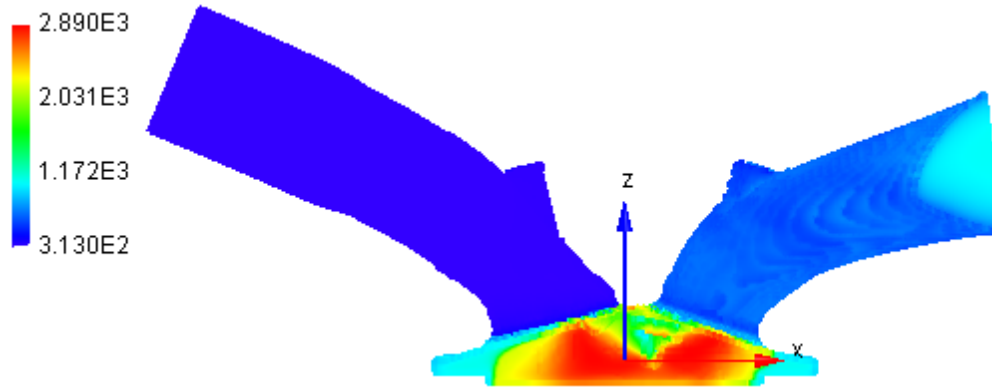
Şekil 3.22. Farklı dolgu şartlarında OKMA için sıcaklık dağılımları
