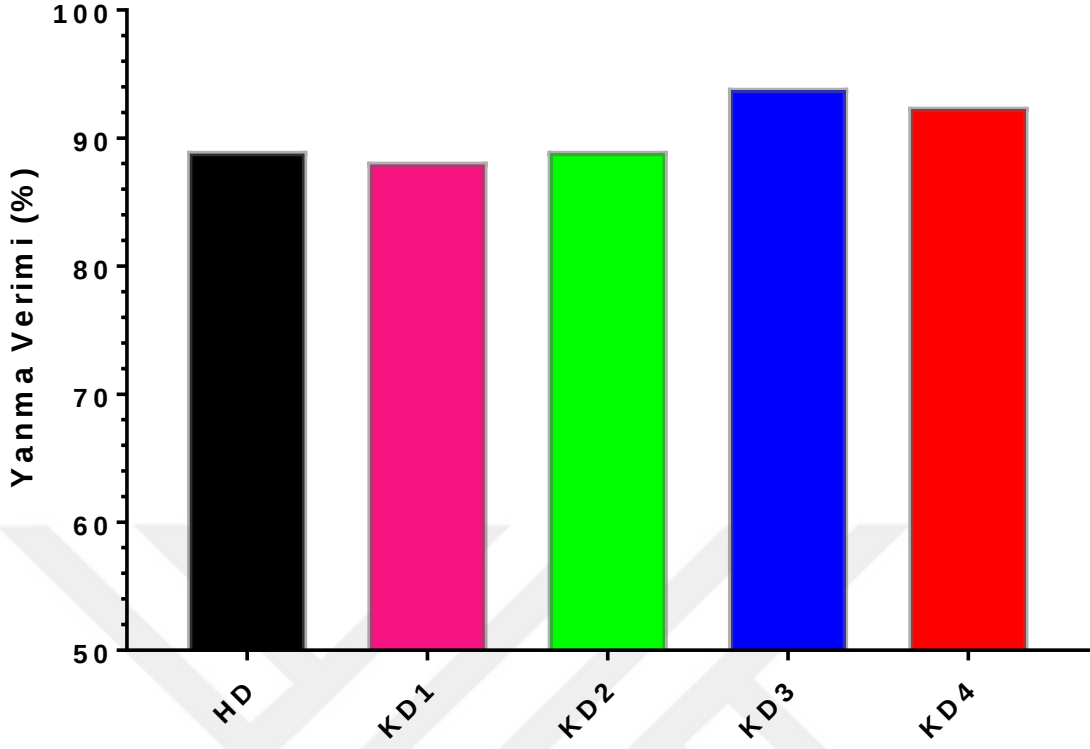
Şekil 3.18. Yanma veriminin farklı püskürtme zamanlamalarına bağlı olarak değişimi
