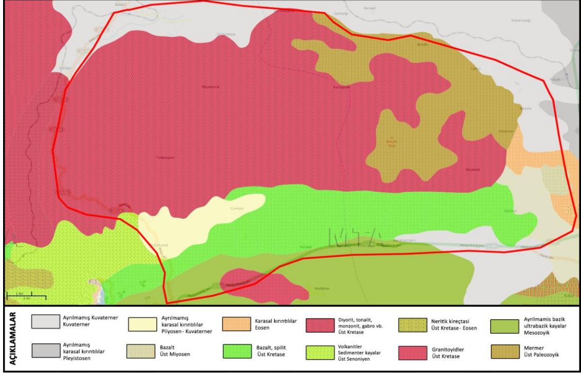
Harita 5: Araştırma alanının Jeolojik Haritası (MTA).
