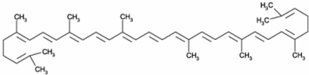
Şekil 4. Likopenin kimyasal yapısı (60)
