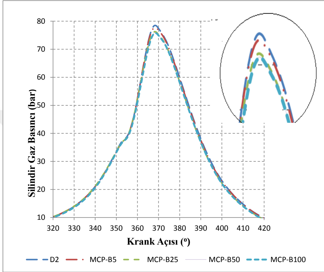
Şekil 4.21. 1500 d/d 10.56 kw yükte D2, MCP-B5, MCP-B25 ve MCP-B50 yakıtları için silindir gaz basınç değişimleri
