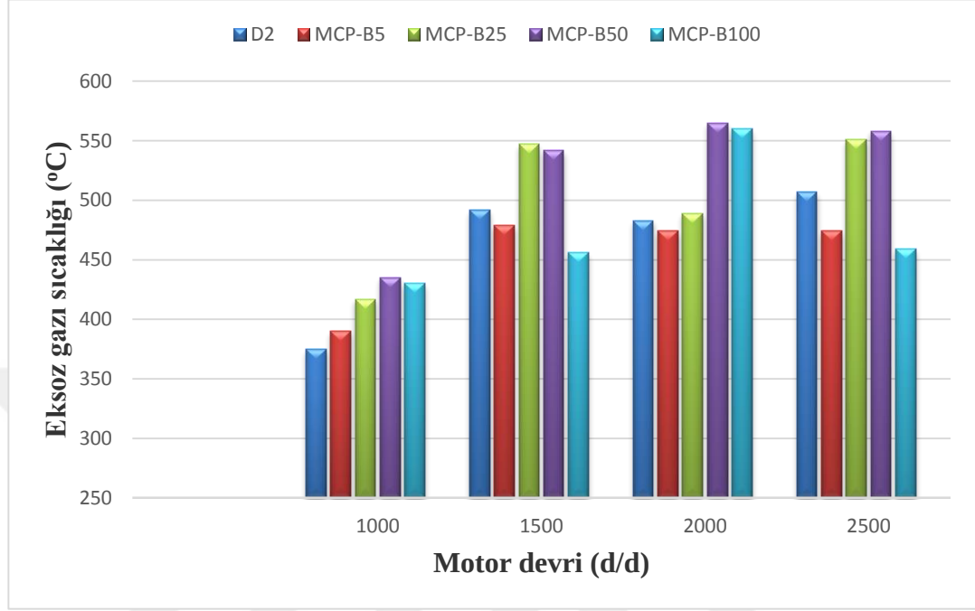
Şekil 4.8. Dizel yakıtı ile biyodizel karışımlarının motorun sabit gaz keleşi konumunda ve deęişik devir sayılarına göre egzoz gaz sıcaklığı deęişimi
