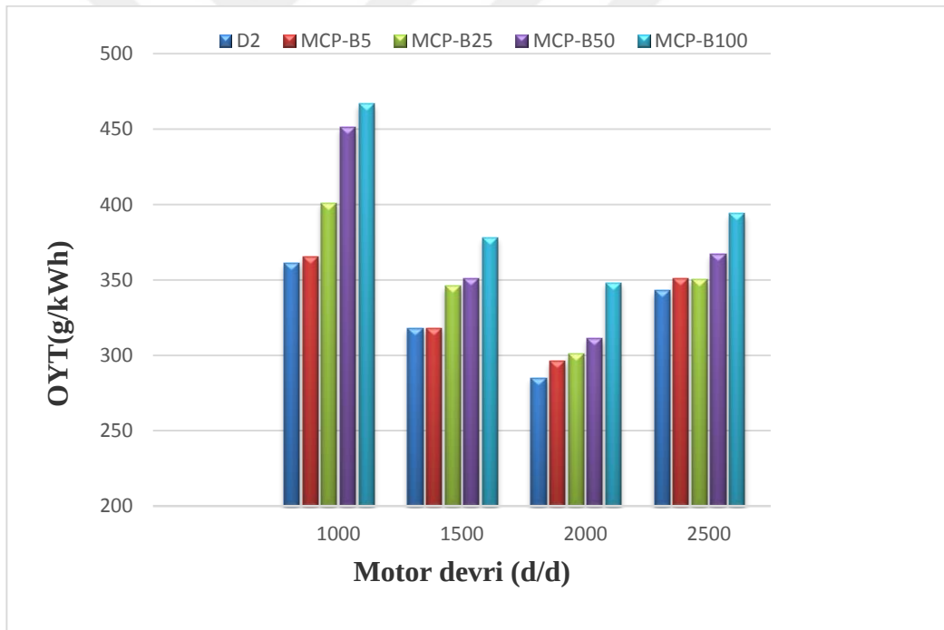
Şekil 4.3. Dizel yakıtı ile biyodizel karışımlarının motorun sabit gaz keleşeği konumunda ve deęişik devir sayılarına baęlı özgül yakıt tüketimi deęişimi
