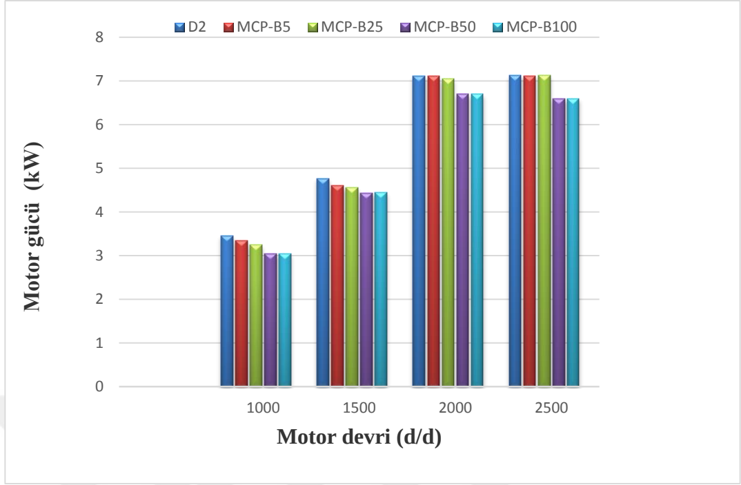
Şekil 4.2. Dizel yakıtı ile biyodizel karışımlarının motorun sabit gaz keleşi konumunda ve deęişik devir sayılarına baęlı efektif güç deęişimi
