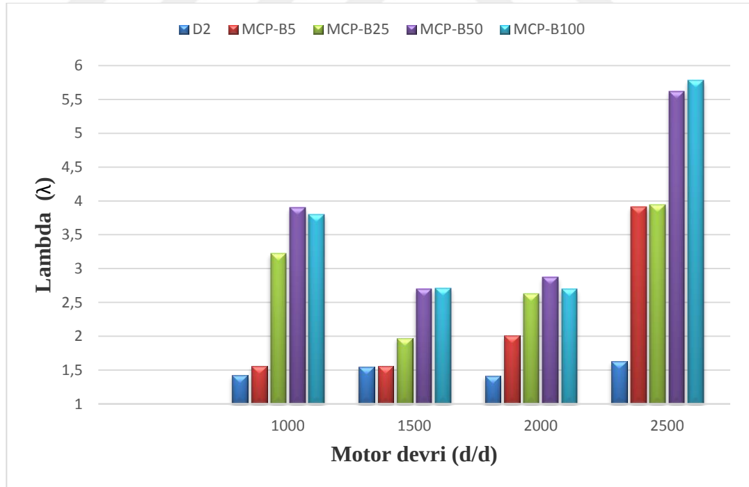
Şekil 4.10. Dizel yakıtı ile biyodizel karışımlarının motorun sabit gaz keleşi konumunda ve deęişik devir sayılarına göre ( \lambda ) deęişimi
