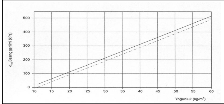
Şekil 3.3. Ekpande polistrenin %10 deformasyondaki basınç geriliminin yoğunlukla değişimi (EN 13163) [28].
