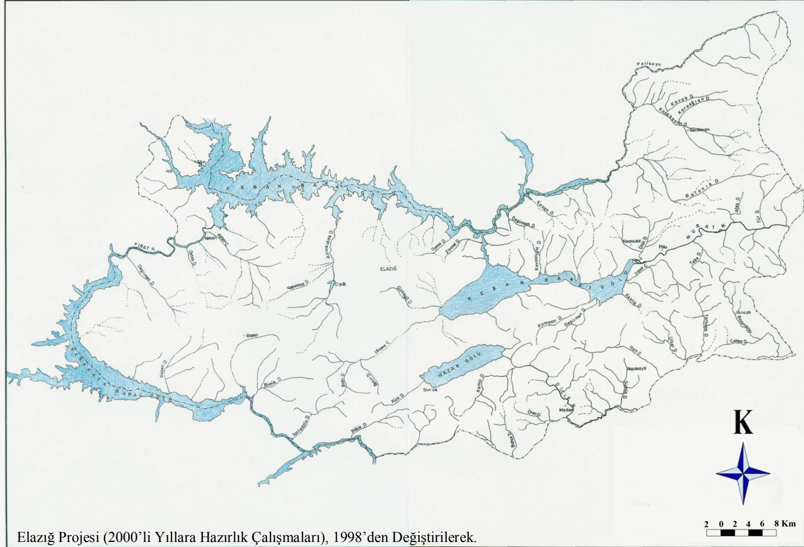
Harita 6: Elazığ İlinin Hidrografya Haritası
