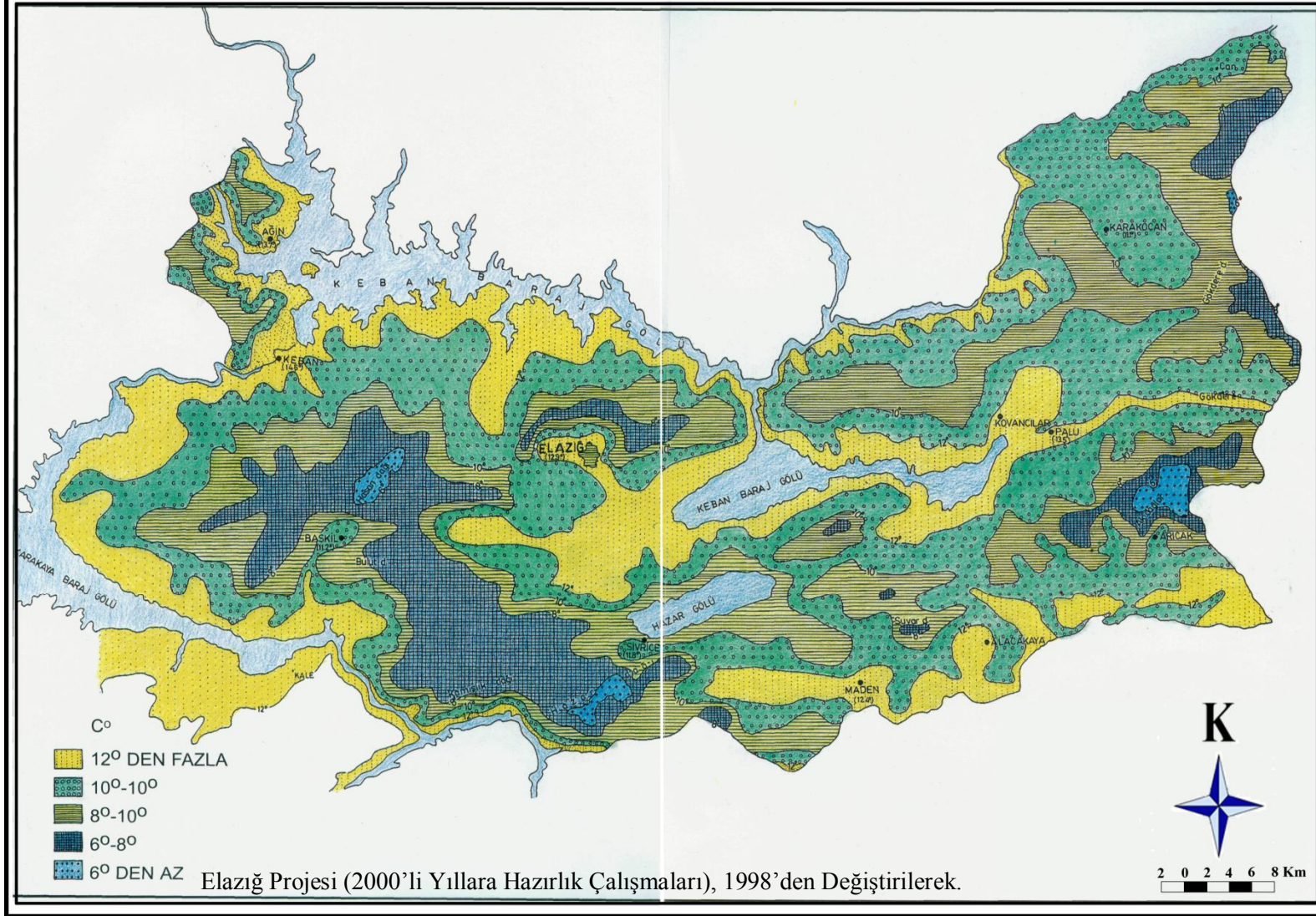
Harita 4: Elazığ İlinin Yıllık Ortalama Sıcaklık Haritası
