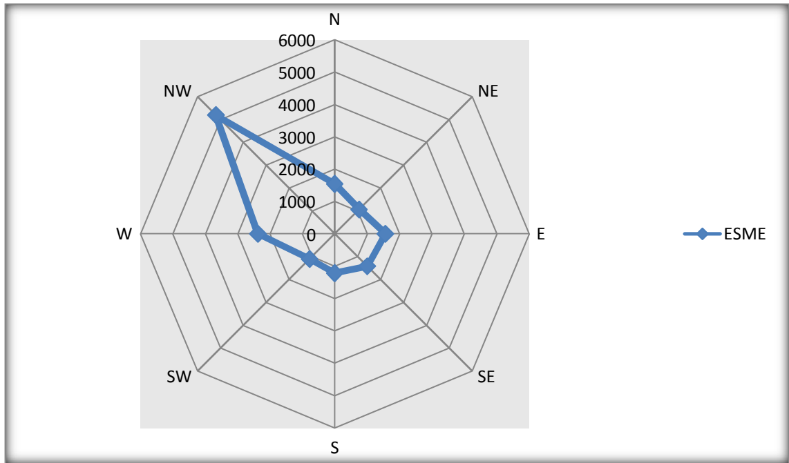
Grafik 2: Elazığ Şehrine Ait Rüzgâr Güllü
