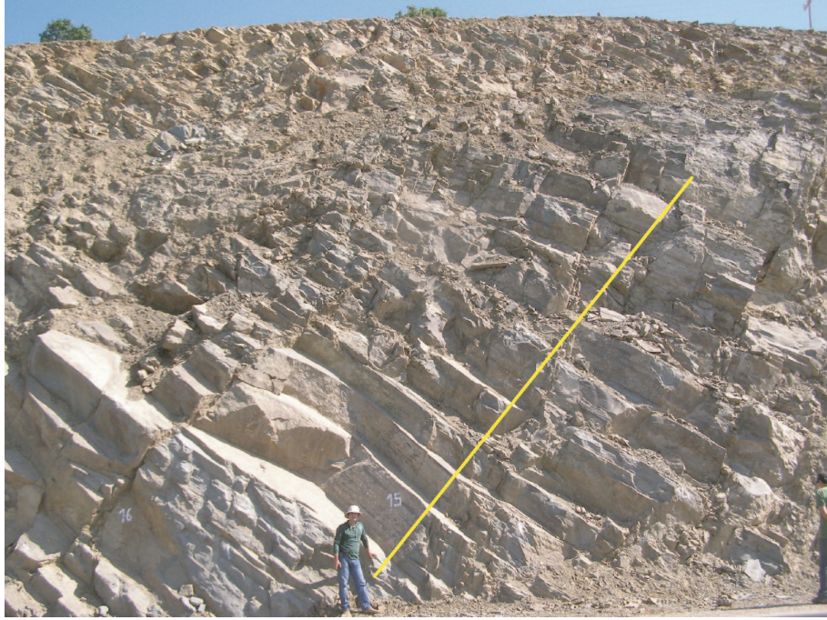
Şekil 4.1. Silttaşlarında hat etüdü çalışmaları.
