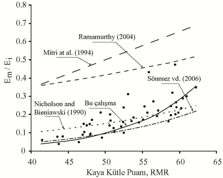
Şekil 5.12. Silttaşı kaya kütlelerinde E_m/E_i ile RMR arasındaki ilişkiler ve diğer araştırmalar ile karşılaştırılması
