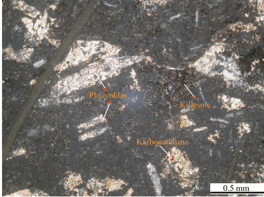
Şekil 3.7. Maden Karmaşığı'na ait bazaltlardaki mikrolitik porfirik dokunun çift nikoldeki mikroskop görünümü.
