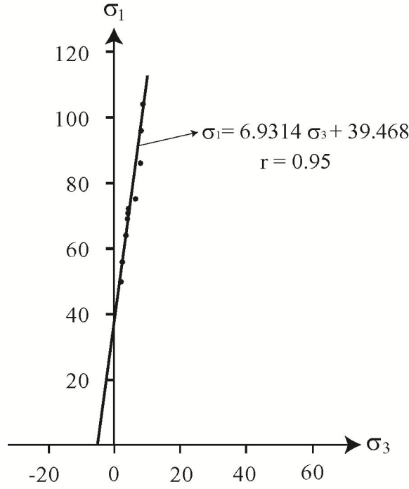
Şekil 4.26. \sigma_1 ve \sigma_3 veri çiftleri kullanılarak çizilen regresyon grafiği
